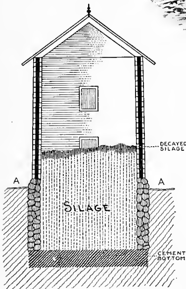
FIG. 140.— Section of Silo.
