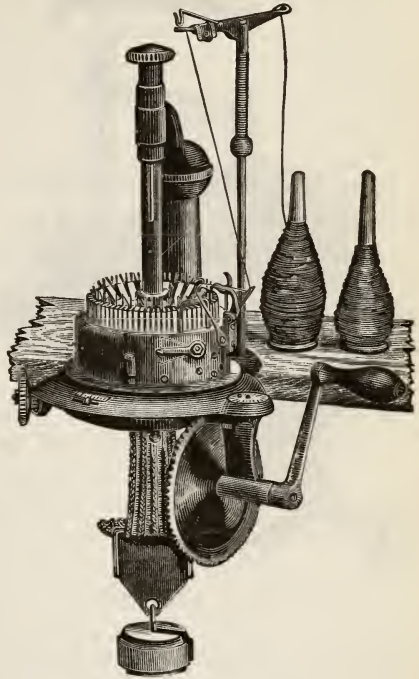
LAMB KNITTING-MACHINE.
