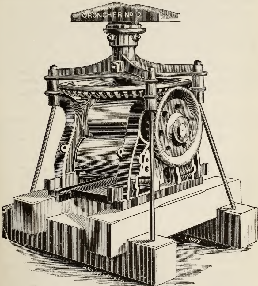
SUGAR-MILL.
