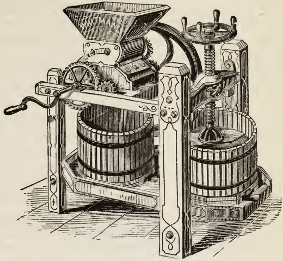
CIDER-MILL.
