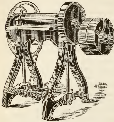
POWER-ROLLER.
