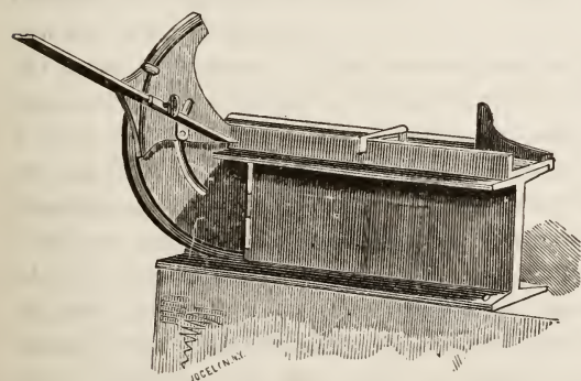
MITRING-MACHINE.
