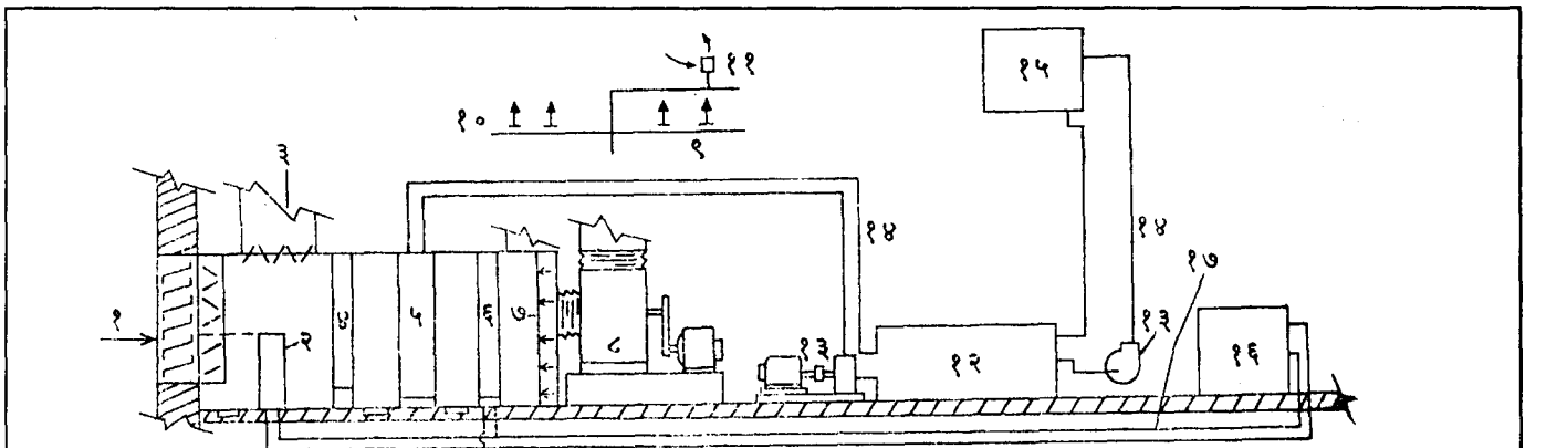
मध्यवर्ती वातानुकूलन यंत्रणा : हवा विभाग - (१) बाह्य हवा प्रवेश मार्ग, (२) पूर्वतापक, (३) परतुपी हवा, (४) गाळणी, (५) निराद्रीकारक, (६) पुनर्तापक, (७) आर्द्रीकारक, (८) पंखो, (९) हवा वाहिन्यो, (१०) आनी (११) हवा क्षेपक/विसारक; प्रशीतन विभाग - (१२) प्रशीतन यंत्रणा; जलविभाग - (१३) पंप, (१४) जलवाहिन्यो, (१५) शीतक मनोरो; तापन विभाग - (१६) बाश्पीत्र आनी सहाय्यक साधनां, (१७) तापक नळ.
