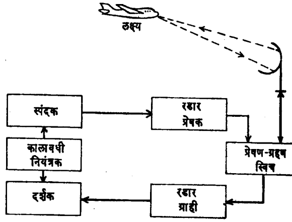
स्पंद रडार प्रणाली
