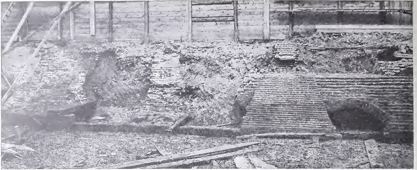
C — FUNDEERING VOORMALIGE N. Z. KAPEL TE AMSTERDAM.
