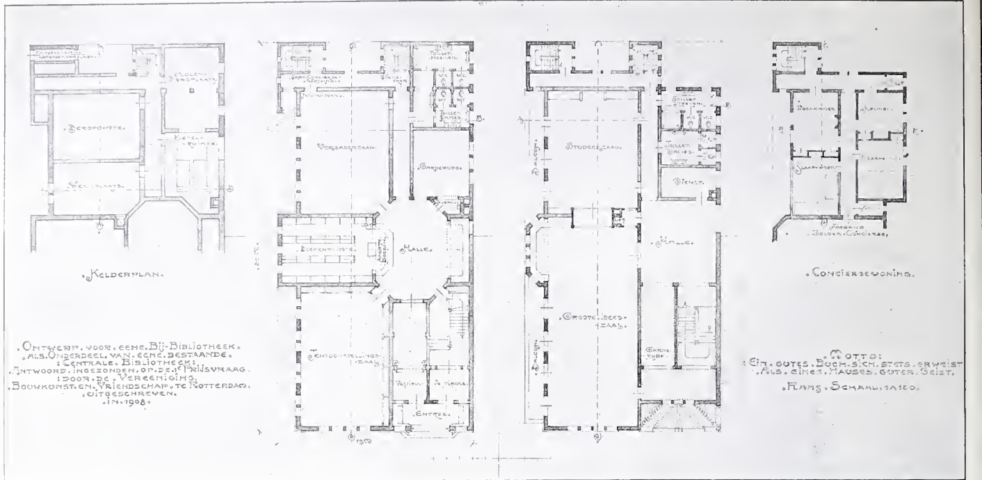
PLATTEGRONDEN BIJ-BIBLIOTHEEK, MOTTO: „EIN GUTES BUCH" U.S.W.—TWEEDDE PRIJS H. G. KRIJGSMAN, ZEIST.
