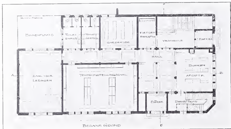
PLATTEGRONDEN BIJ-BIBLIOTHEEK, MOTTO: „ENFIN”. — VERHOOGDE DERDE PRIJS A. A. VAN NIEUWENHUIZEN EN C. HOOGENDIJK, ROTTERDAM.
