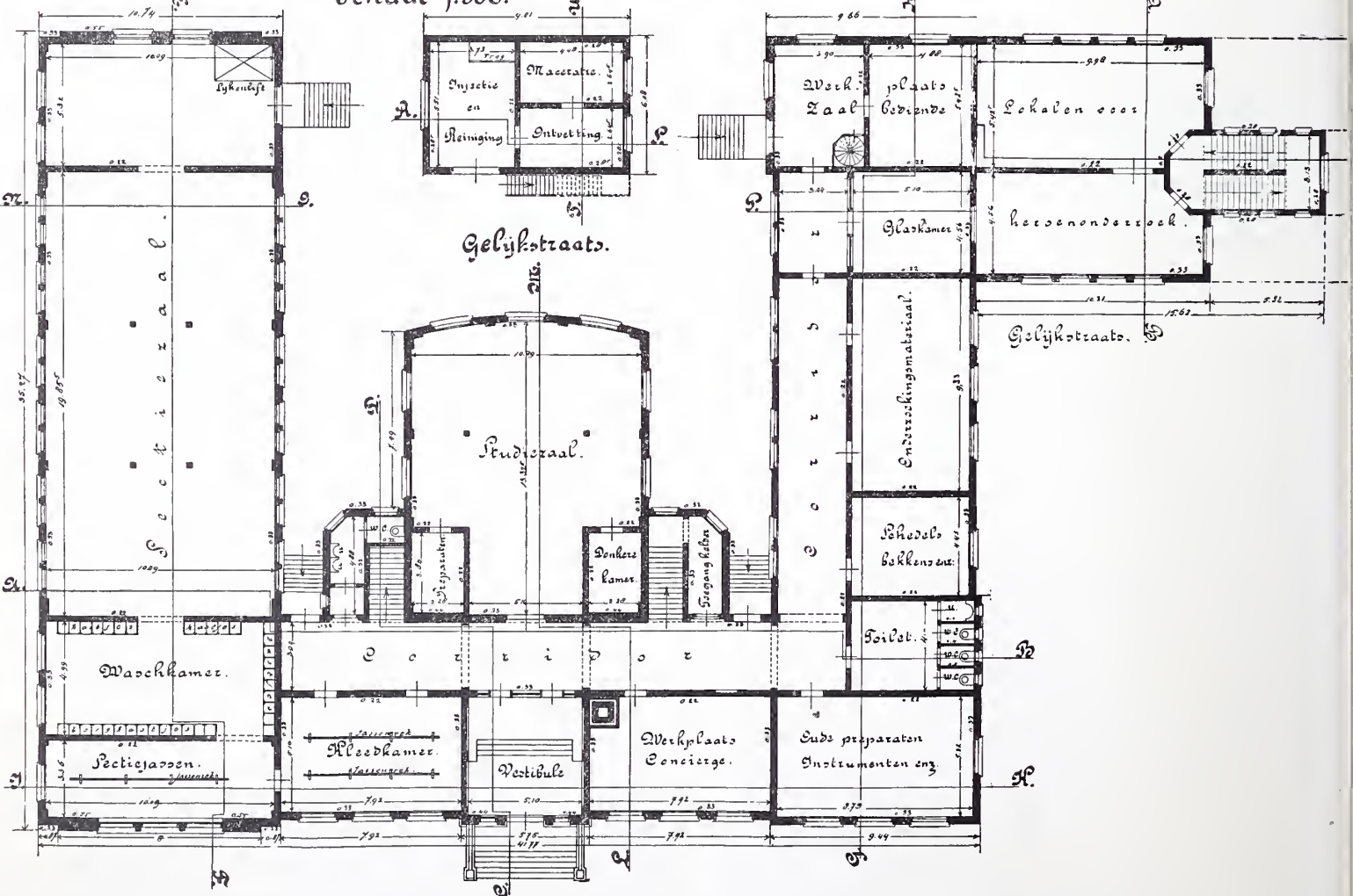
HET ONTLEEDKUNDIG LABORATORIUMGEBOUW DER GEMEENTELIJKE UNIVERSITEIT TE AMSTERDAM.
