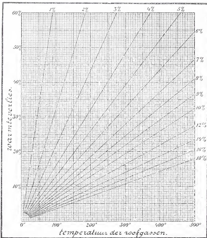
De getallen, geschreven bij de uiteinden der schuine lijnen, geven aan het koolzuurgehalte der rookgassen.
