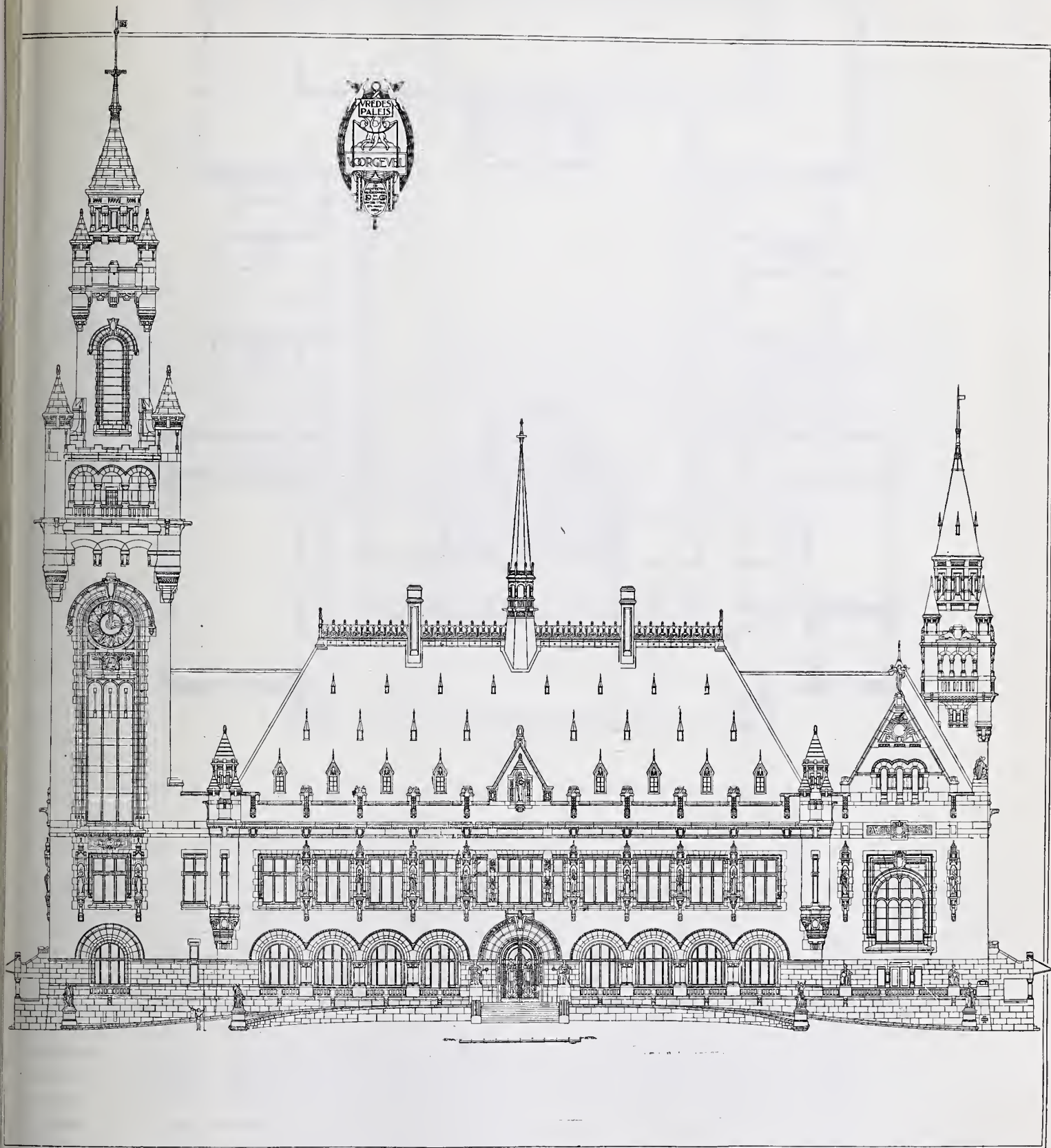
VOORGEVEL VAN HET VREDESPAELIS.
