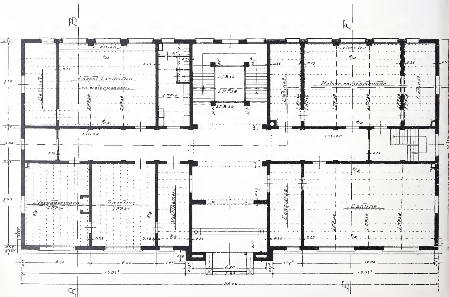
PLAN BEGANEGROND EN PLAN 2DE ETAGE. — Schaal 1 à 200*.) Architect A. W. C. DWARS. (Plan 1ste etage = plan 2de etage; echter bevinden zich onder het leeslokaal links van het trappenhuis een leeszaal en W. C.)
