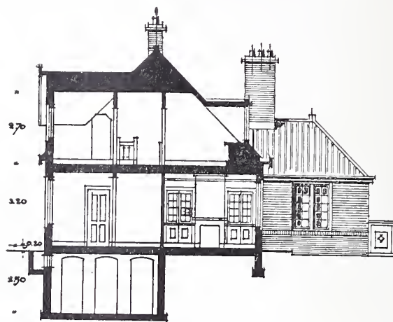
DWARS DOORSNEDE.
