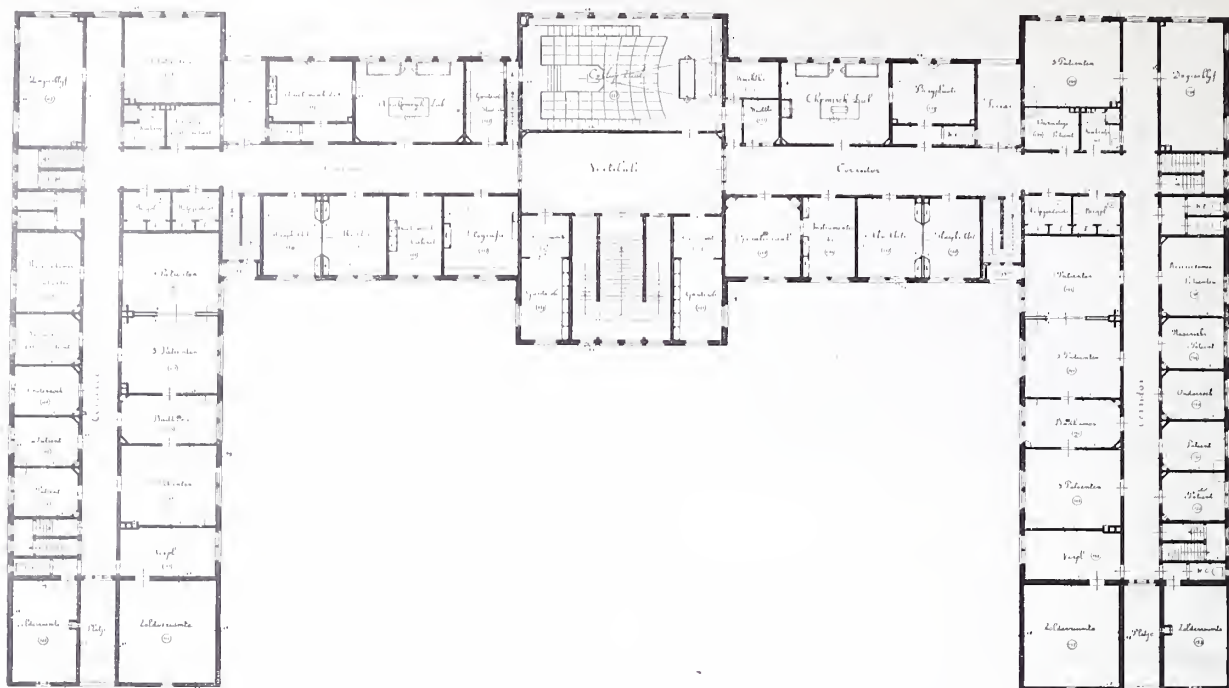
KLINIEK VOOR PSYCHIATRIE EN NEUROLOGIE TE AMSTERDAM. 1ste ETAGE. H. BONDA, Architect.
