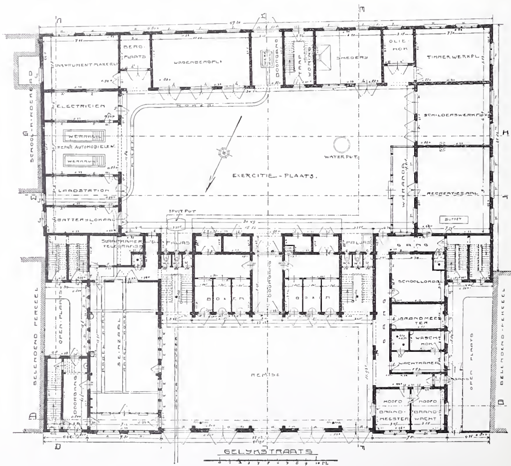
HET NIEUWE CENTRAAL BUREAU. HOOFDWACHT VOOR DE BRANDWEER TE AMSTERDAM.
