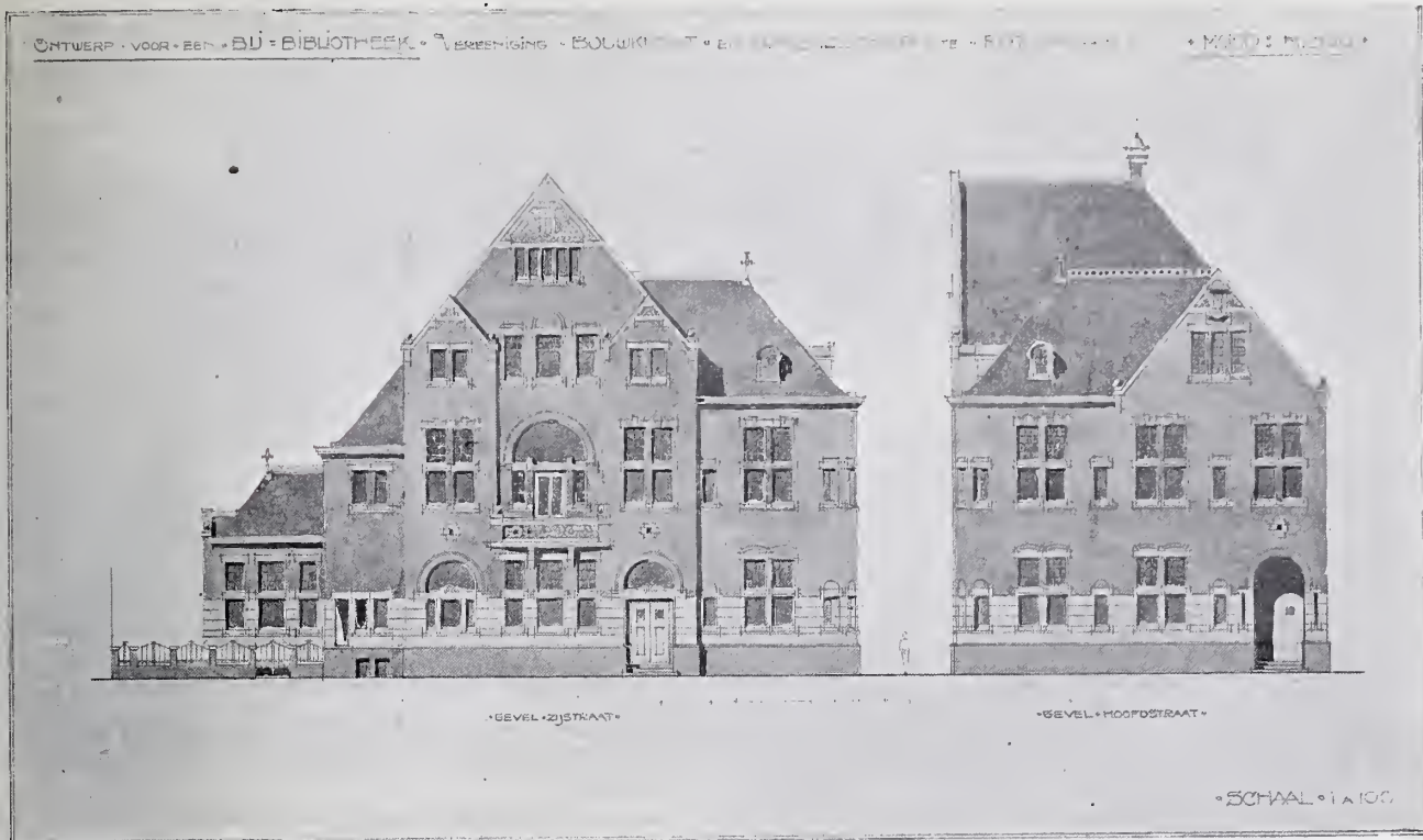
GEVELS BIJ-BIBLIOTHEEK, MOTTO: „HIBOU”. — VERHOOGDE DERDE PRIJS CHARLES ESTOURGIE, AMSTERDAM.
