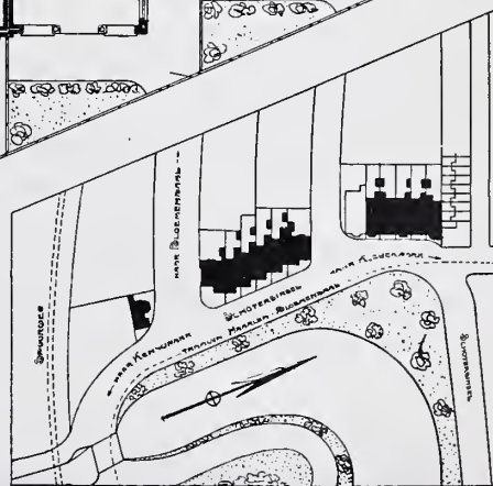
SITUATIE
