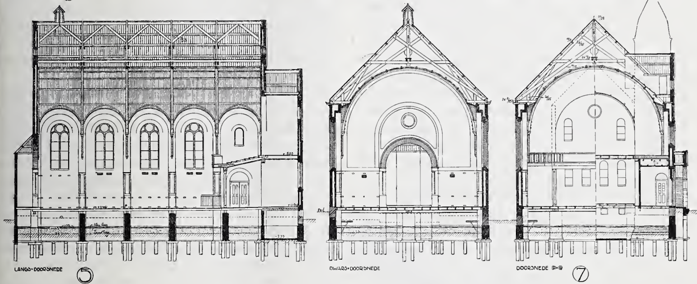
KERK VOOR DE AFDEELING VAN DEN NED. PROTESTANTEN BOND TE SCHIEDAM.
