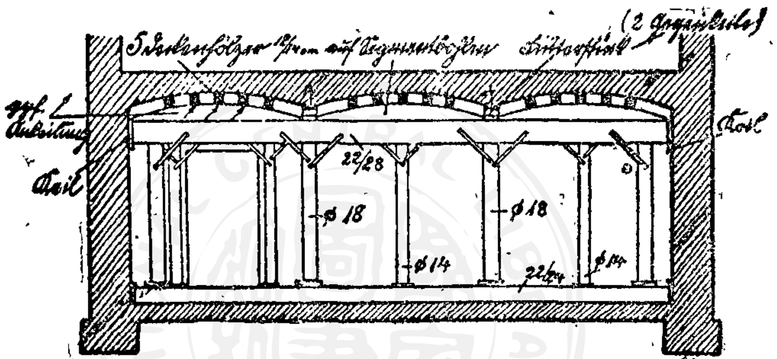
(其一) 橫剖面
