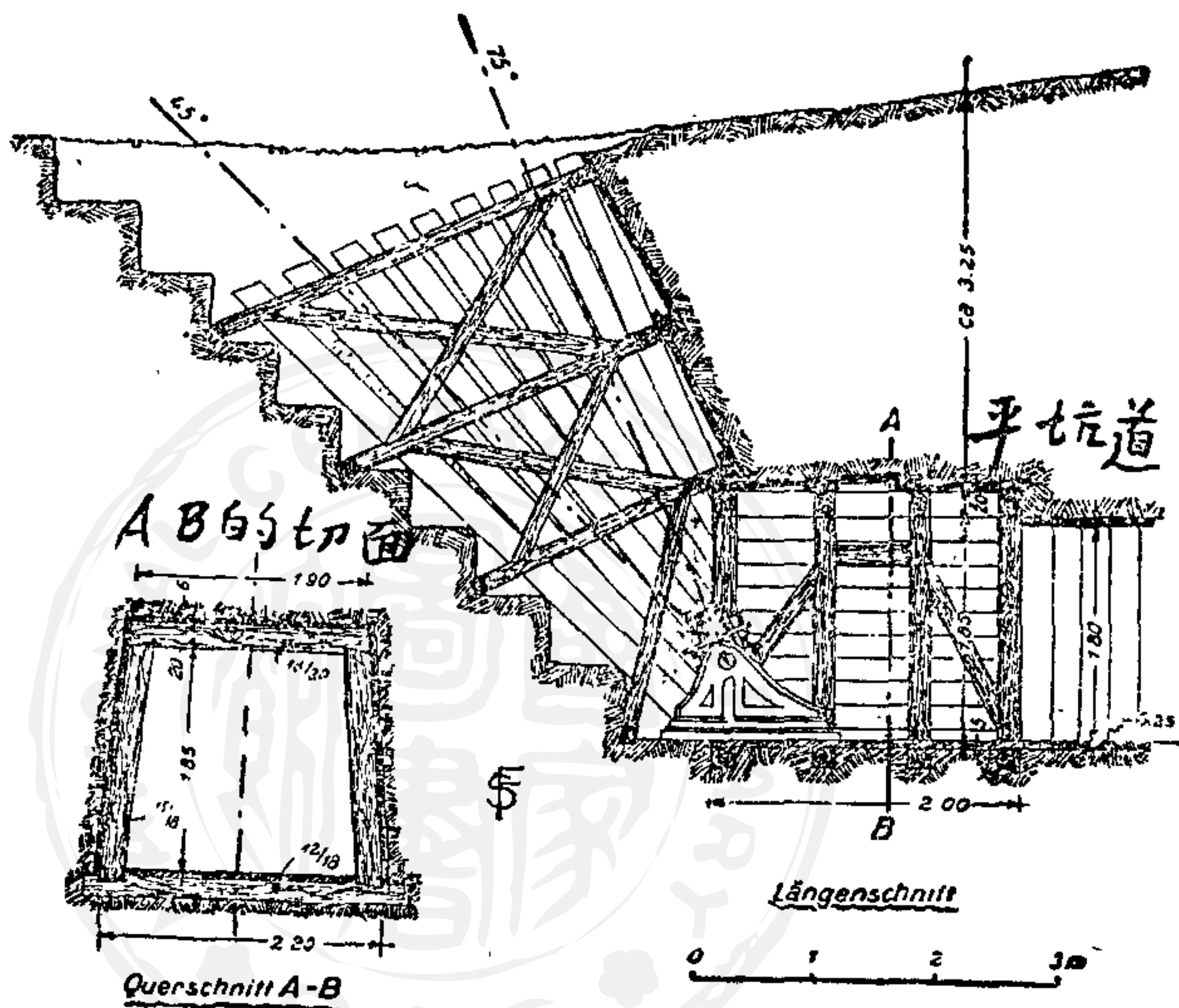
平坑道 ( 築圖 15 ) 坑道口為迫擊砲陣地
