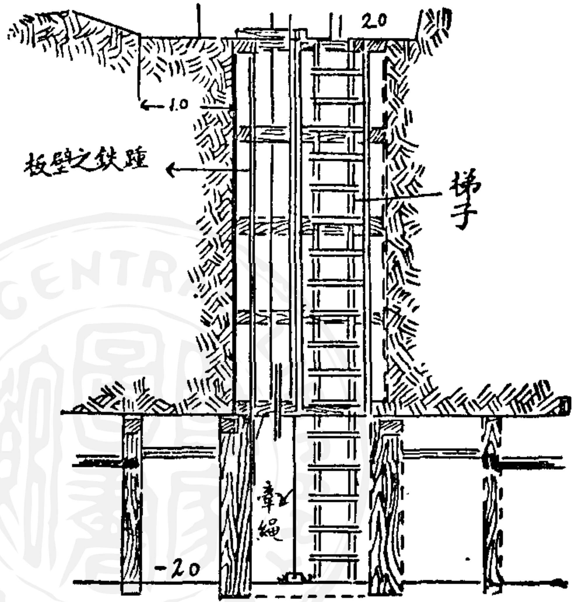
(築圖 13) 垂坑道之一例
