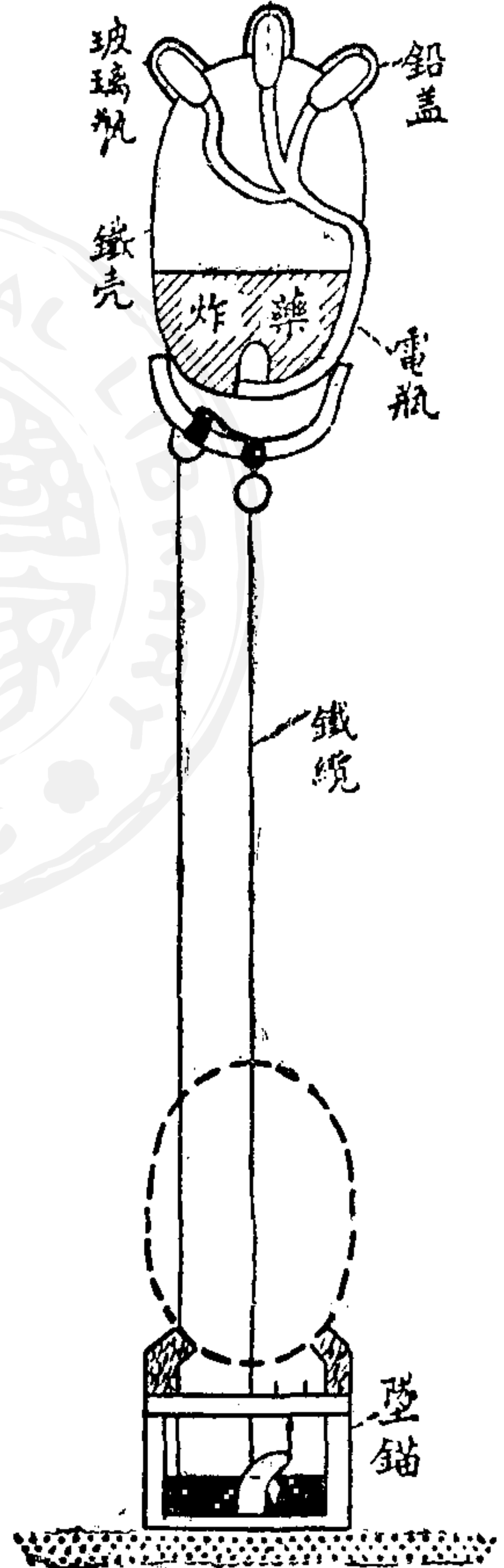
(海圖 10)
