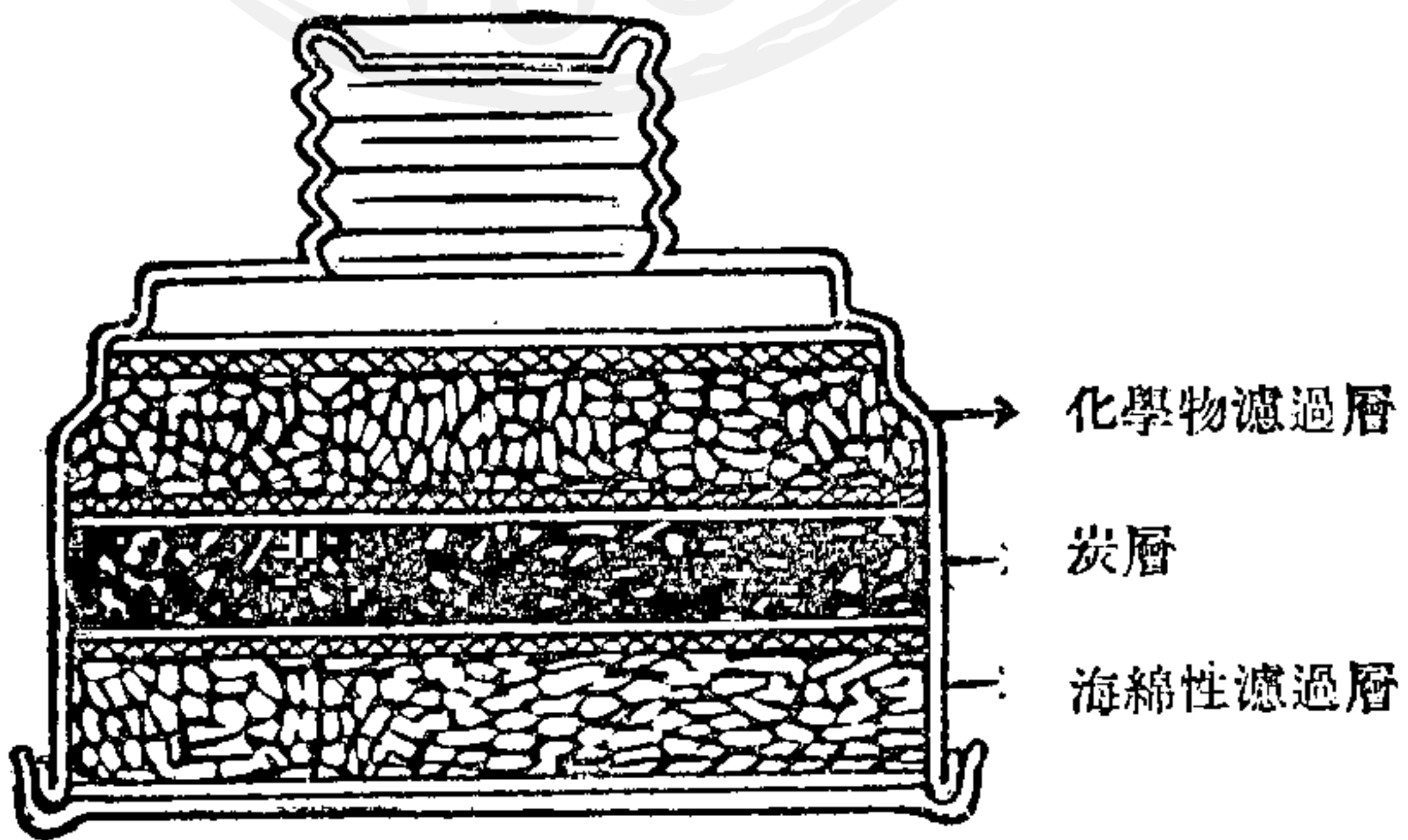
三層式濾毒罐剖面 ( 防毒圖 3 )
