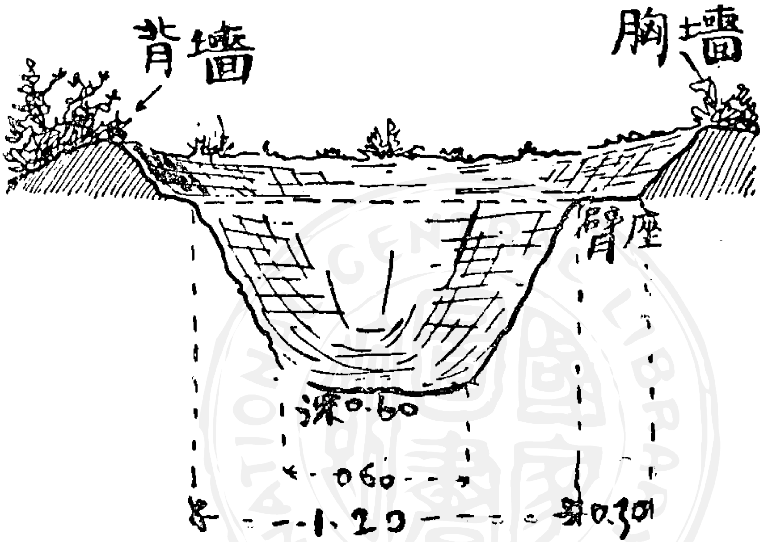
A. 跪射散兵坑
