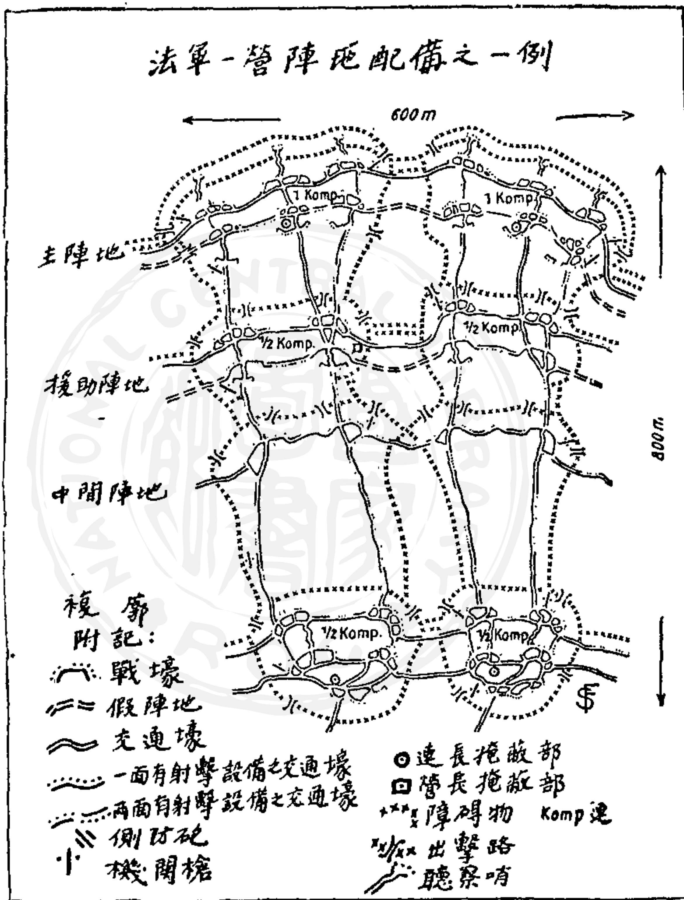
( 築圖 12 )
