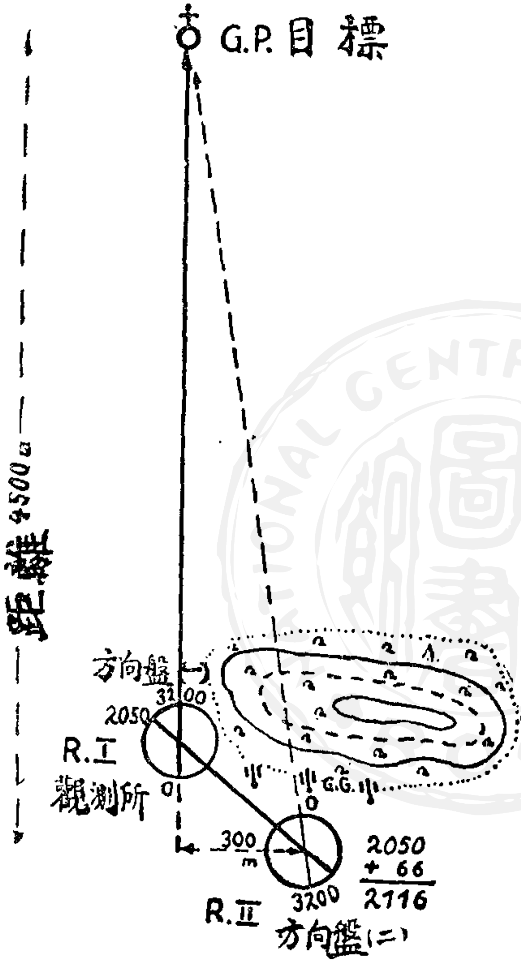
用一個方向盤間接瞄準法 (砲圖 5)
