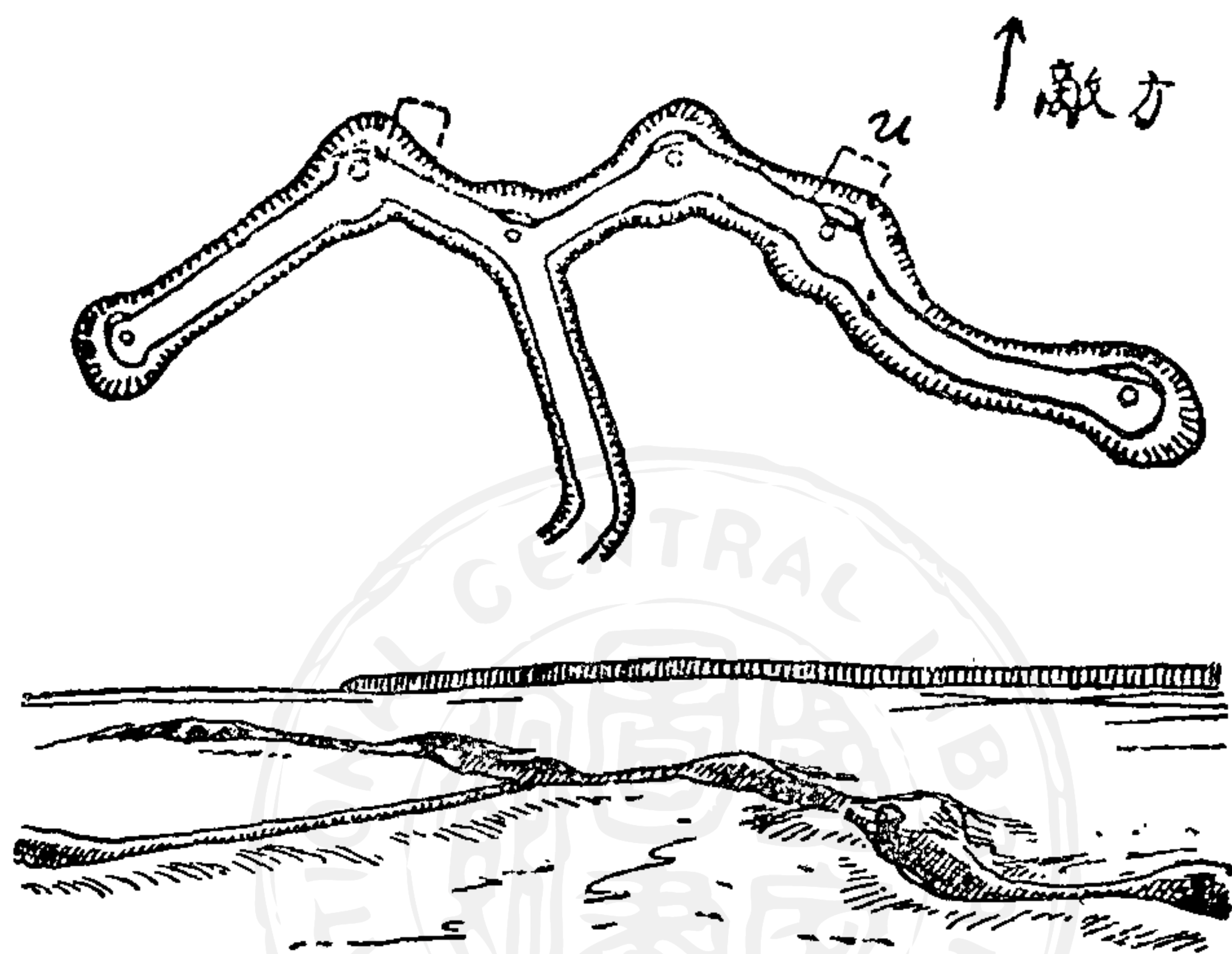
(築圖 7) B. 班陣地之一例
