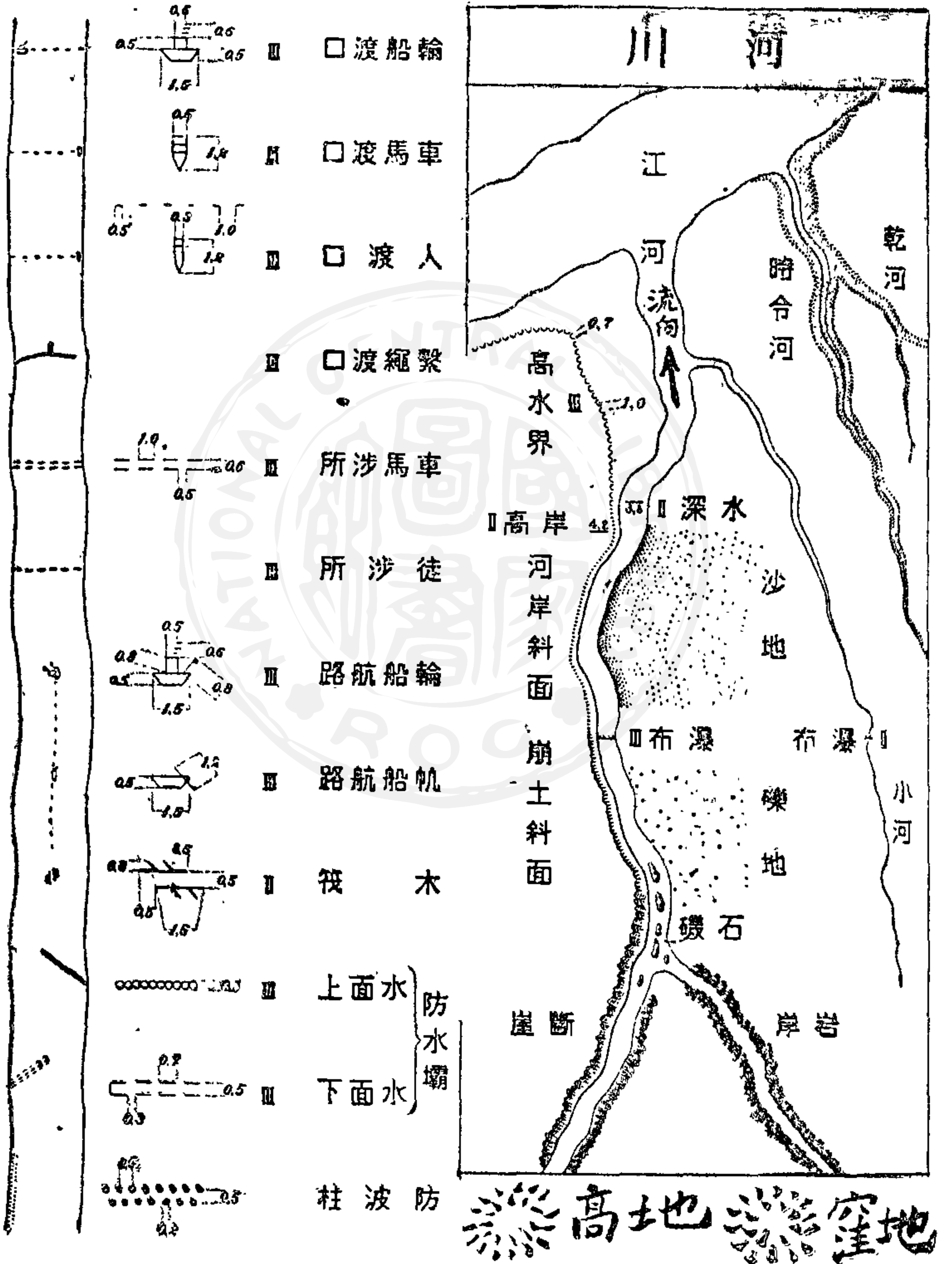
(步圖 13)
