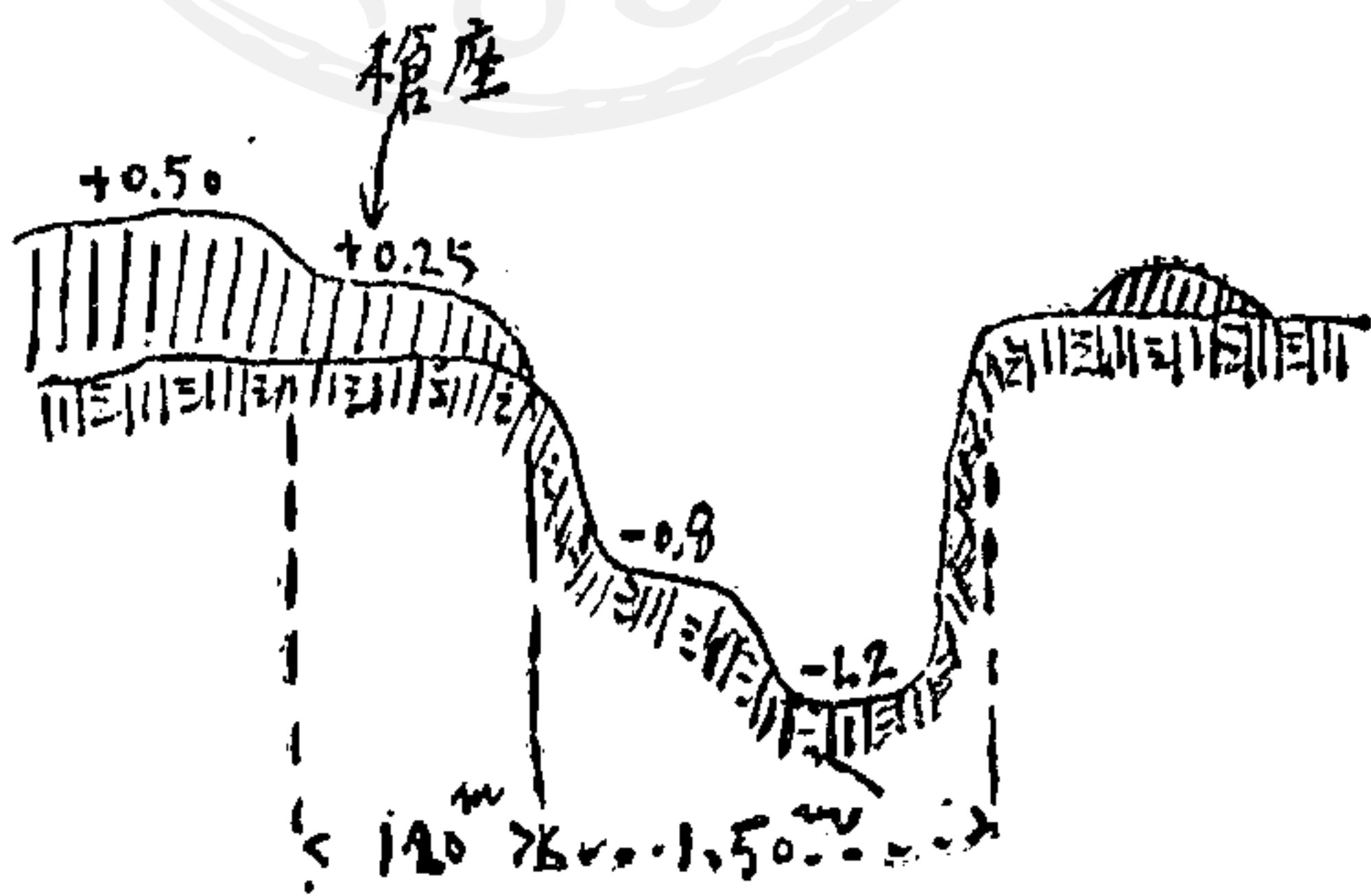
B. 陣地上之輕機關槍掩體
