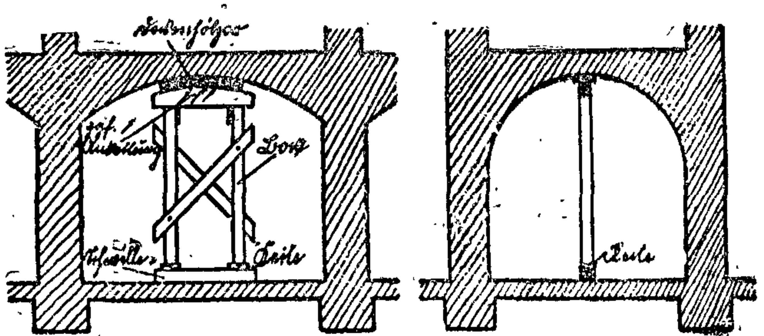
(其二) 縱剖面
