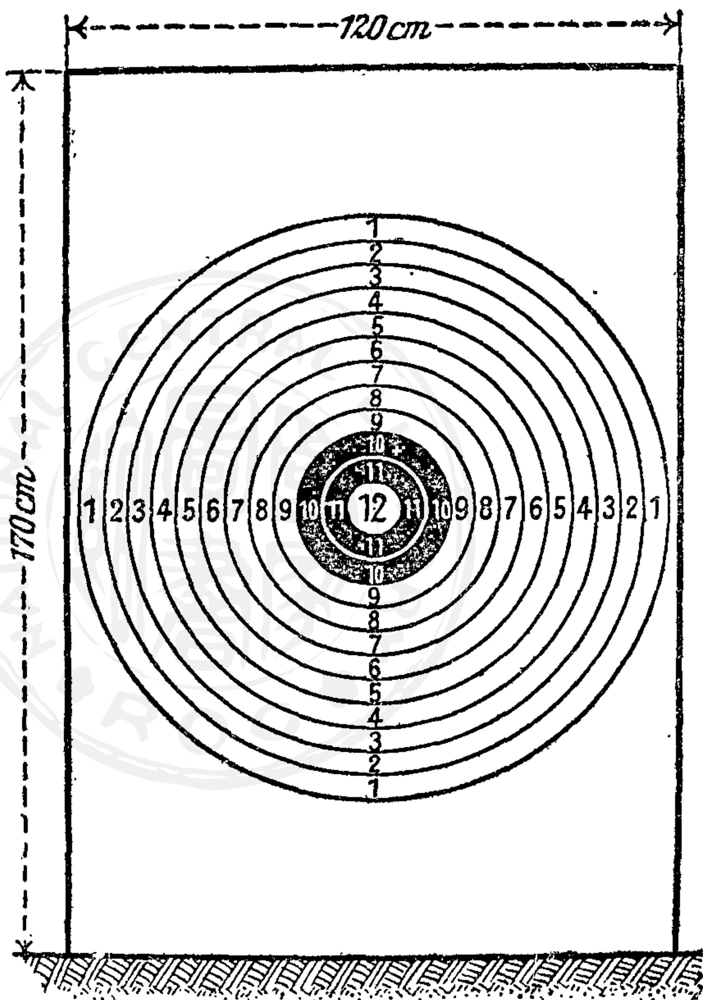
(射圖 6)
