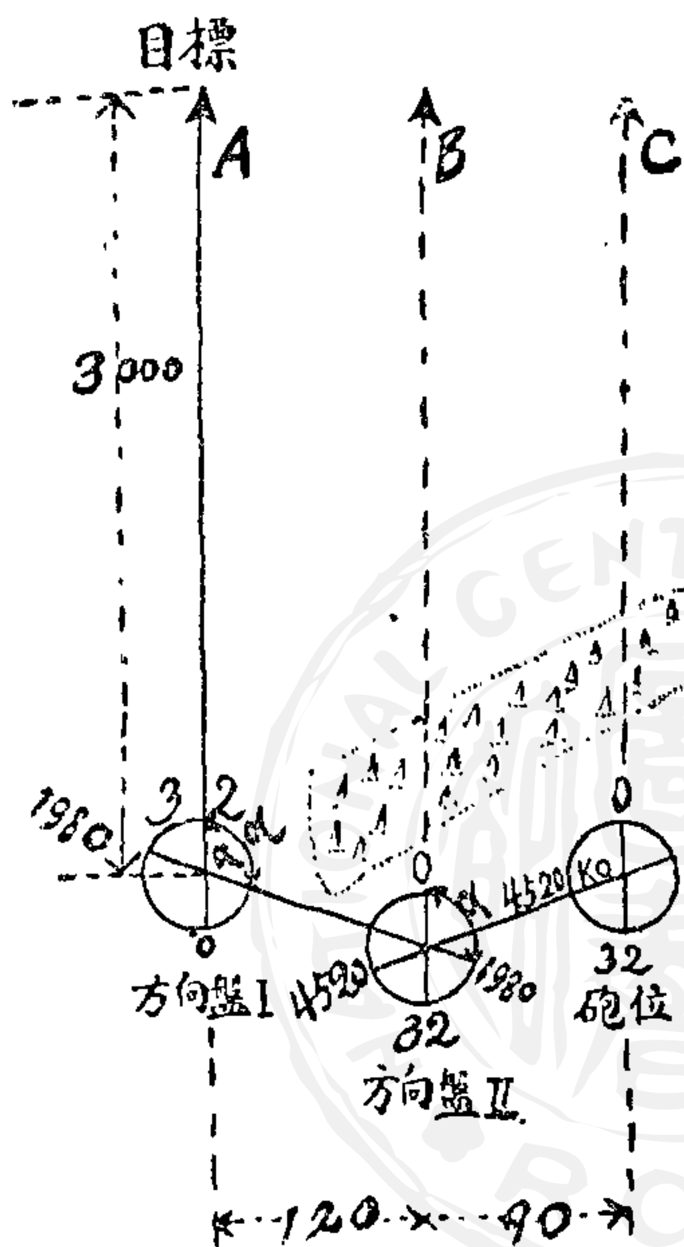
(砲圖 6)
