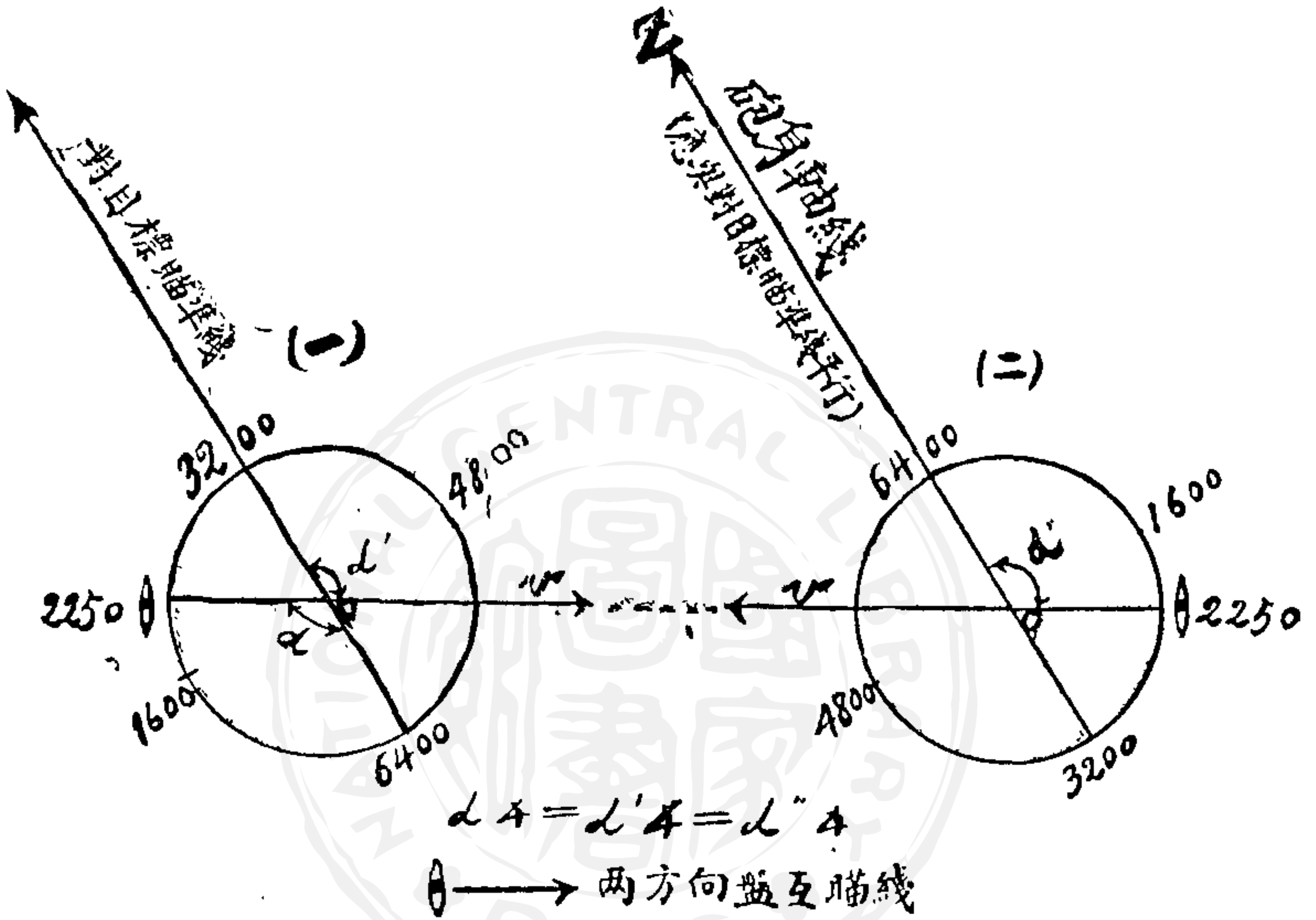
(砲圖 3)
