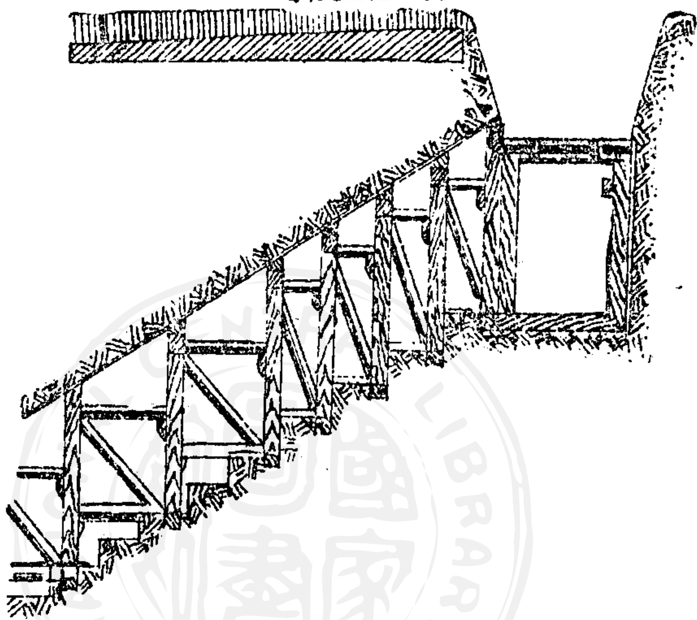
斜坑道之一例
