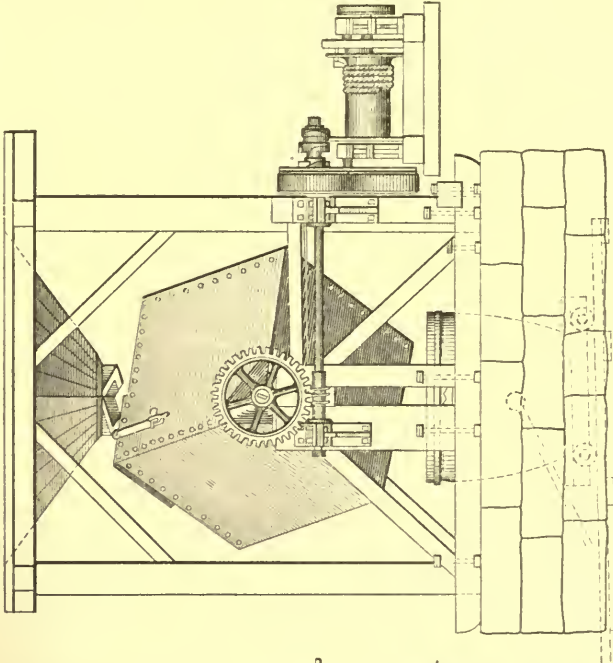
END ELEVATION
