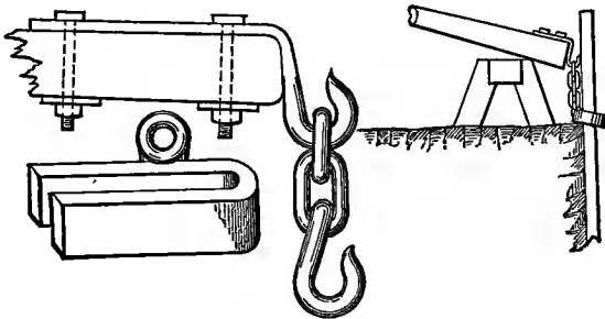
FIG. 18.—SHEATHING-PULLER.
