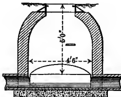
FIG. 2. SHALLOW MANHOLE.
