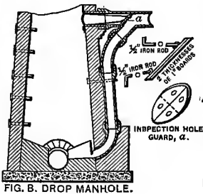
FIG. B. DROP MANHOLE.
