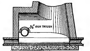
FIG. 3. SHALLOW MANHOLE.
