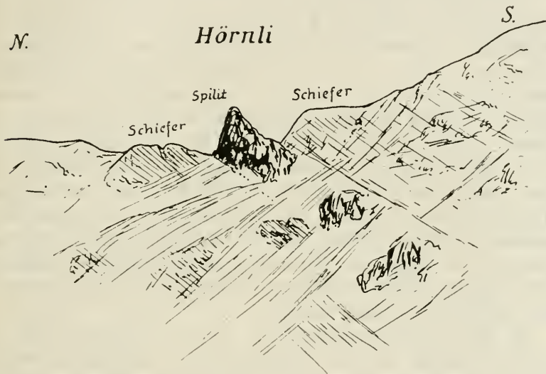
Fig. 4. Das Hörnli von Westen gesehen (nach Photographie des Verfassers) Spilit concordant zwischen liassischen Schiefem gelegen.
