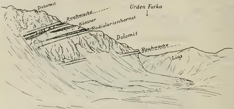
Fig. 16. Die Ueberschiebung der unteren Scholle des Parpaner Weisshornes (jüngere Rauh- wacke , Hauptdolomit , Kössner — mit Lias - und Radiolarienhorn- stein -Fetzen —) über den Lias der Urden-Furka , sowie der oberen Schuppe (jüngere Rauh- wacke und Hauptdolomit über die untere). (Nach Photographie des Verfassers.)
