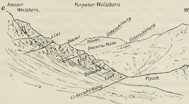
Fig. 2. Skizze der Schuppen des Arosaer Weisshornes sowie der Ueberschiebungen des Parpaner Weisshornes. Die Hauptueberschiebung (über Flysch) nur im Vordergrund sichtbar. Gez. nach einer Photographie des Verfassers.
