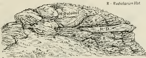
Fig. 19. Block am Ostabhang des Brüggerhornes . Länge ca. 6 m. (Nach Photographie des Verfassers.)
