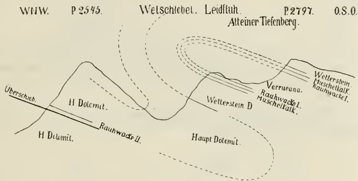
Fig. 6. Profil durch die Strela-Amselfuhfalte, Schafsrücken-Erzhornfalte etwas südwestlich vom Profil No. 5. Massstab ca. 1 : 40 000.
