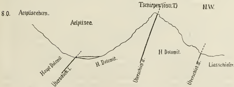
Fig. 13. Massstab ca. 1 : 25 000. Drei Parallelschnitte durch das Keilstück des Parpaner Weisshornes-Tschirpen. Besonders gewählt zur Erklärung des verdreifachten Hauptdolomits an der Schnittlinie Aelpliseehorn-Tschirpen.
