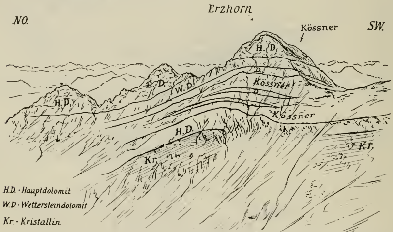
Fig. 10. Eine Face-Ansicht der Erzhornkette (nach Photographie des Verfassers) vom Aelpliorn gesehen. Zeigt das kurze horizontale Ausmass der Einspitzungen der N.-W.-Wand des Erzhornes.
