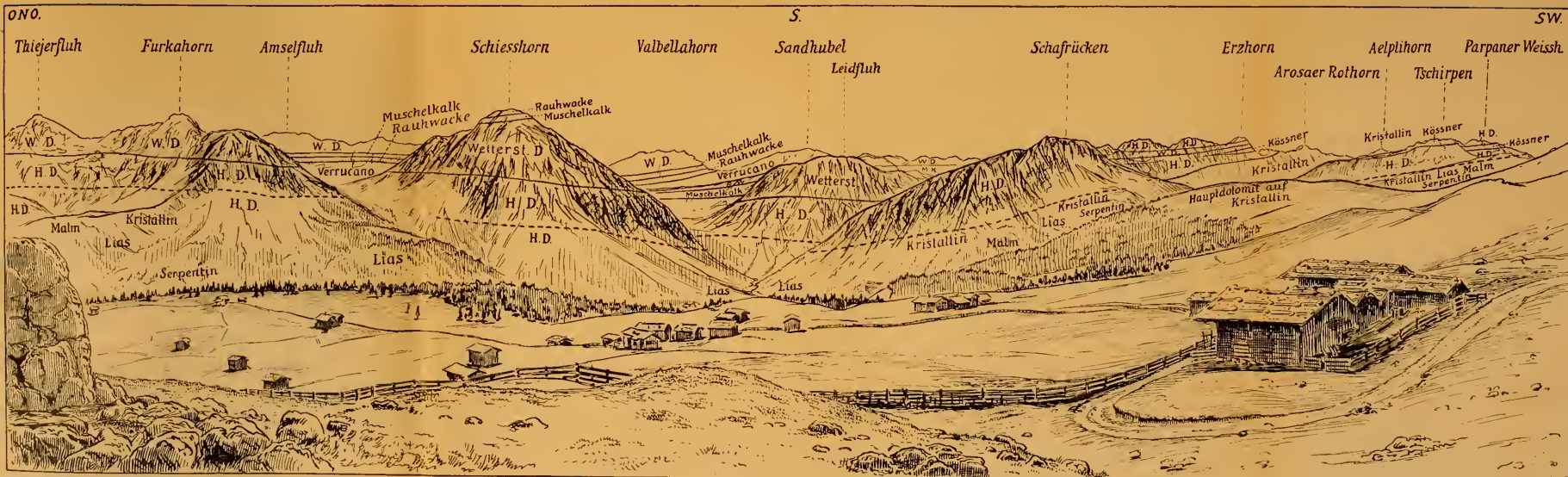
Strela-Amselfluhkette und Schafrücken Erzhornkette („Zone normaler Faltung“), sowie Tschirpen und Parpaner Weisshorn („Zwischenstück“) von Maran gesehen. Im Vordergrund das Plateau von Arosa („Anbruchzone“).
