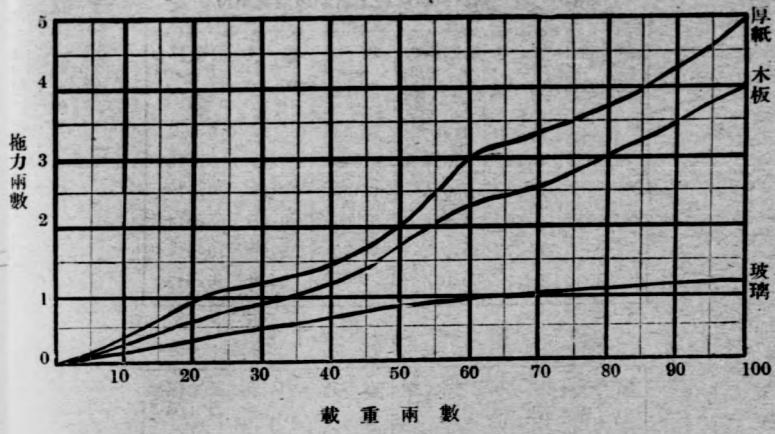
第五圖 載重與拖力之關係
