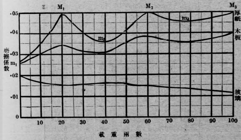
第六圖 載重與摩擦係數之關係
