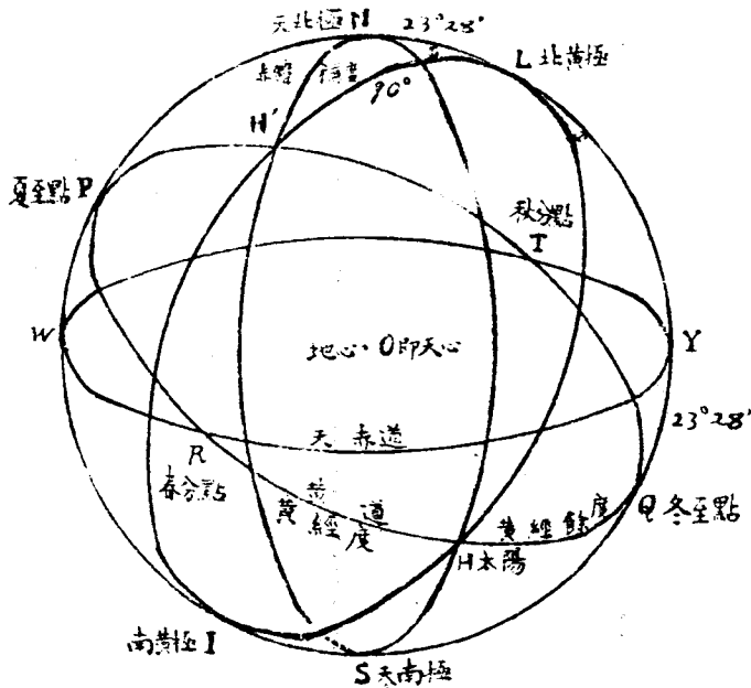
附註：本圖表以 \angle NLH = 黃經餘度 QH (= PH) 推定赤緯補度 NH 之法。
