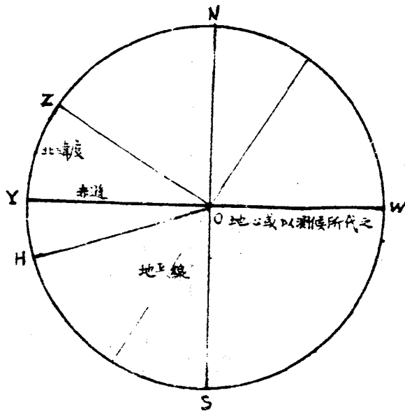
附註：本圖表太陽在赤道南時（冬至前後）以 NH 求北緯度 ZY 之法。
