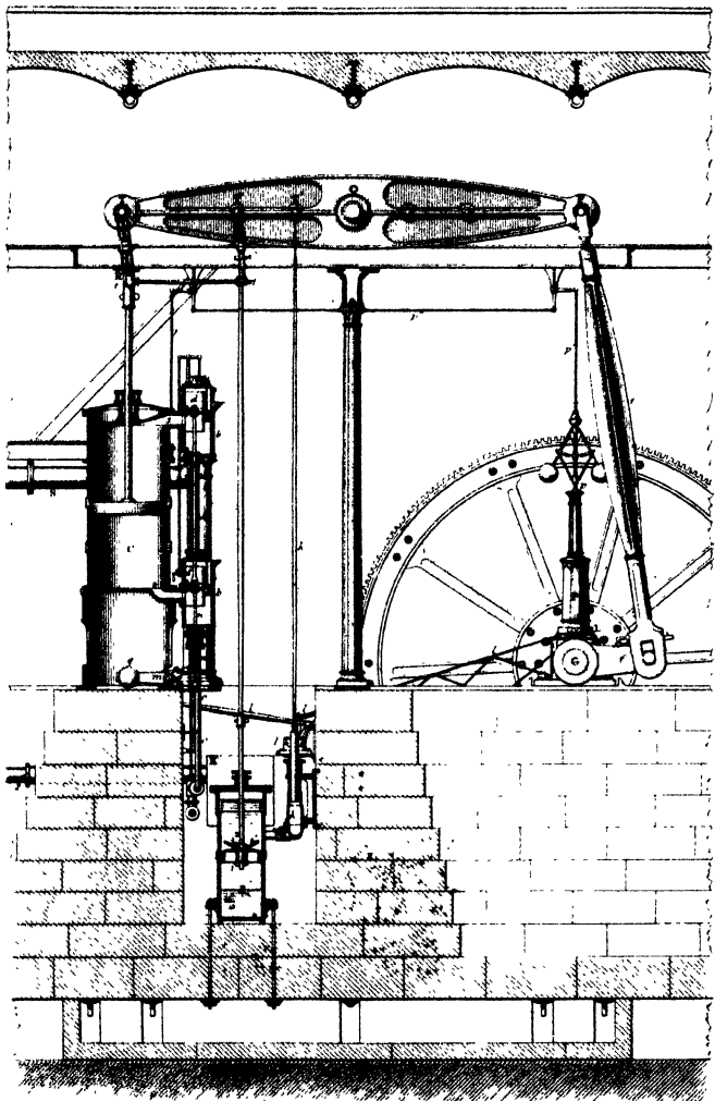
Longitudinal Section
