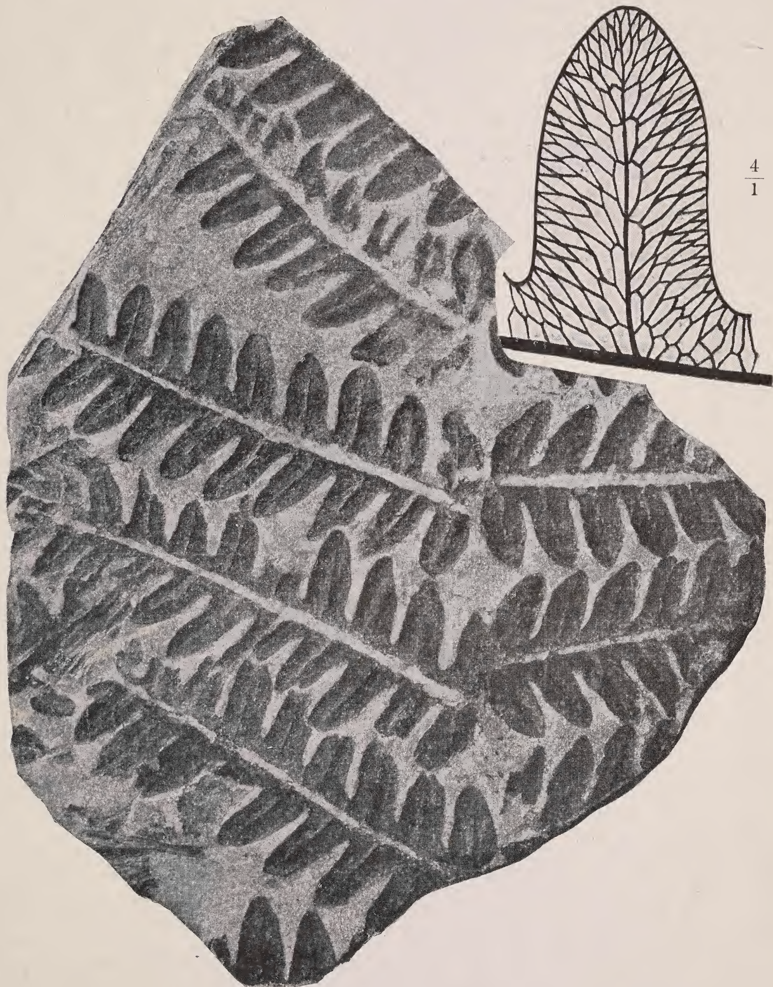
Fig. 1. Lonchopteris Bricei .
