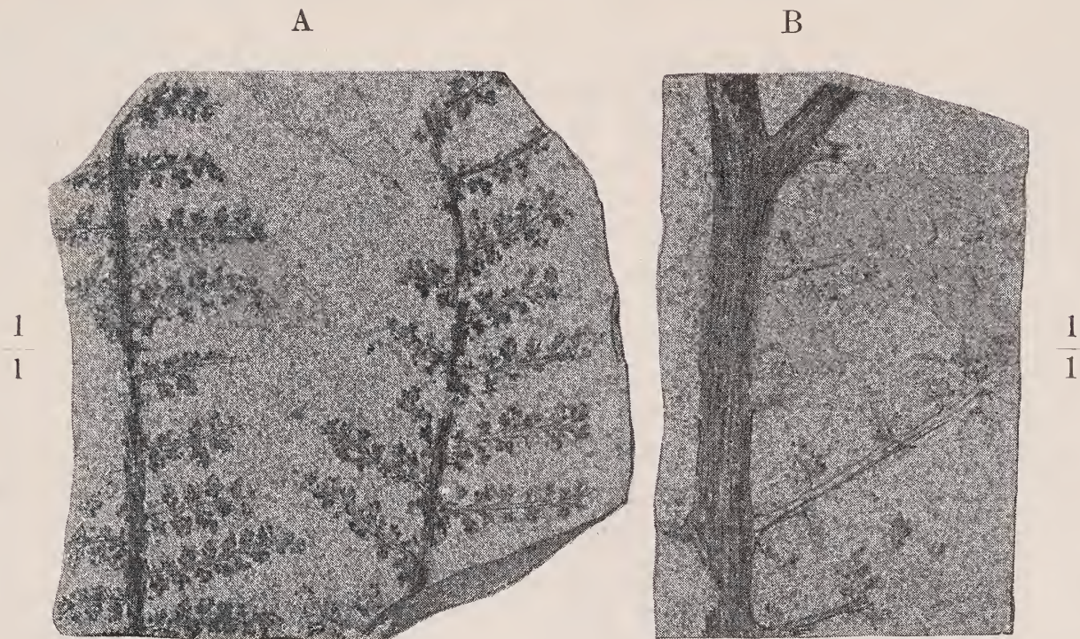
Fig. 1. Callipteris Moureti .
