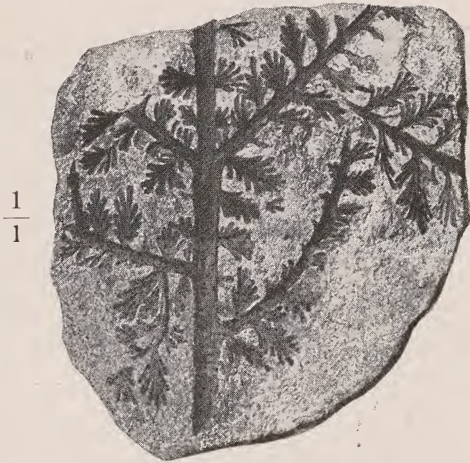
Fig. 2. Callipteris Raymondii .
