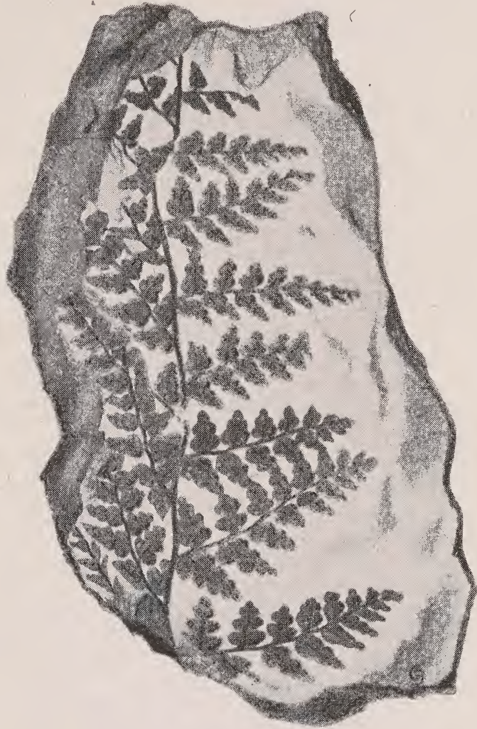
Fig. 3. Sphenopteris Laurenti .
