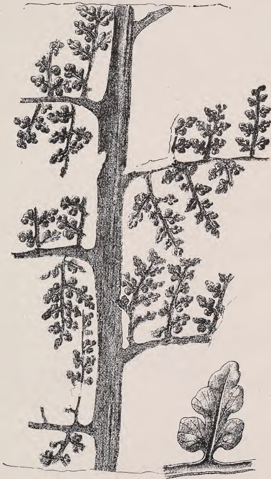
Fig. 1. Sphenopteris trigonophylla .
