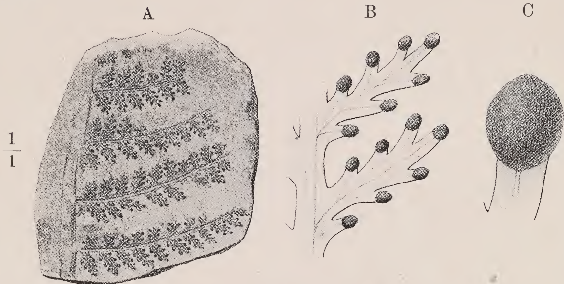
Fig. 3. Owopteridium Gutbierianum .
