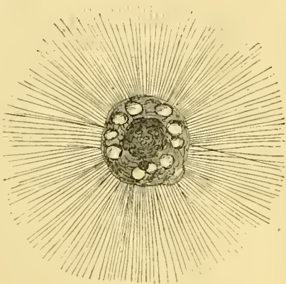
Fig. 12.— Actinophrys sol .
