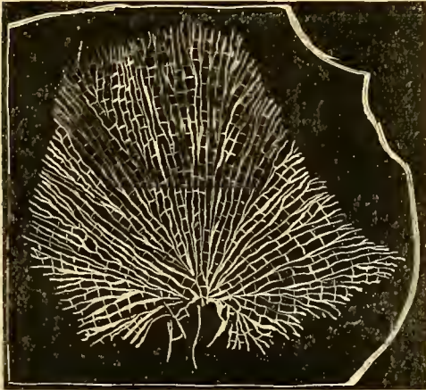
Fig. 90.— Fenestella plebeia .
