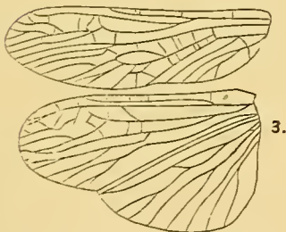
Fig. 18.— Dictyopteryx microcephala .
