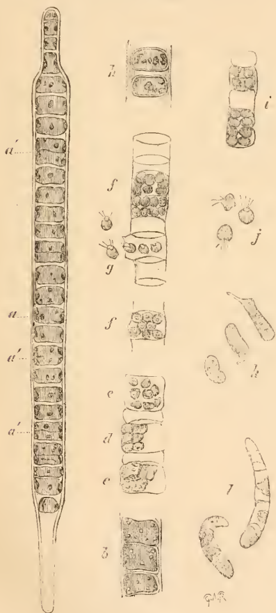
Fig. 110. Ulothrix.
