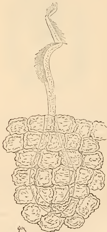
Fig. 115. Chatospira Mülleri × 380.
