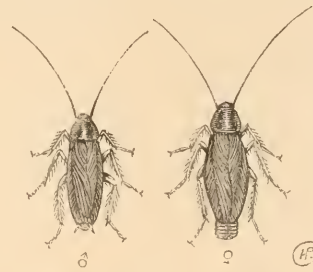
Fig. 9. Ectobius Germanica .
