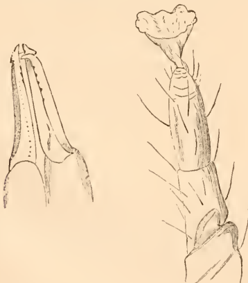
Fig. 223. Proboscis.
