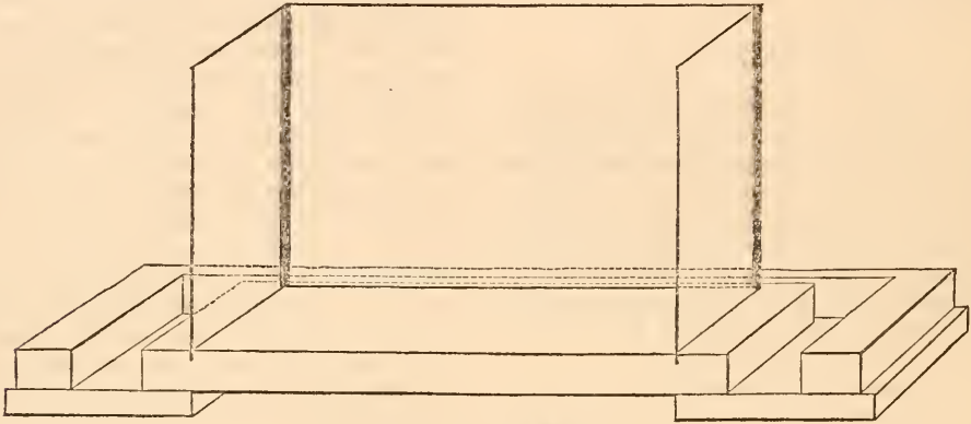
Fig. 195. THE FORMICARY.
