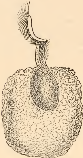
Fig. 116. Chatospira mucicola × 380.
