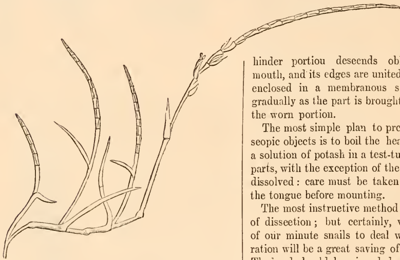
Fig. 206. Lepturus incurvatus .
