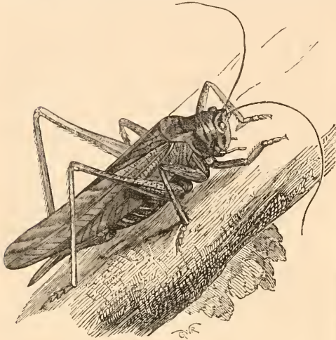
Fig. 198. Acrida viridissima.
