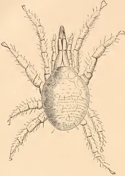
Fig. 222. Mole Mite.
