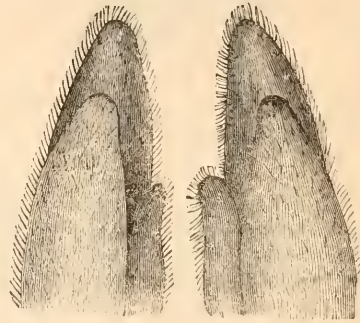
Fig. 123. Spinnerets.
