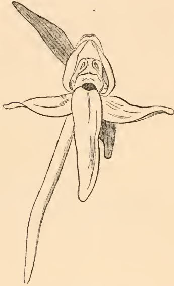
Fig. 166. Habernaria chlorantha .
