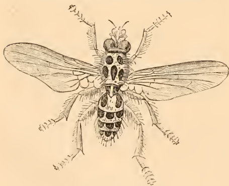
Fig. 247. Anthomyia pluvialis .
