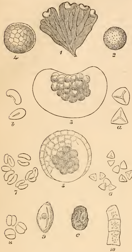
Fig. 197. Fern Spores.
