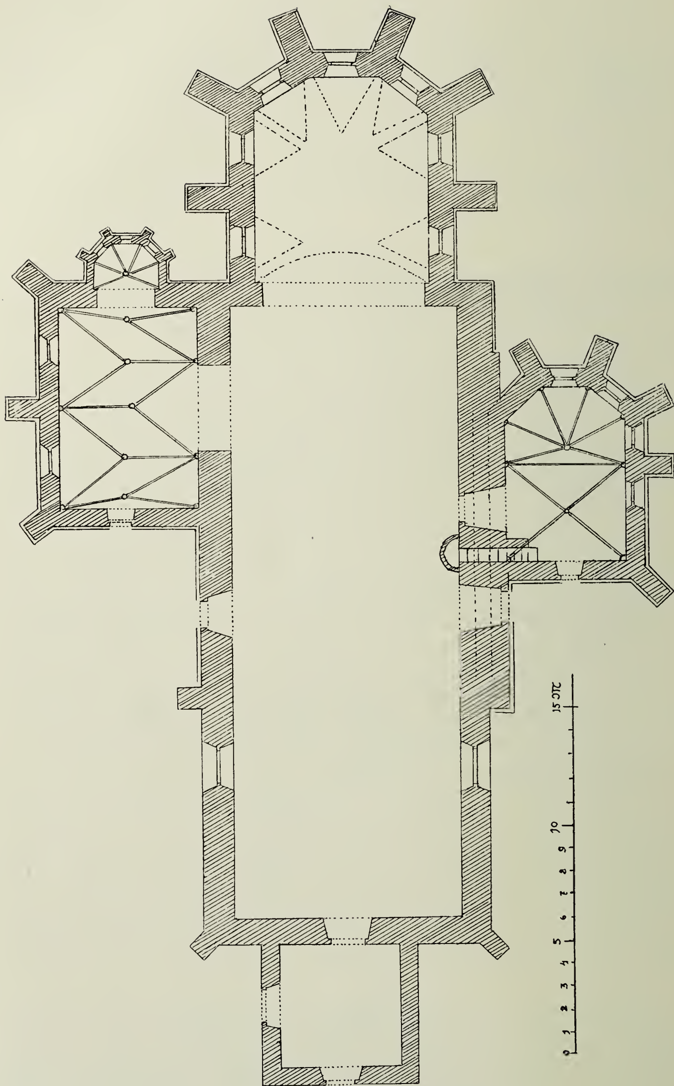
Obr. 27. Půdory kostela v Sezemicích.
