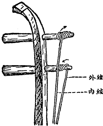
(圖十七) 胡琴絃索旋轉之方向 (箭頭示卷軸之方向)
