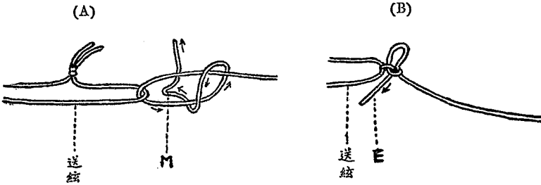
(圖十六) 活結之挽法
