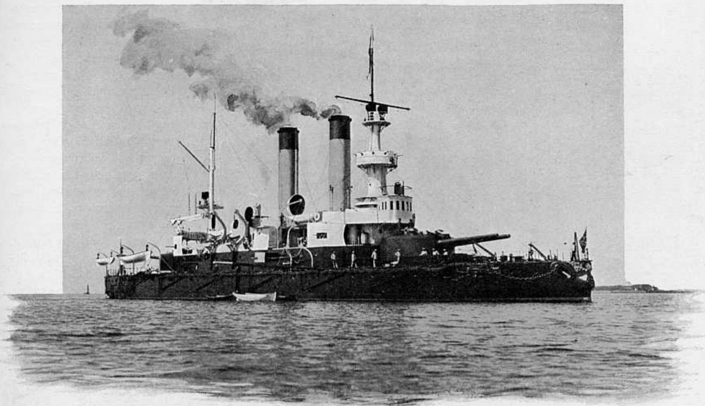
БРОНЕНОСЕЦЪ «ГЕНЕРАЛЬ-АДМИРАЛЬ АПРАКСИНЪ».
