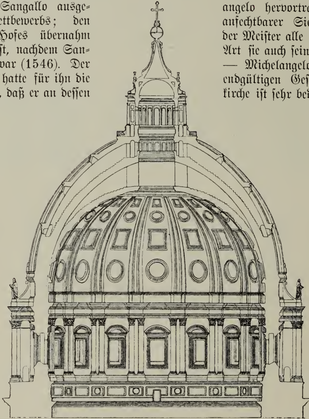
Abb. 75. Durchschnitt von Michelangelos Modell für die Kuppel der St. Peterskirche in Rom.
