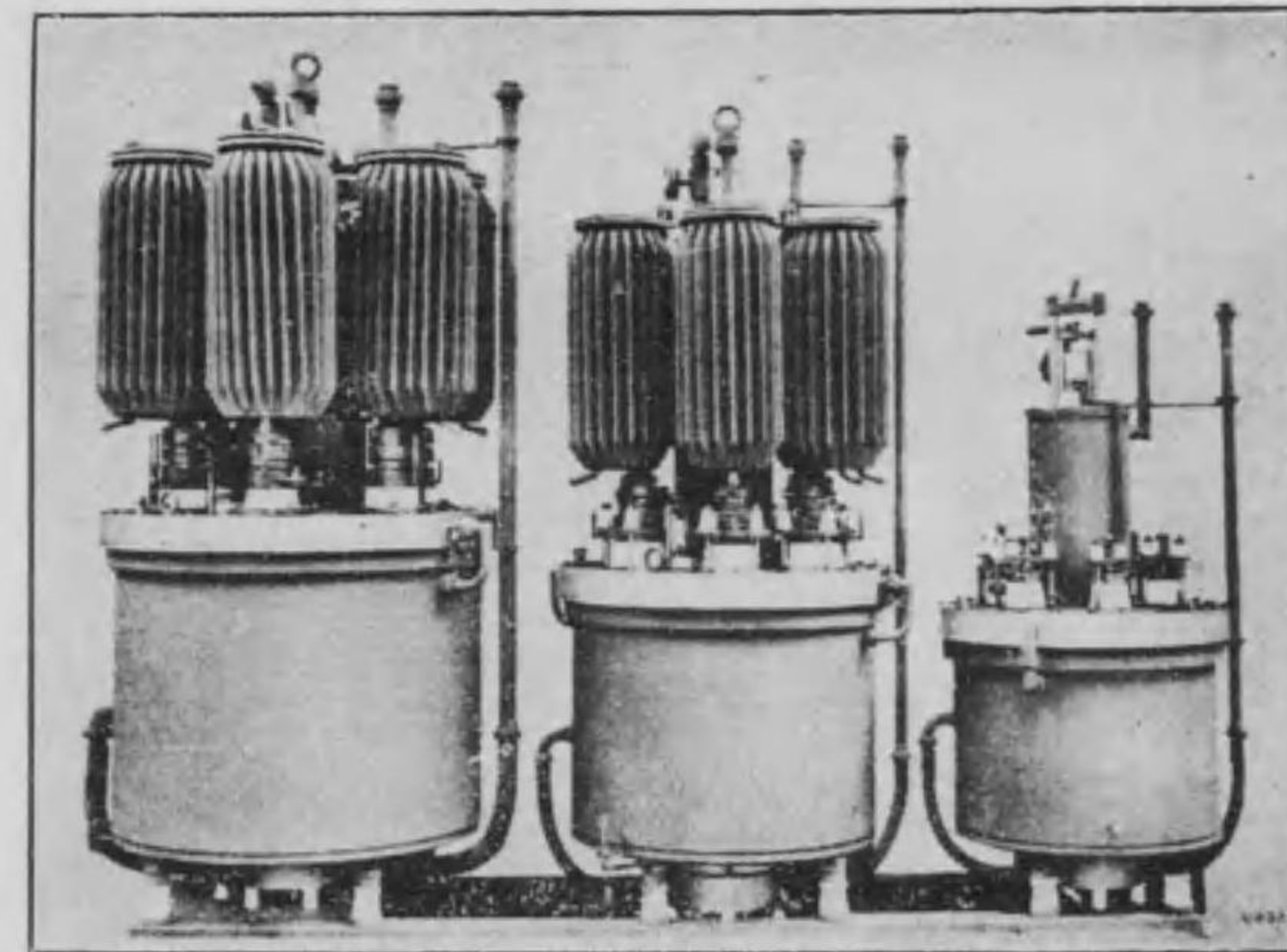
D.C. 750A, 1200V. 500A, 1200V. 250A1200V.
