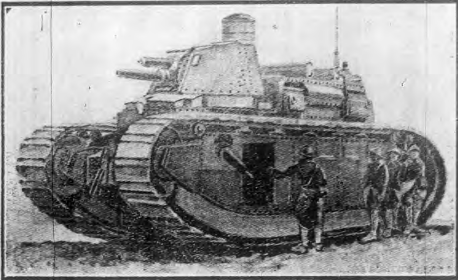
法國之重克車：此車重六十八噸。車上裝有野砲數門及機關槍多架。
