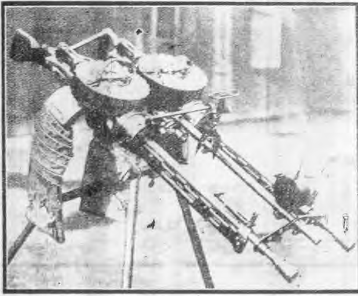
左：世界最新式之捷克斯拉胡飛機 上用之變管機關槍，據云每分 鐘可發出九百子彈。
