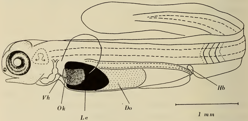
FIG. 13. — Perca , 4. pT.
