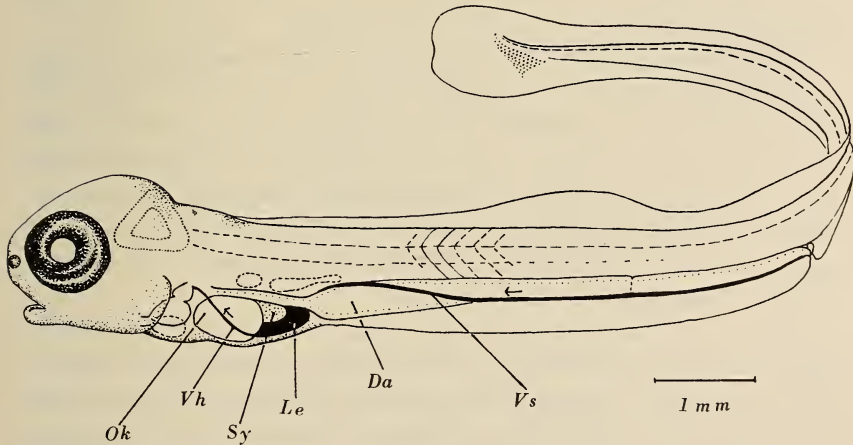
FIG. 3. — Coregonus , 25. pT.
