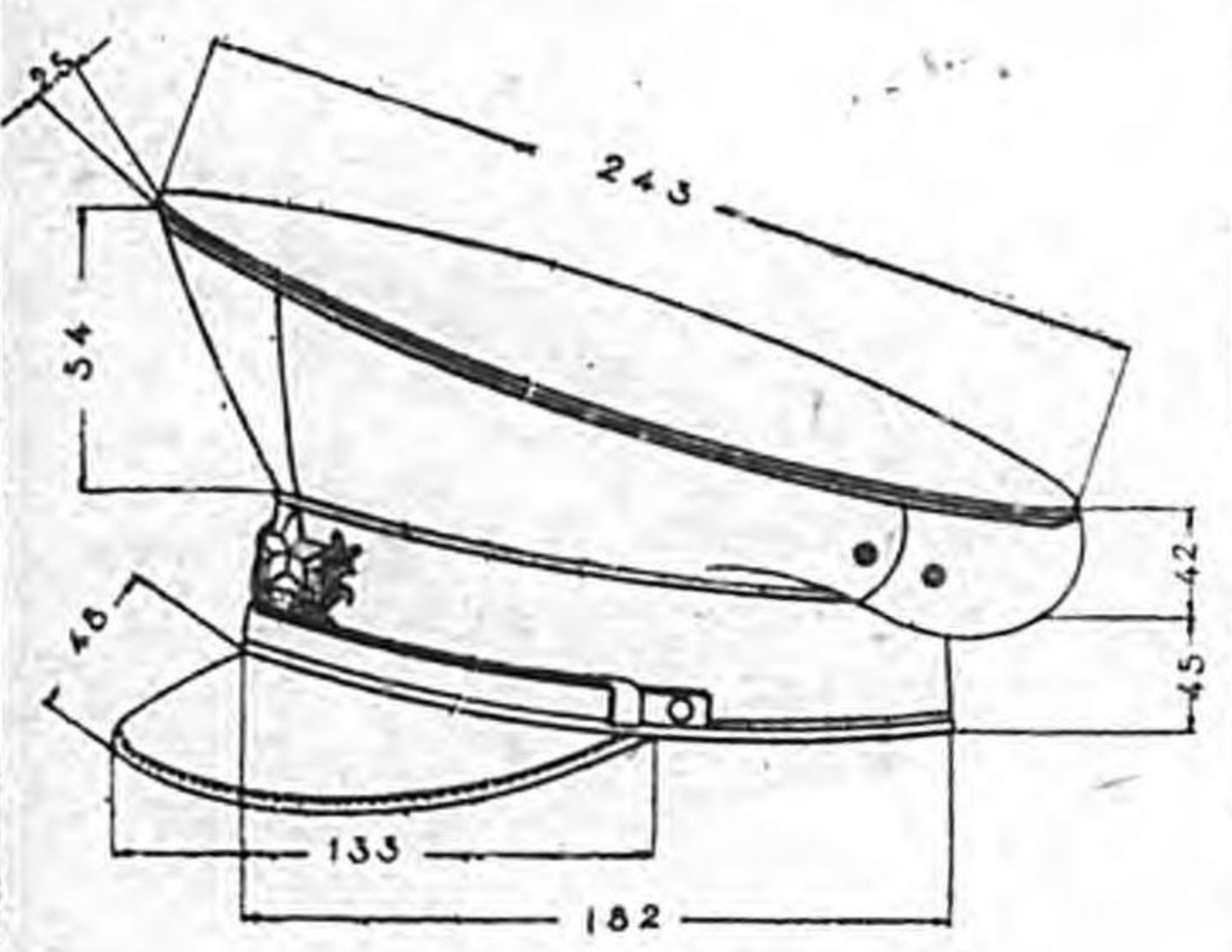
第四圖 軍帽 (衞軍軍帽) (寸法耗)
