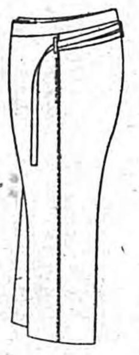
第九圖 夏禮袴 (寸法耗)
