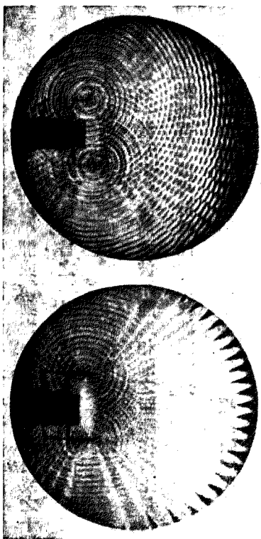
圖二 紋波之干涉
