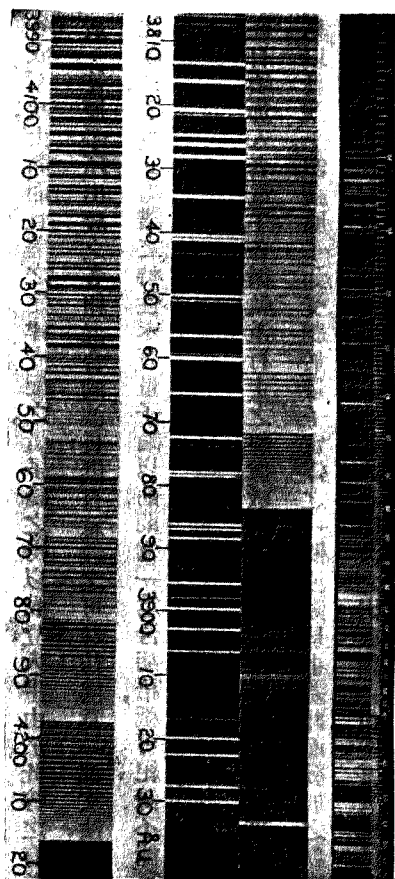
圖七 各式光譜
