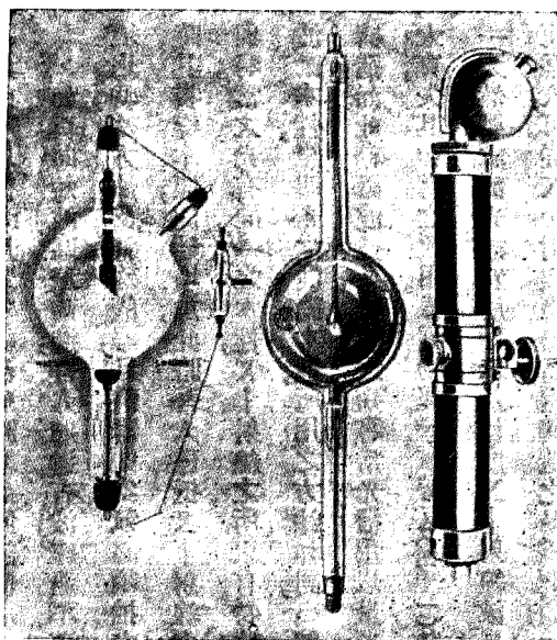
圖五 X-射線管
