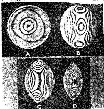
圖三 光學工業中干涉方法之應用
