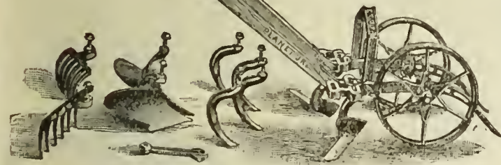
PLANET JR. DOUBLE WHEEL HOE.
