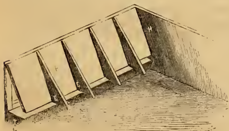
Fig. 2.—FRONT PARTITION.
