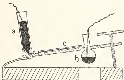
Fig. 8. Kapillarelektrometer.
