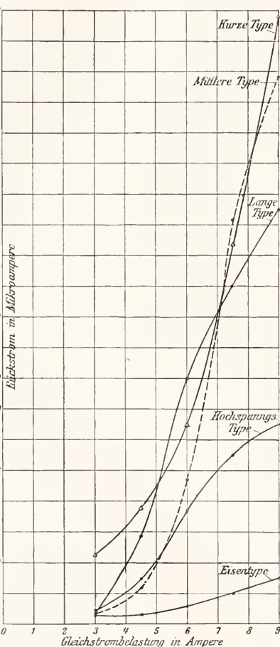
Fig. 14. Abhängigkeit des mittleren Rückstromes verschiedener Quecksilbergleichrichter für einphasigen Wechselstrom von der Gleichstrombelastung bei 240 V Wechselspannung zwischen den Anoden.
