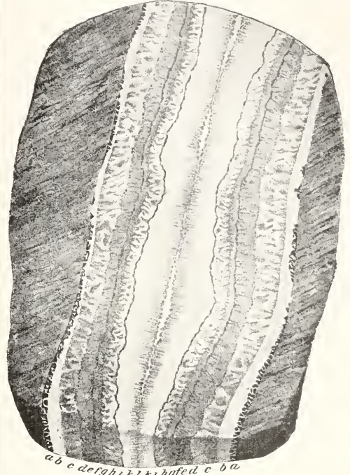
Fig. 6. Gangstufe der barytischen Bleifloration vom Prinzen-Spat der Grube Churprinz bei Freiberg. a Braune Blende, b weißer Quarz, c spargelgrüner Flußspat, d zarter Saum von brauner Blende, e schmutziggelber, krummschaliger Schwerspat, f schmaler Saum von Strahlkies, g Schwerspat = e, h Flußspat = c, i Strahlkies = f, k weißer Kalkspat, l lichtweingelber Kalkspat, in der Mitte kleine Drusen bildend. Nach v. Weißenbach.
