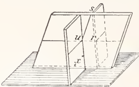
Fig. 2. Quer- verwerfung. x Sprungwinkel, u flache Sprung- höhe, ru Seiten- verschiebung.
