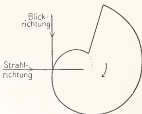
Fig. 17. Archimedische Spirale zur Sichtbarmachung von Oszillographenschwingungen.
