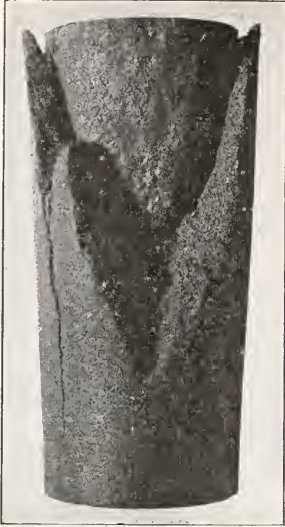
Fig. 10. Sandsteinkörper nach Druckversuch mit Kegelbildung.
