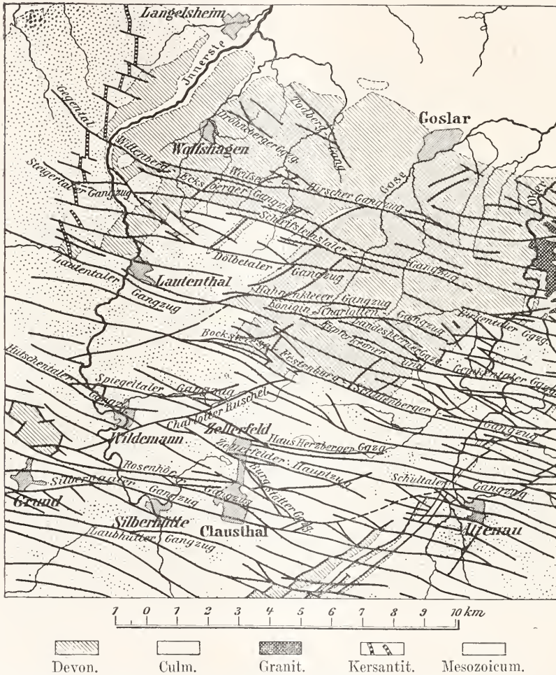
Fig. 5. Die Spalten, Erzgänge und Ueberschiebungen („Ruscheln“) im Oberharz. Nach Beushausen. Aus Stelzner-Bergeat, Erzlagerstätten.
