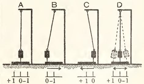
Fig. 11. Die Bewegungen eines Vertikalpendel-Seismometers während eines Erdbebens. A Ruhezustand. B und C während einer Bodenerschiebung in der Pfeilrichtung; die Masse bleibt stationär. D das Pendel ist in Eigenschwingungen geraten.
