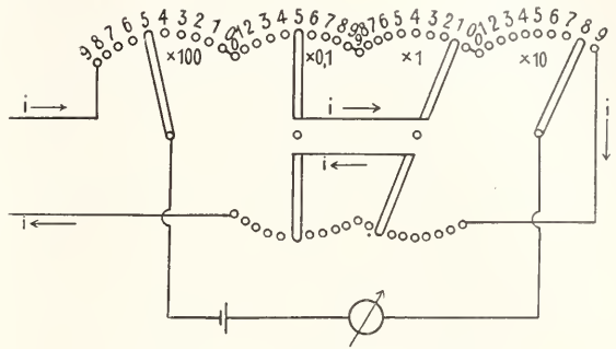
Fig. 2. Schema eines Kompensators nach Feußner.
