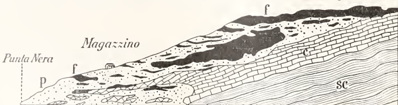
Fig. 14. Schematisches Profil durch die Eisensteinlagerstätten von Calamita auf Elba. sc Schiefer; c Kalkstein; p Pyroxen-Ilvait-Granatfels. f Magnetit. Nach Fabri und Lotti. Aus Stelzner-Bergeat, Erzlagerstätten.
