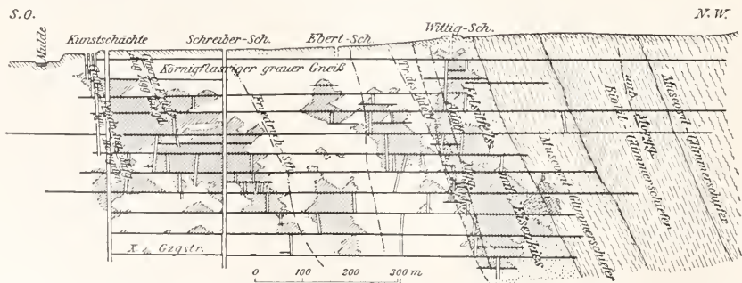
Fig. 7. Die Verteilung der Erzmittel im Ludwigspatgang zu Freiberg und ihre Abhängigkeit vom Nebengestein. Nach H. Müller. Aus Stelzner-Bergeat, Erzlagerstätten.
