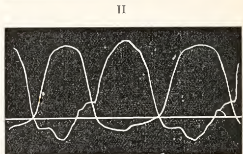
Fig. 21. Ventilwirkung von Aluminium in wässriger Lösung von Ammoniumborat. I Wechselspannung 90 Volt effektiv, II Wechselspannung 300 Volt effektiv. Ventil infolge von Ueberschreitung der Maximalspannung in der Sperrichtung teilweise durchlässig.
