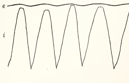
Fig. 17. Oszillogramme eines Drehstromquecksilbergleichrichters ohne Drosselspule im Gleichstromkreise. e Spannung, i Strom, I eines Zweiges (Ventiles), II des Gleichstromverbrauchskörpers (Glühlampen), III des Gleichstromverbrauchskörpers (Akkumulatoren-batterie).
