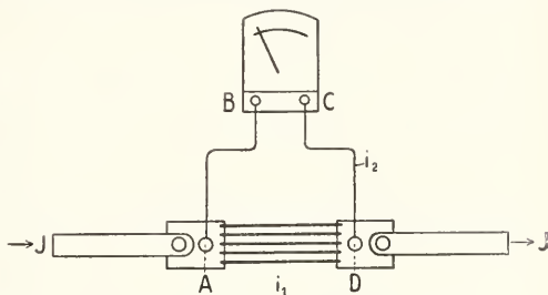
Fig. 1. Prinzip der Stromverzweigung.
