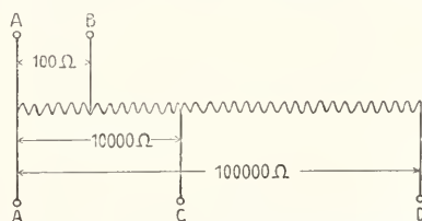
Fig. 5. Schema eines Spannungsteilers.
