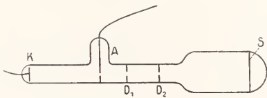
Fig. 14. Braunsche Röhre.
