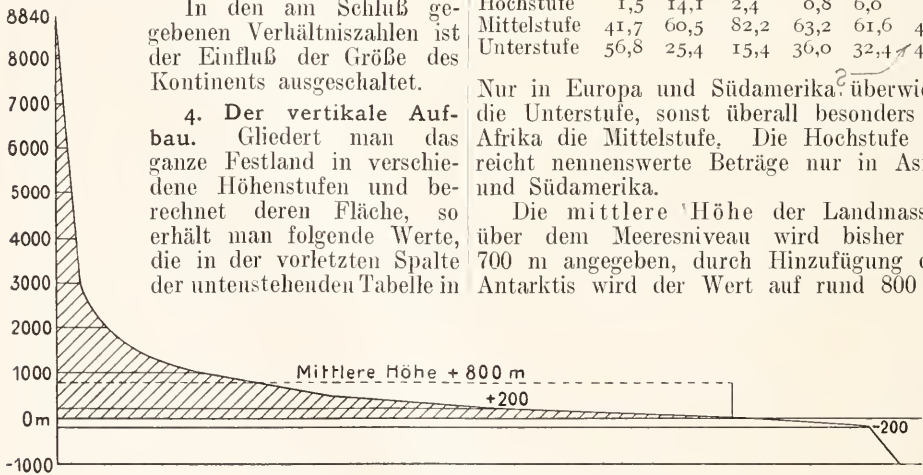
Hypsographische Kurve des festen Landes.
