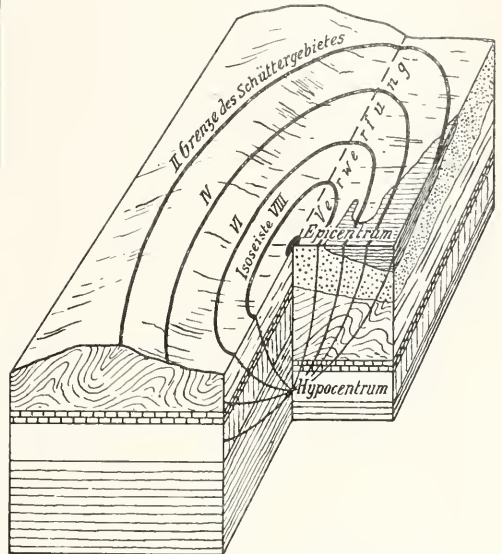
Fig. 1. Modell zur Veranschaulichung der wichtigsten seismologischen Begriffe.
