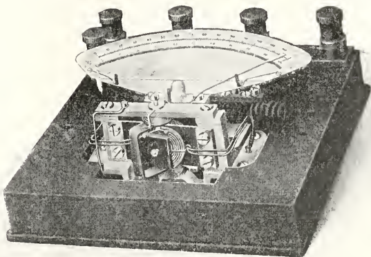
Fig. 8. Dynamometrischer Strommesser.
