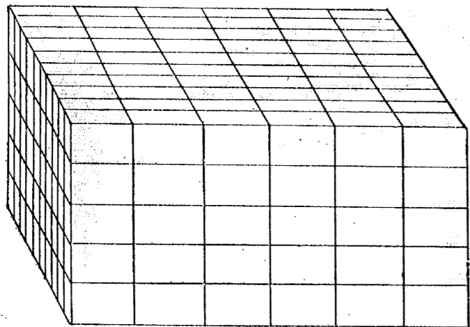
第貳圖 長壽煙九拾五瓦入木箱詰方法
