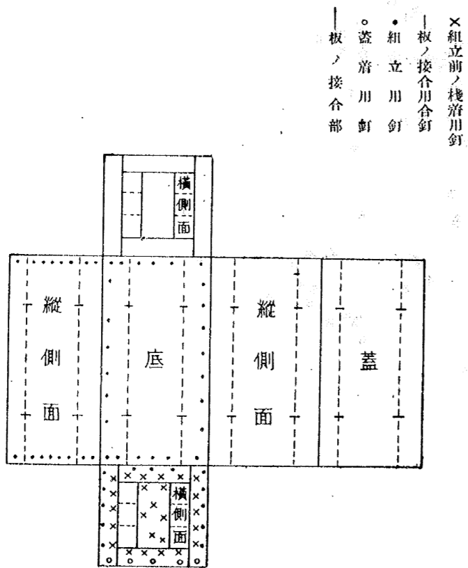
朝日釘打仕罫圖
