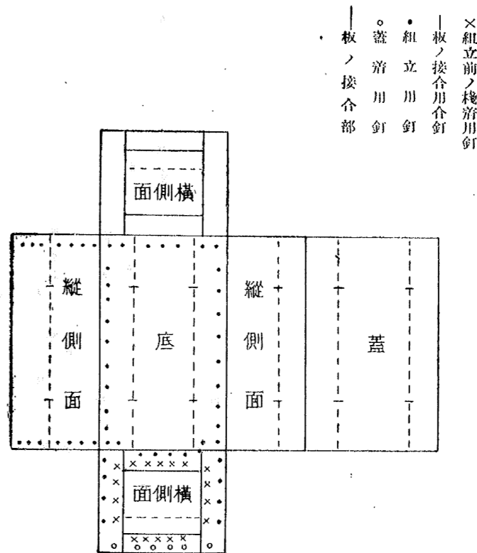
敷島、松風釘打仕罫圖
