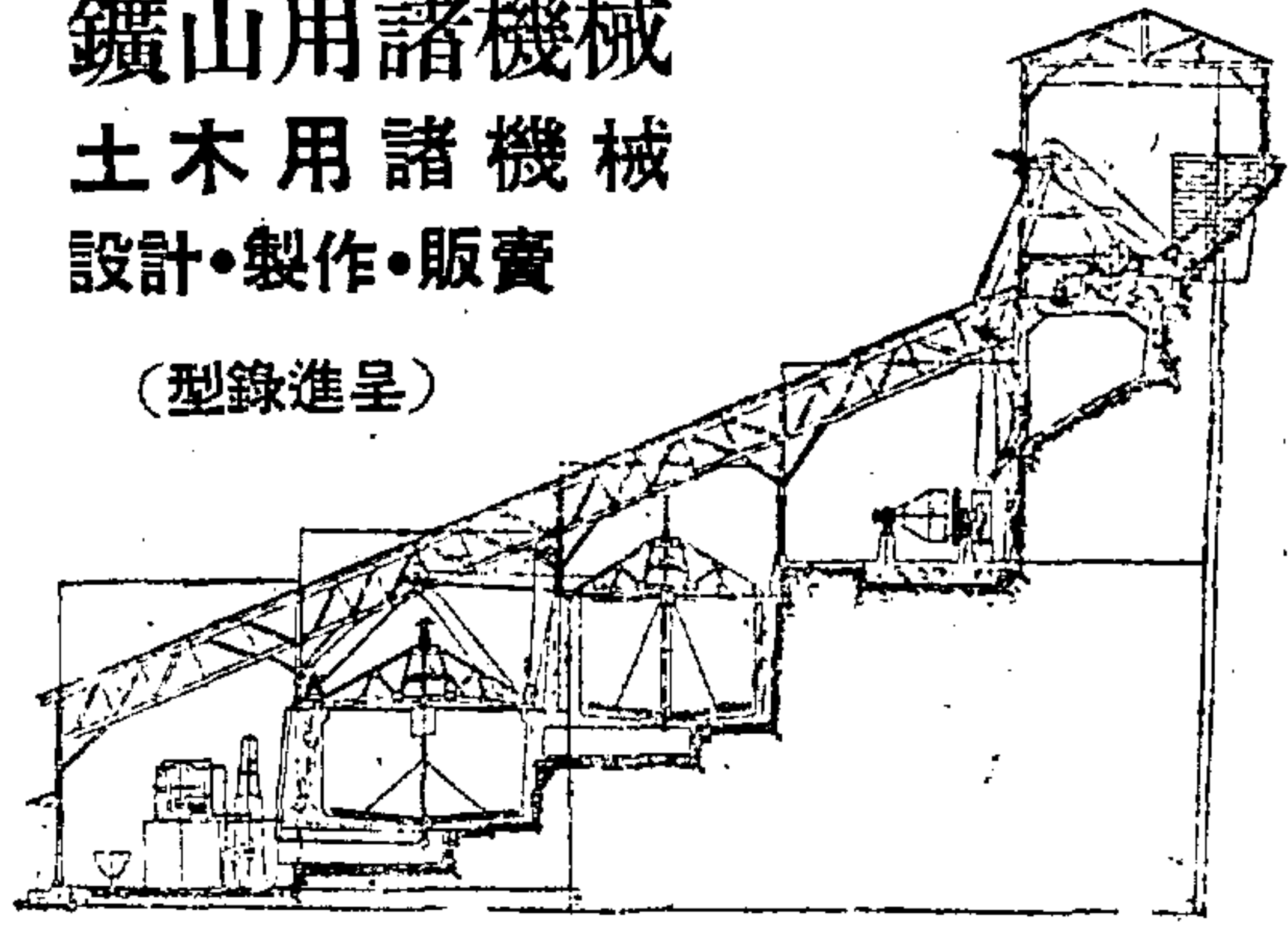
製鍊所断面圖
