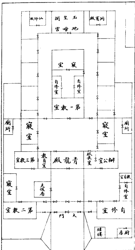
圖舍校校學小等高秋誦立私
