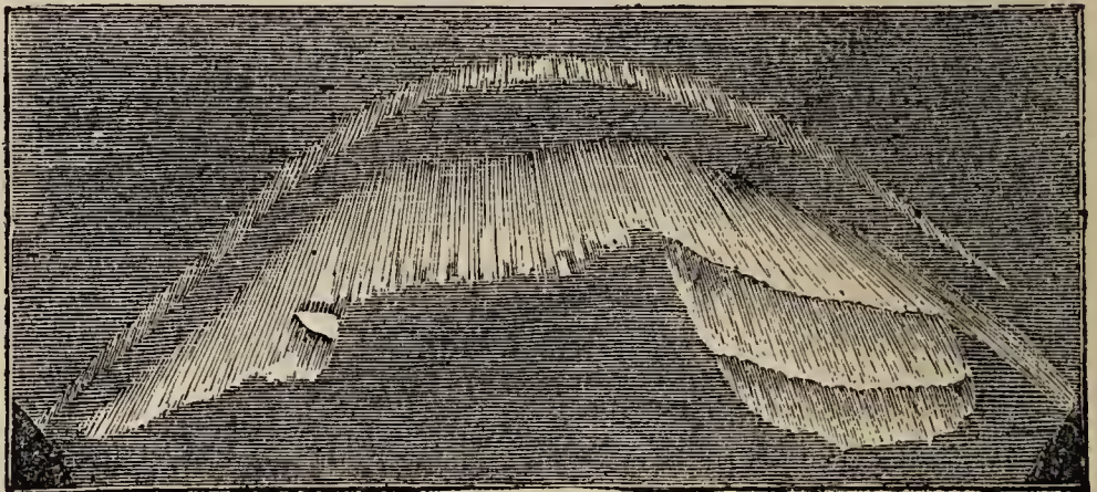
Aurora Borealis.
