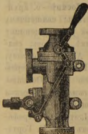
Универс. Инжекторъ.
