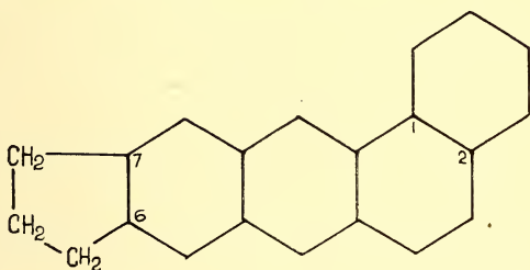
6:7-cyclopenteno-1:2-benzanthracene.
