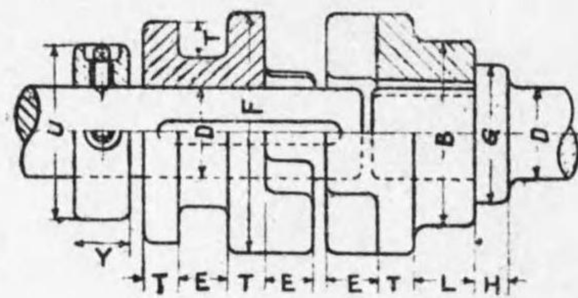
第 3-62 圖 咬合接手
