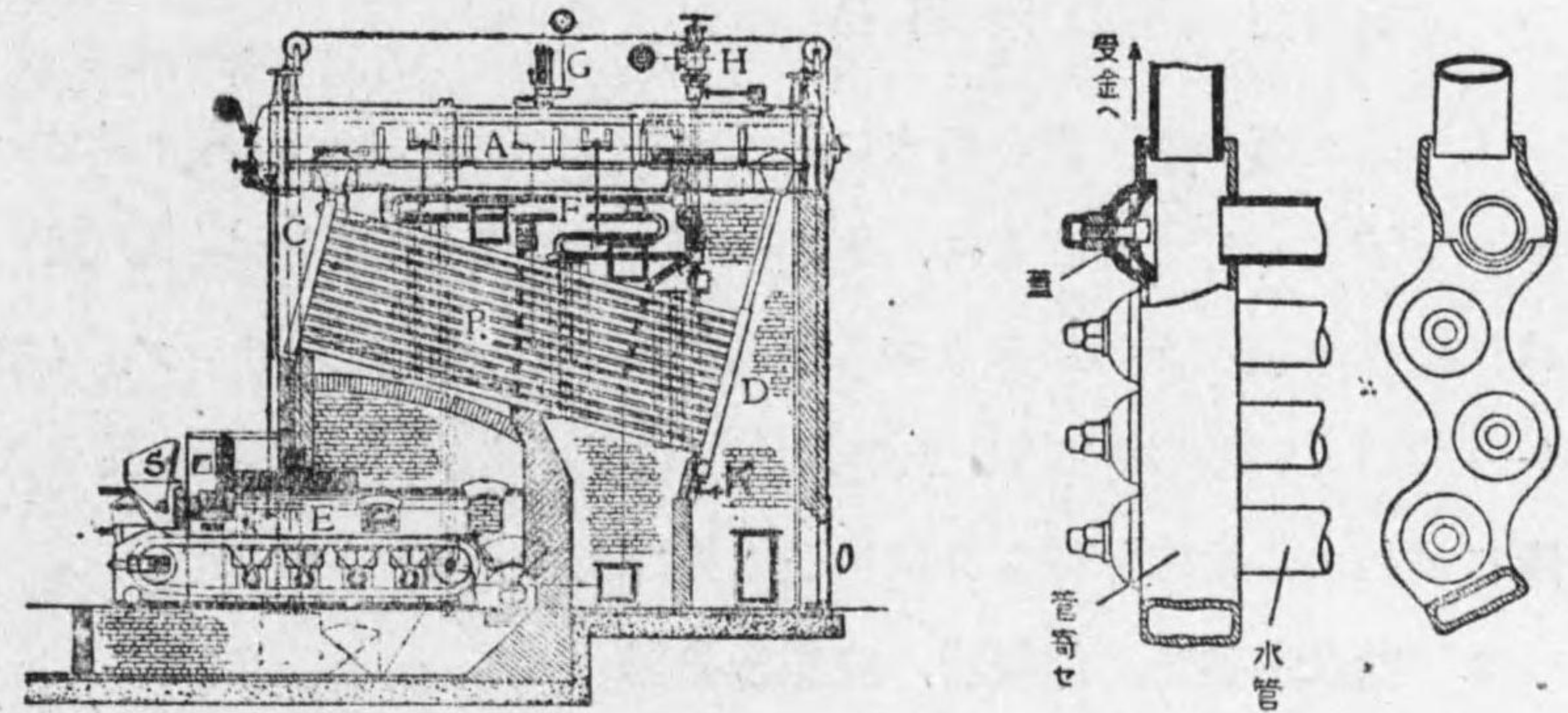
第5-10圖 バブコック・ウイルクソックス罐
