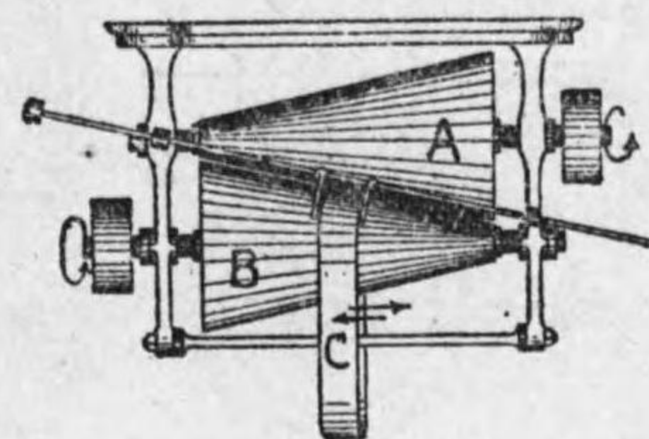
第 3-22 圖 イーバンス圓錐摩擦
