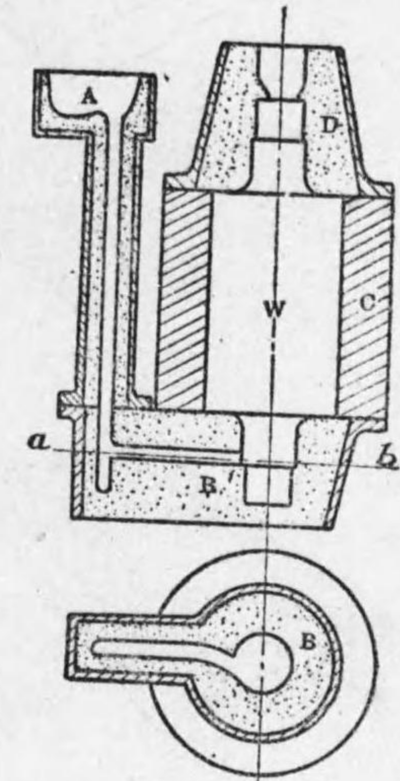
第10-12圖 チル鑄型
