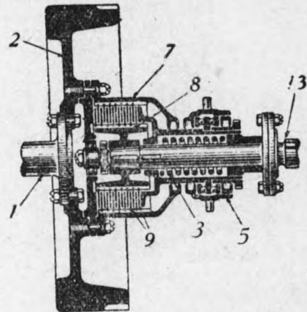
第 8-80 圖 多盤式クラッチ
