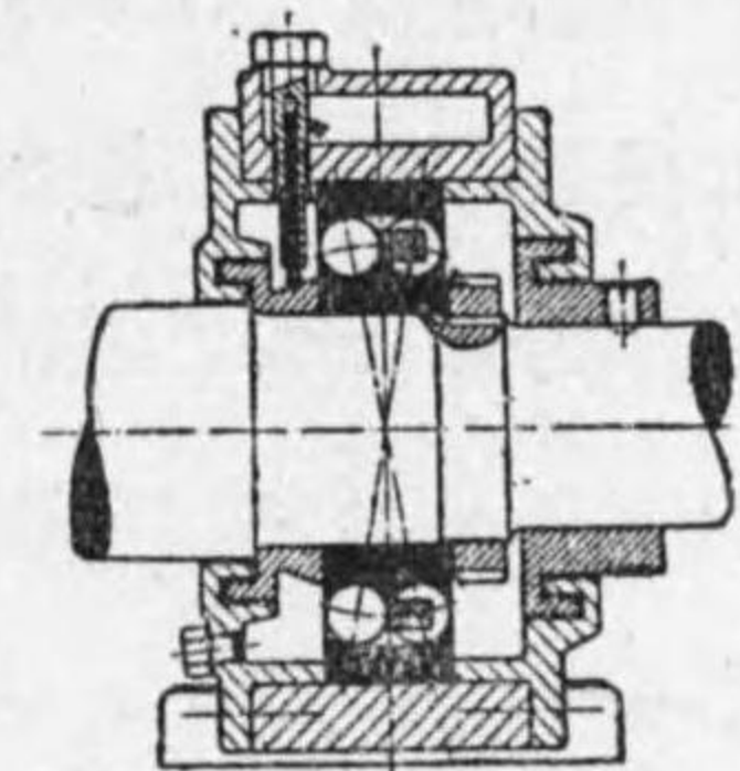
第3-14圖 球入軸承
