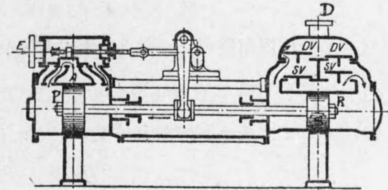
第 4-30 圖 ウオシントンポンプ
