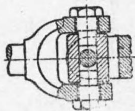
第3-9圖 自在接手
