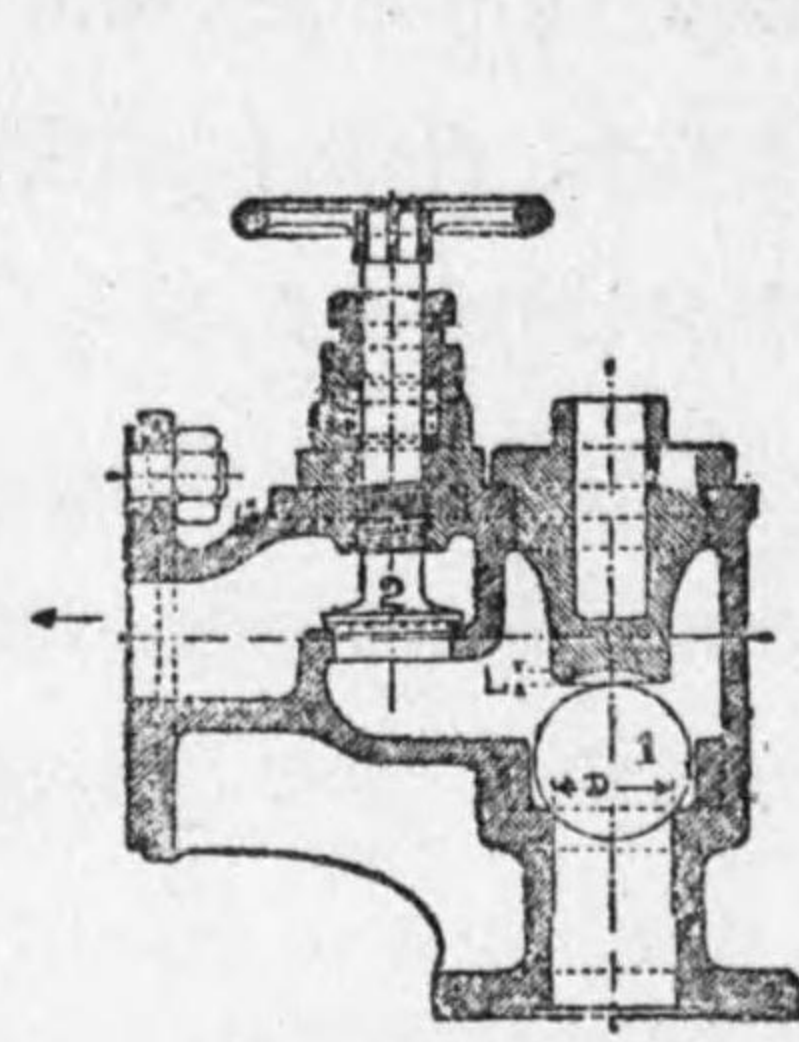
給水逆止弁 第 5-14 圖
