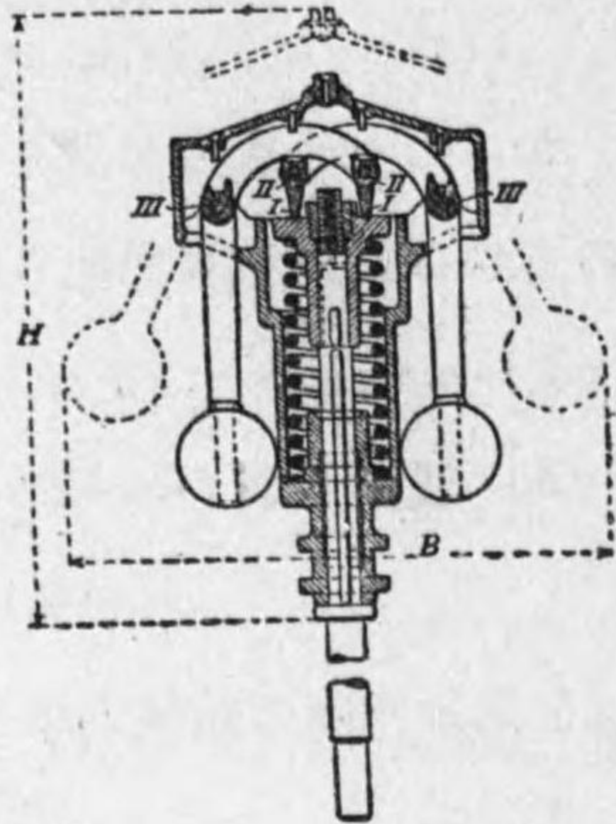
第 6—8 圖 トレンク調速機
