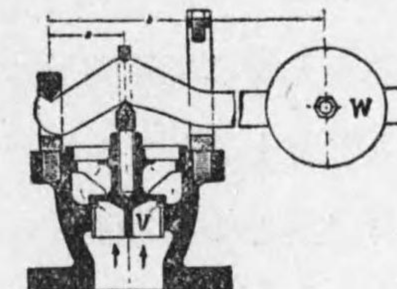
第 5-20 圖 挺子安全弁
