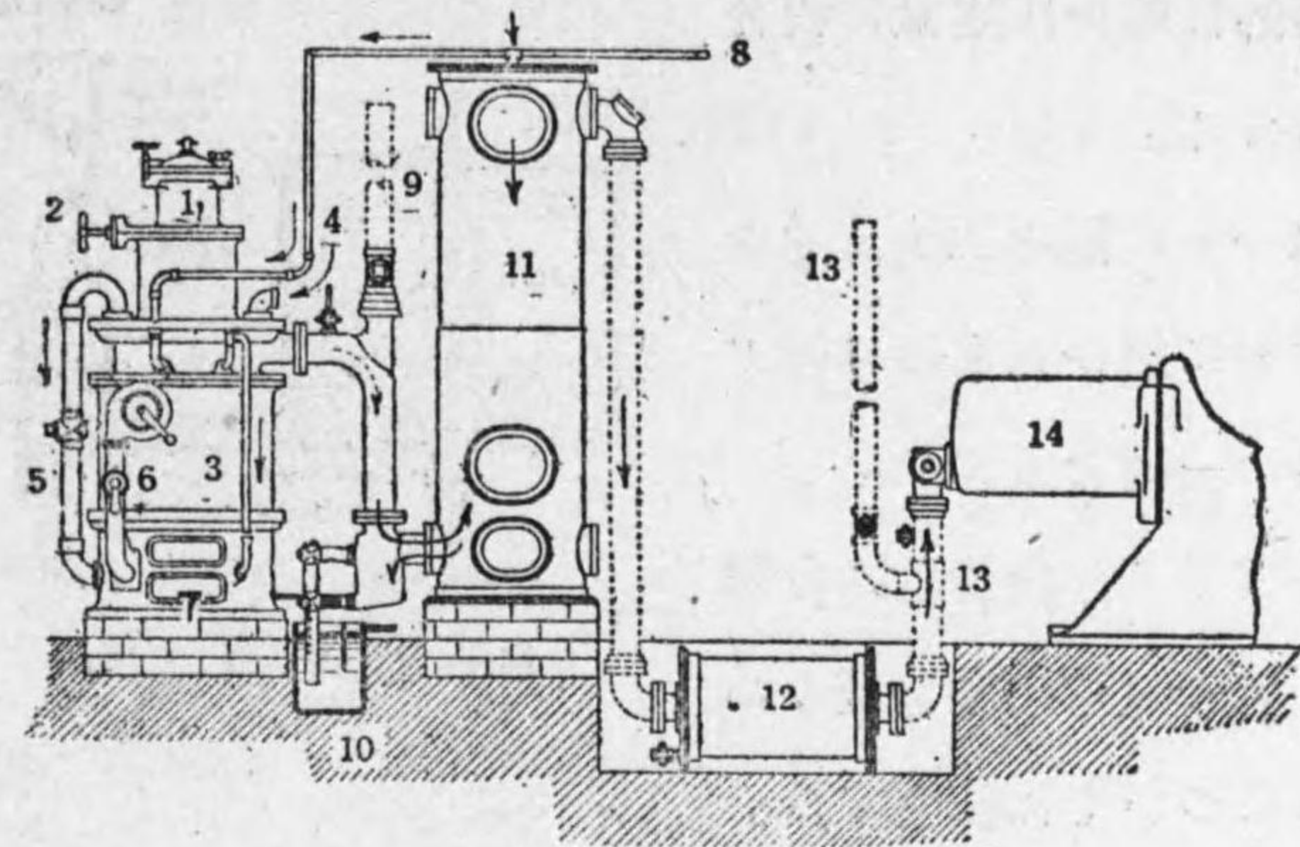
第8—18圖 吸込式發生爐
