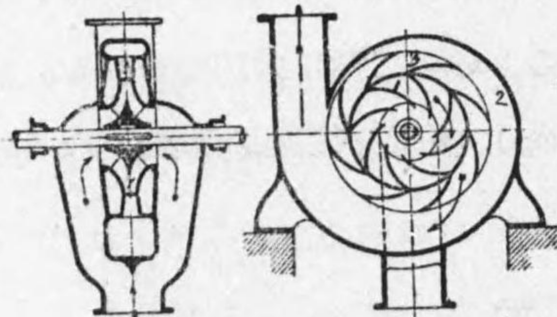
第 4-23 圖 一段タービンポンプ
