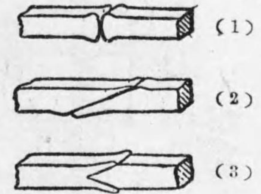
第 10-31 圖 鍛接法
