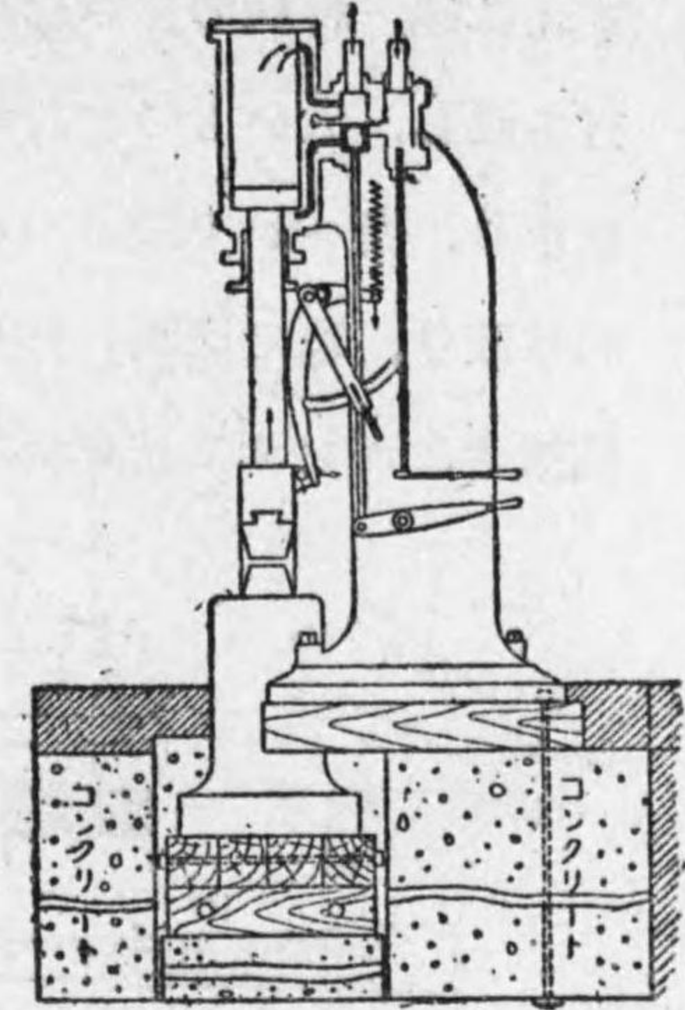
第 10-26 圖 蒸汽錘
