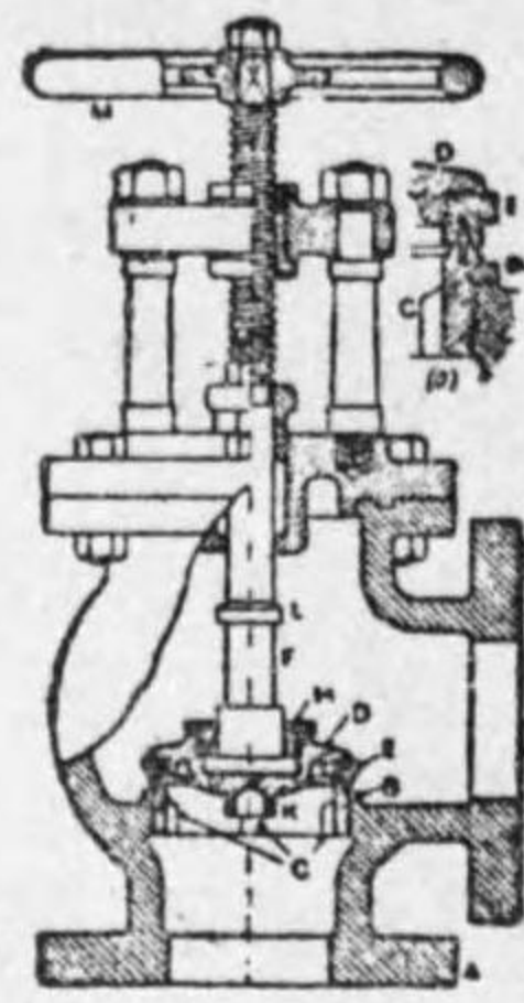
止め弁(球型) 第5-22圖
