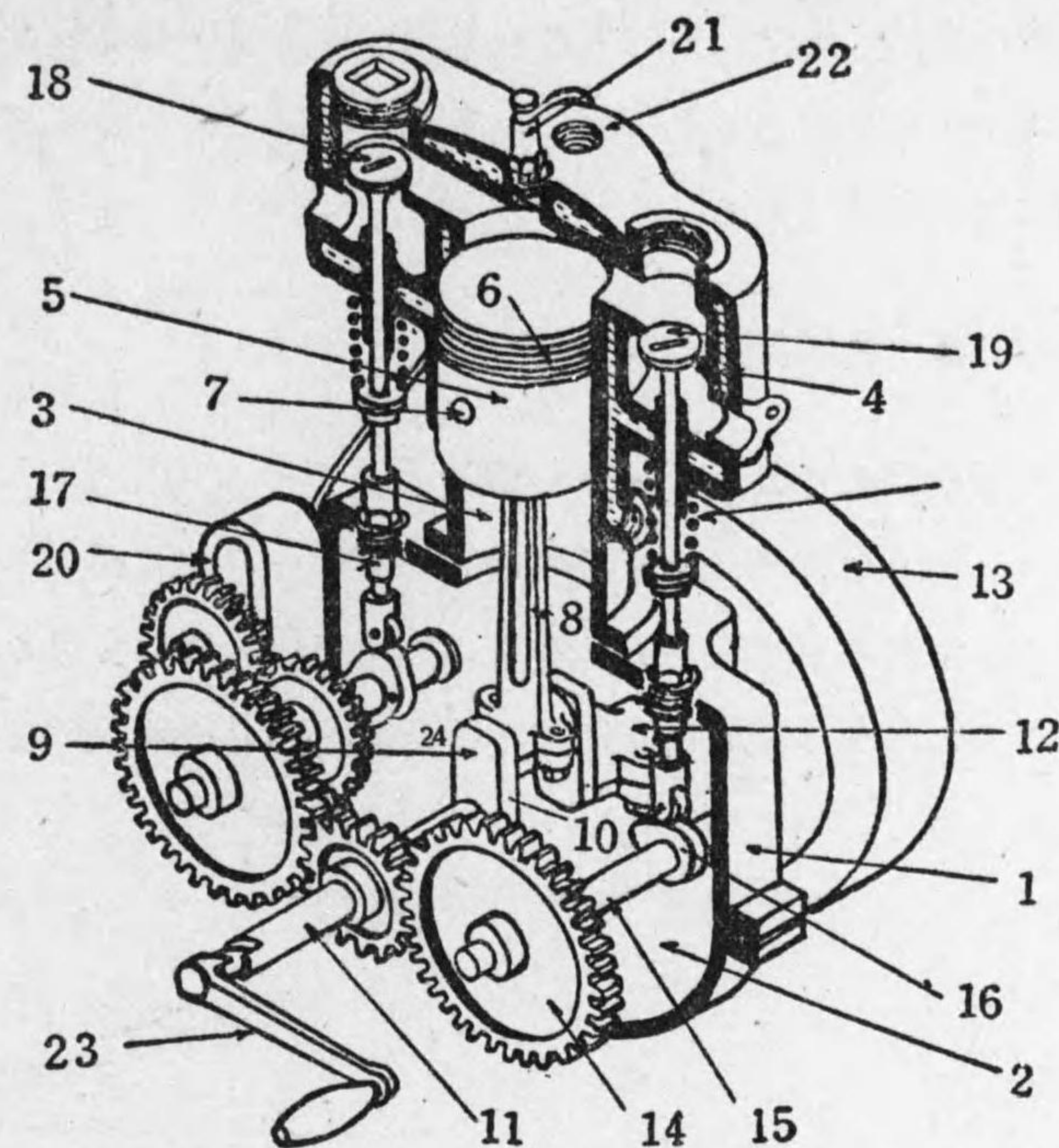
第 8-3 圖 ガソリン機關構造圖
