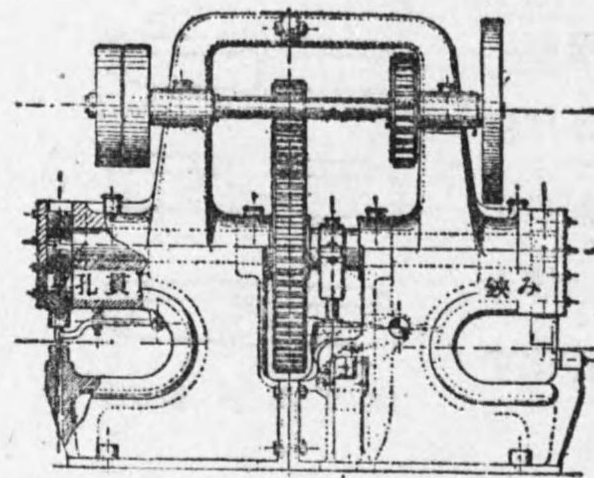
第 10-32 圖 鋏み孔貫盤
