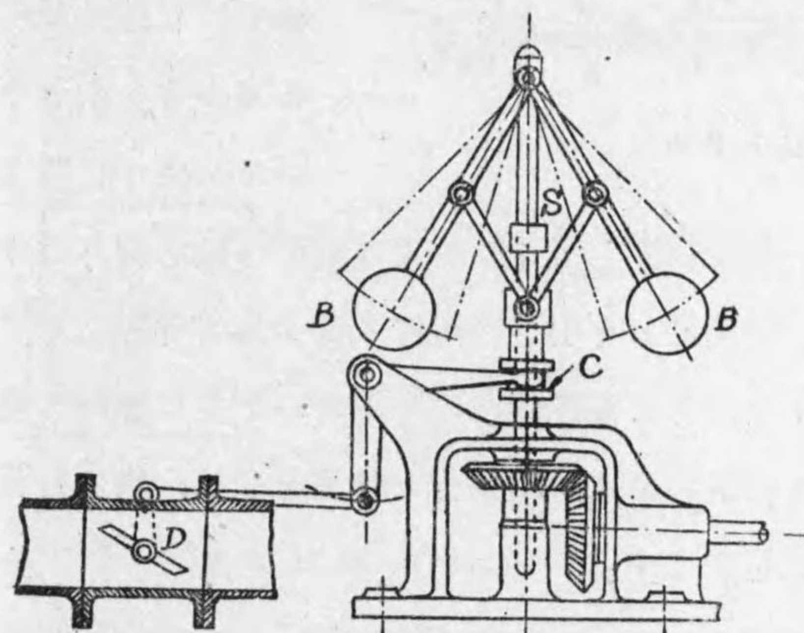
第 6-7 圖 ワット式調速機
