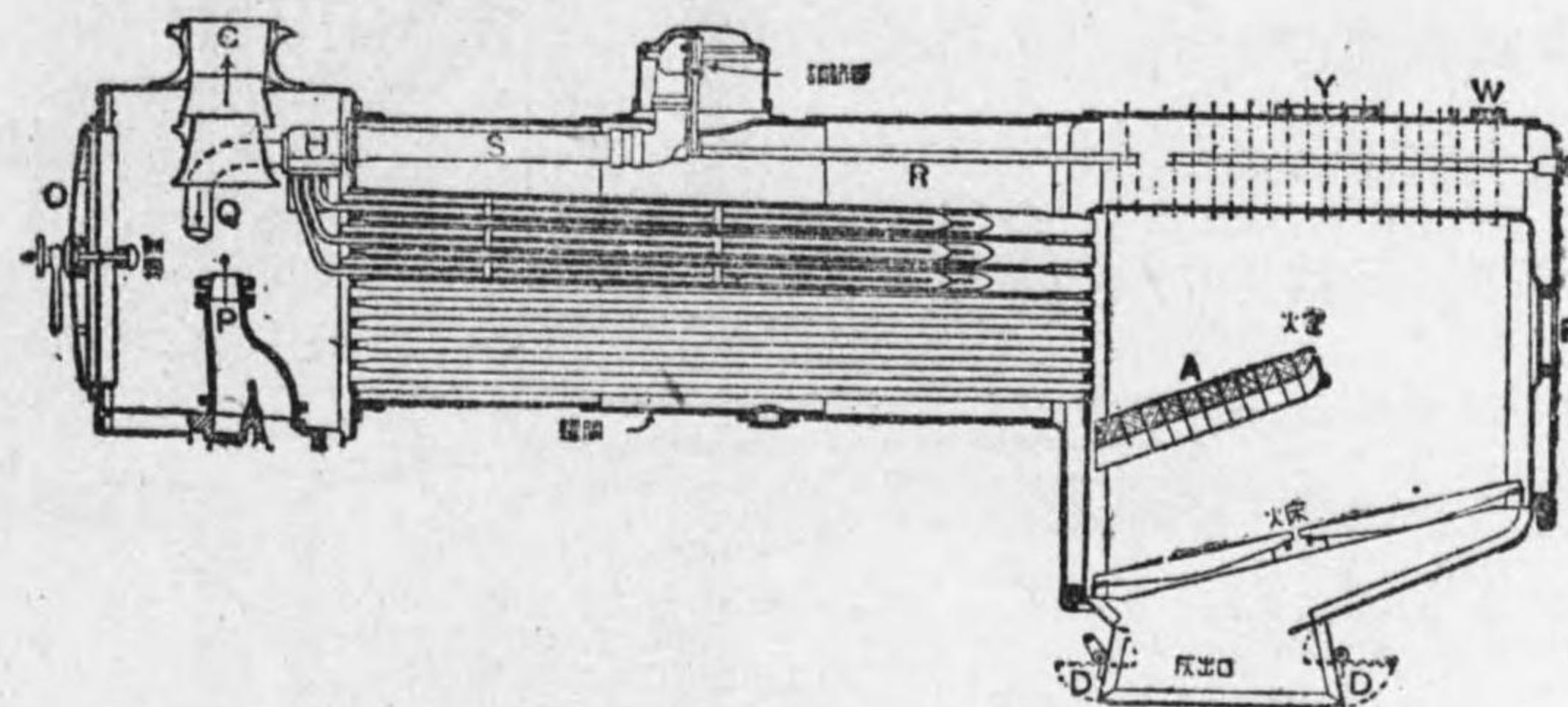
第 5-7 圖 汽 車 鍋
