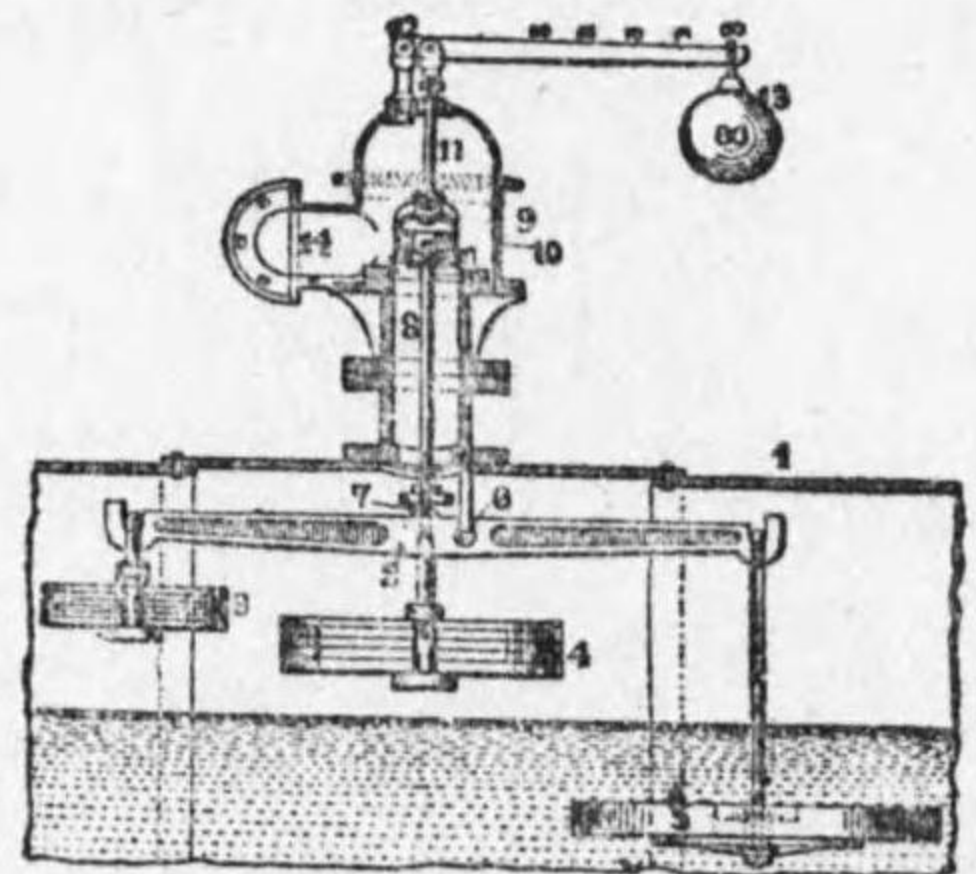
第 5-17 圖 低水報知器
