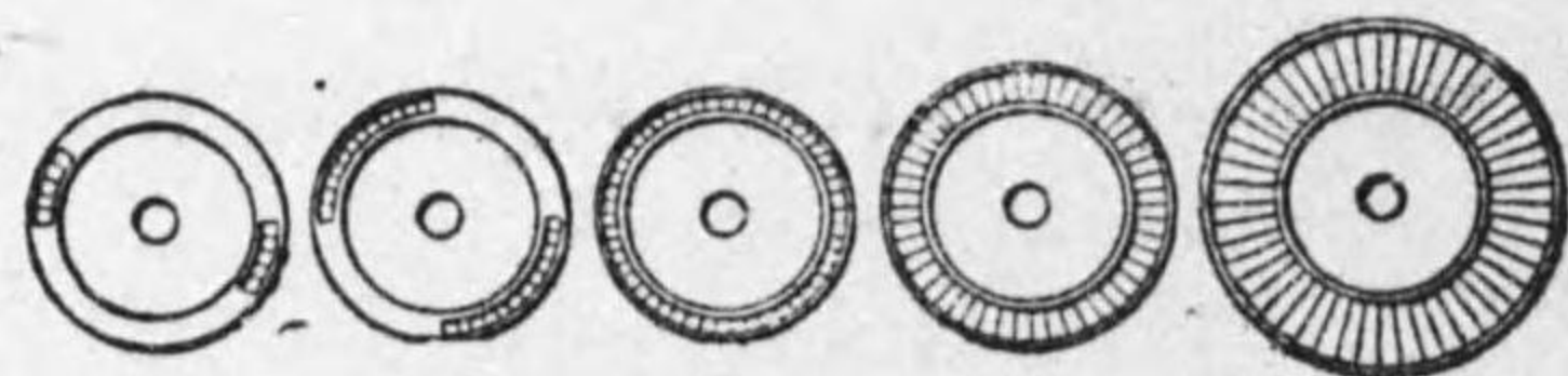
第7-15圖 隔 板
