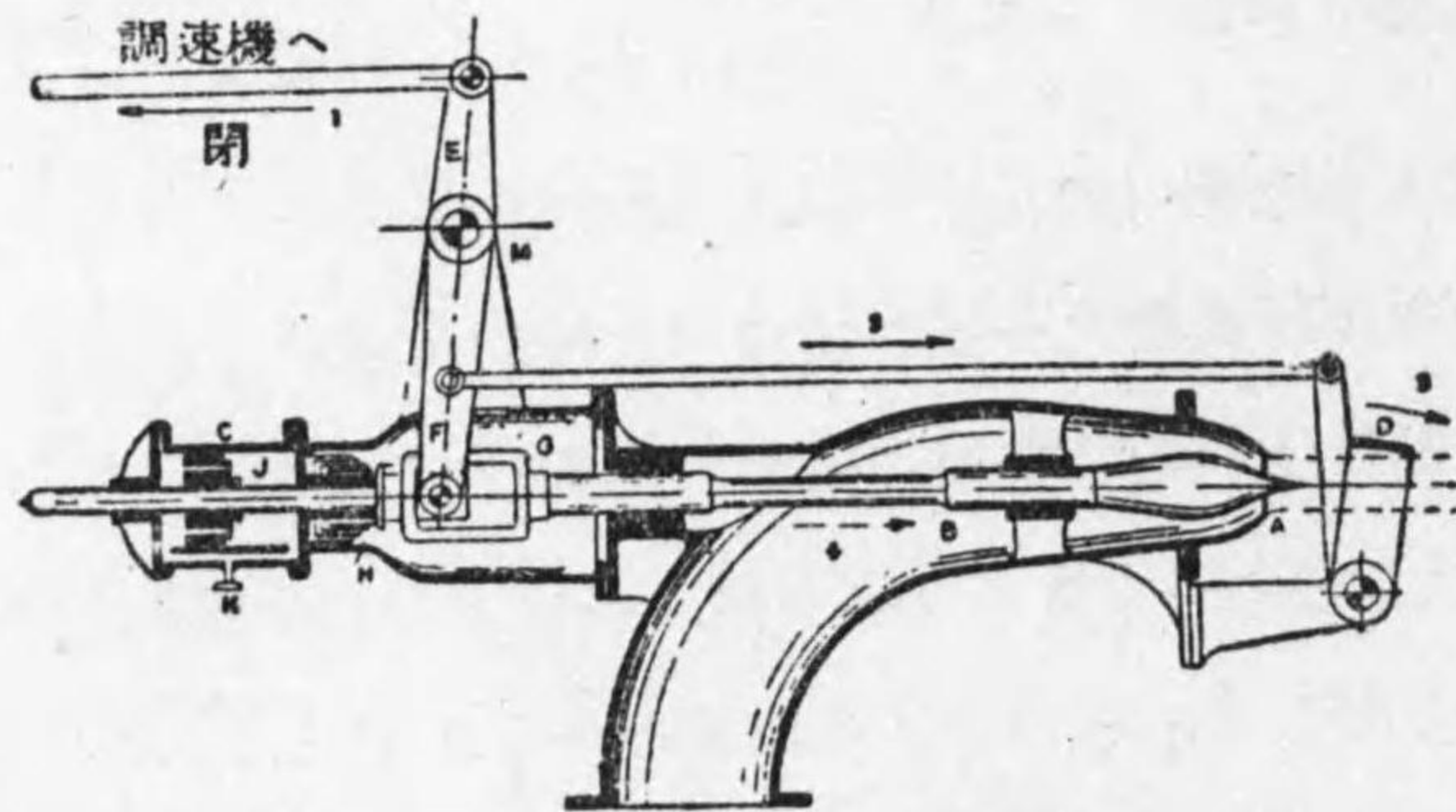
第 4-7 圖 そらせ板調速装置
