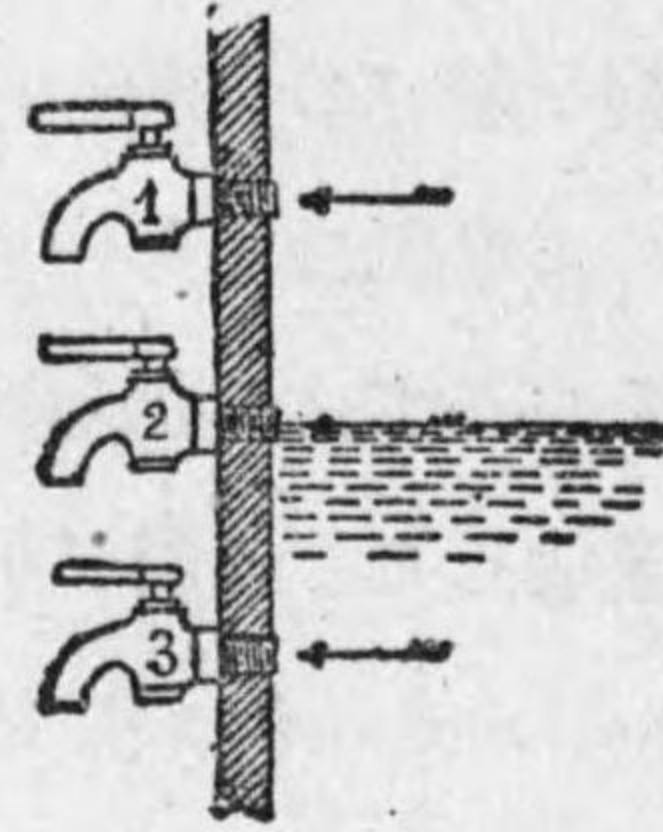
第 5-16 圖 験しコック
