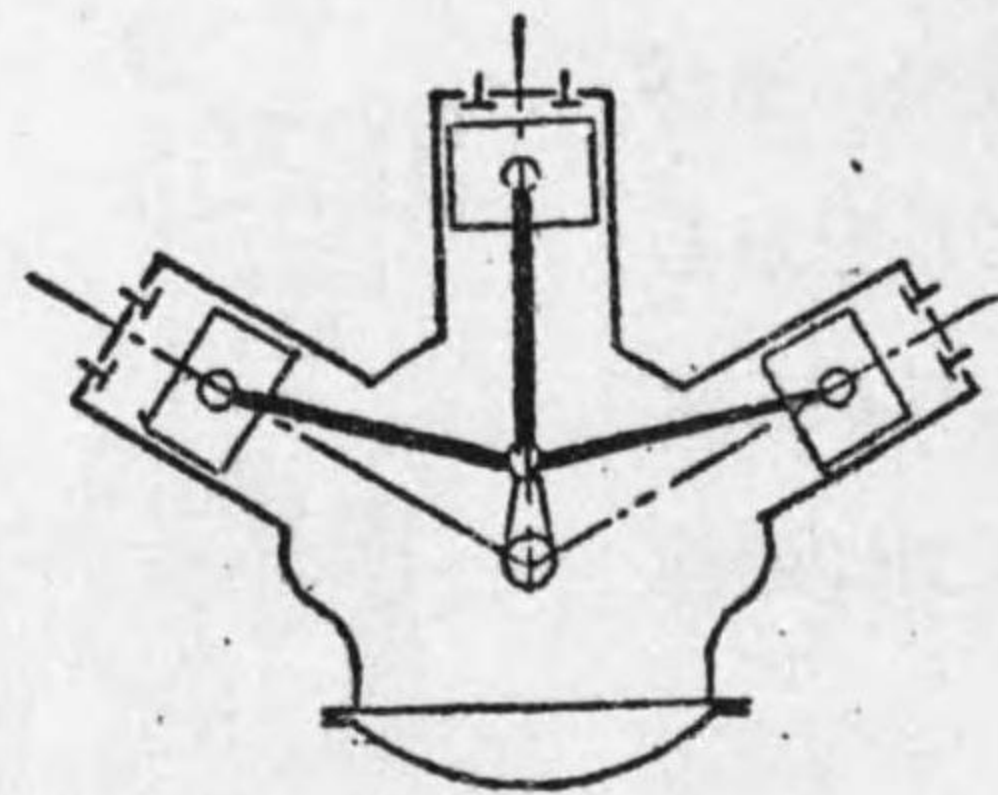
第 8—33 圖 W型機關
