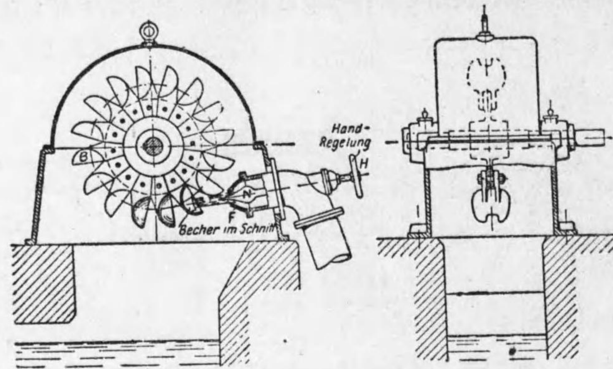
第 4-6 圖 ペルトン水車
