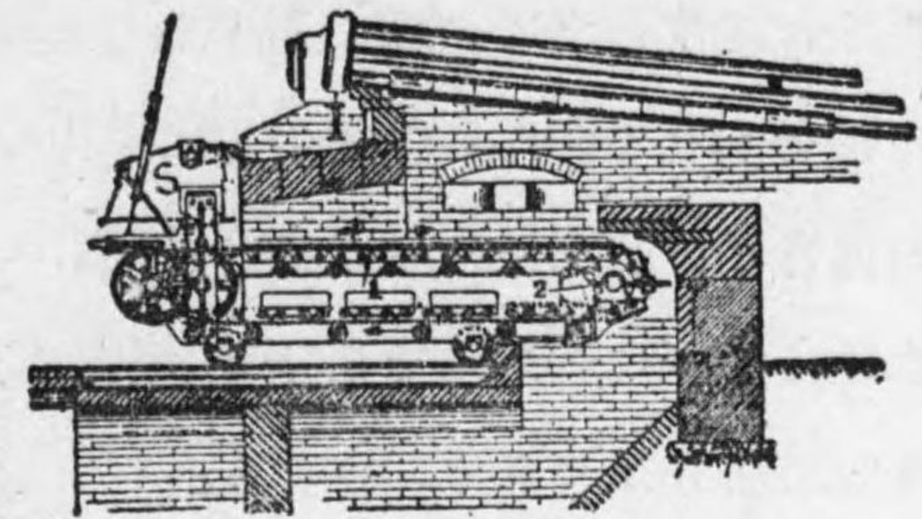
第5-26圖 鎖火格子ストーカー
