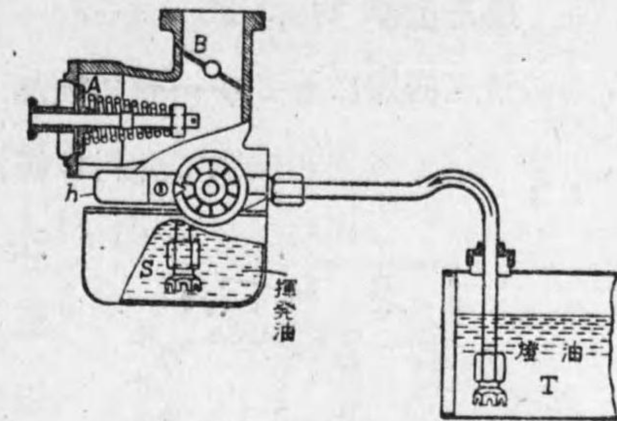
第 8-21 圖 石油機関混和器
