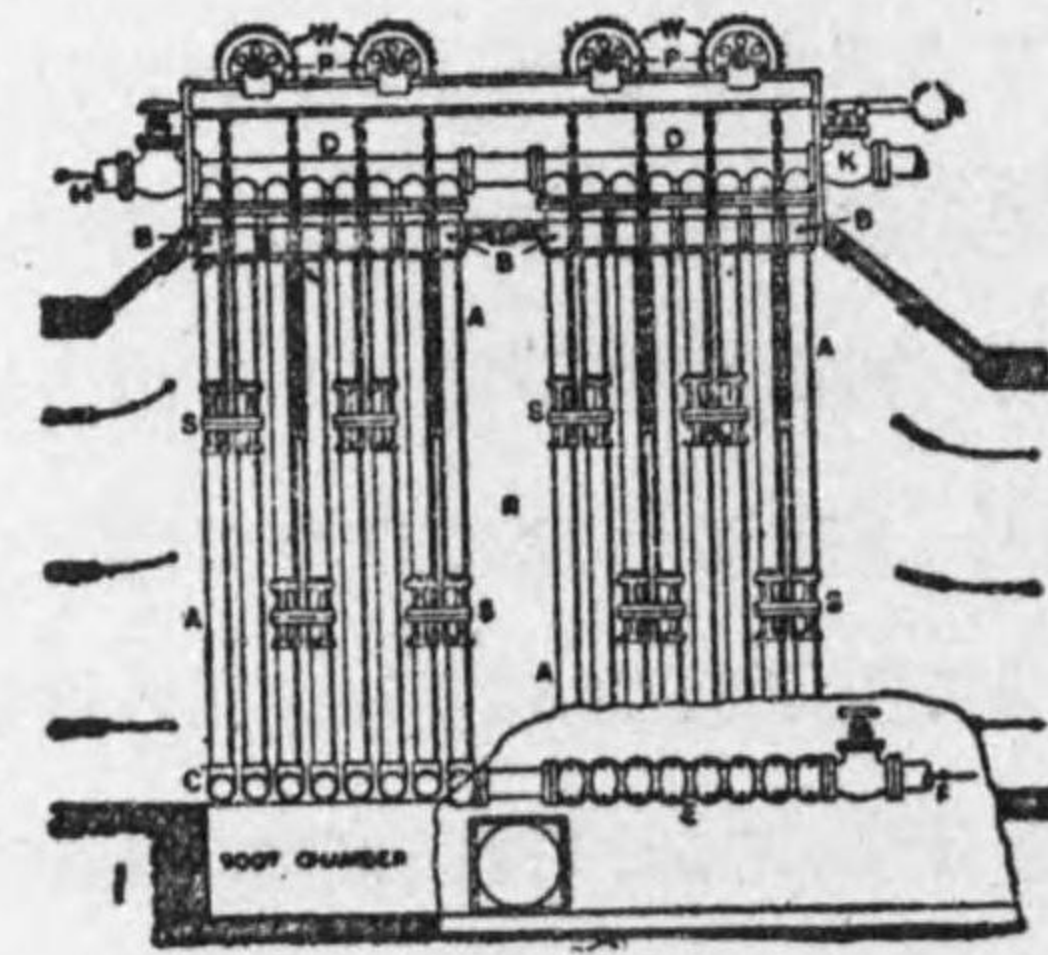
第5—12圖 節炭器
