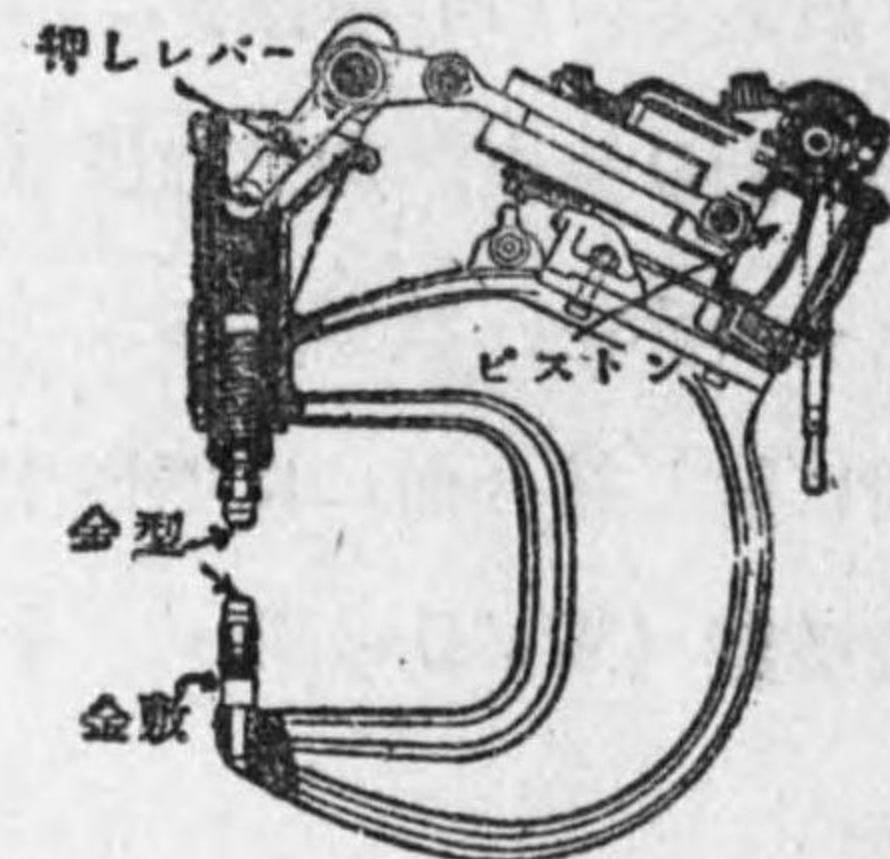
第 10-33 圖 空気鋸締機
