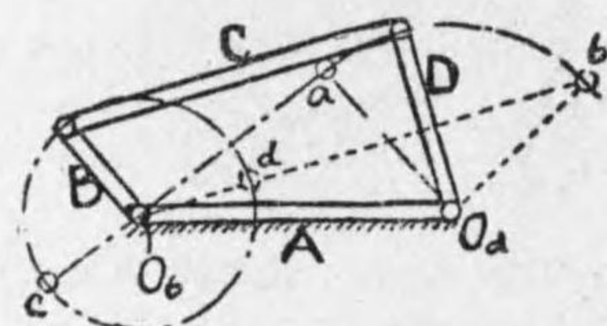
第3-53圖 四つ棒リンク仕掛
