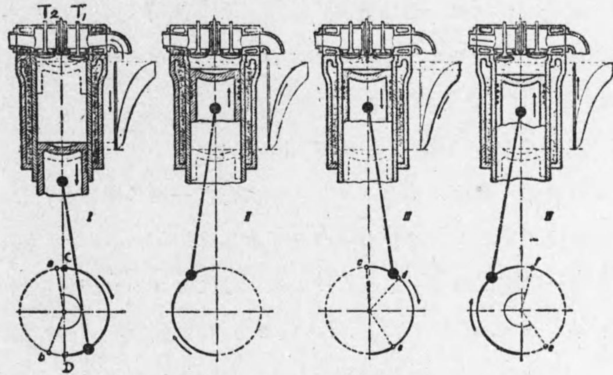
第8-1圖 四サイクル機關
