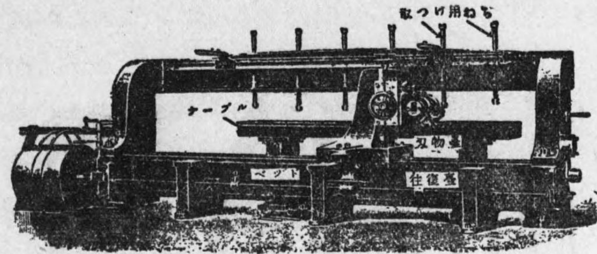
第 10-35 圖 耳 削 盤
