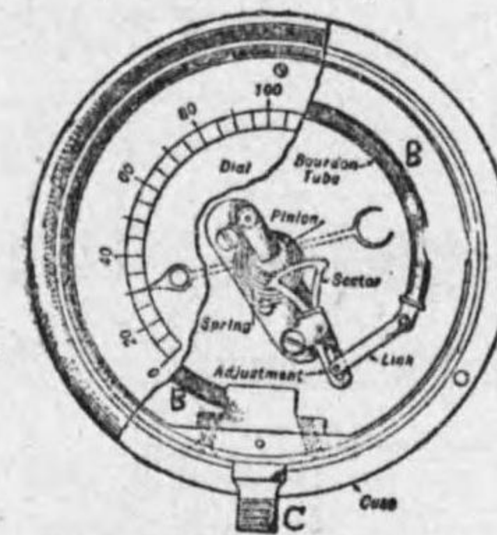
第 5-19 圖 壓力計
