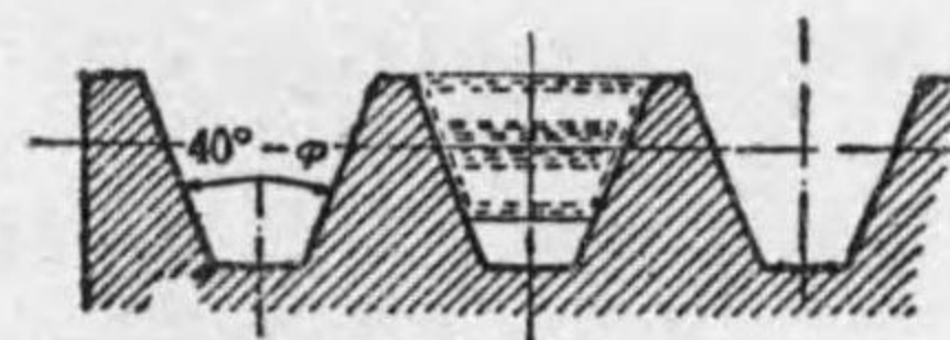
第 3-43 圖 Vベルト溝車
