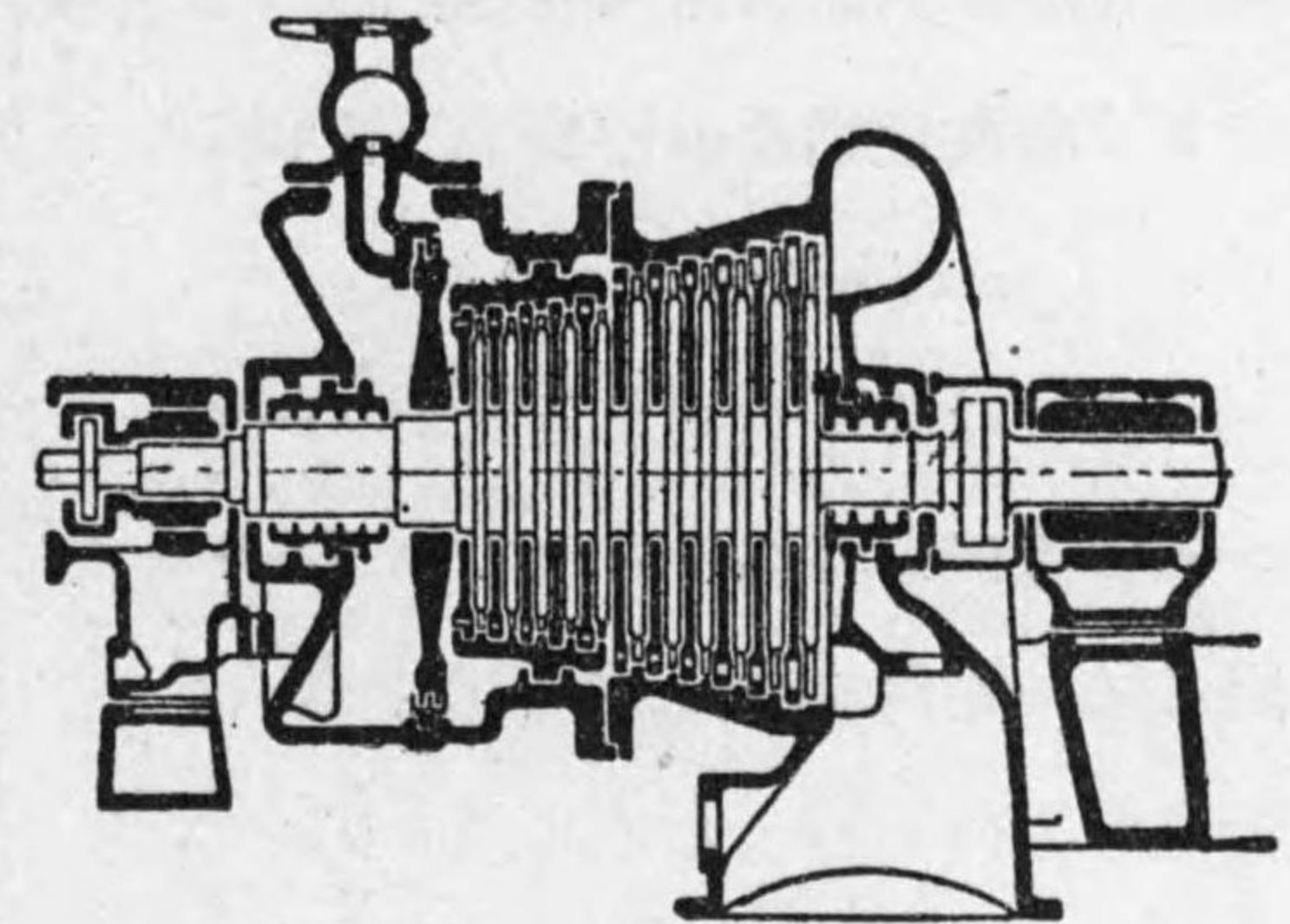
第 7-6 圖 多速多壓段組合せタービン
