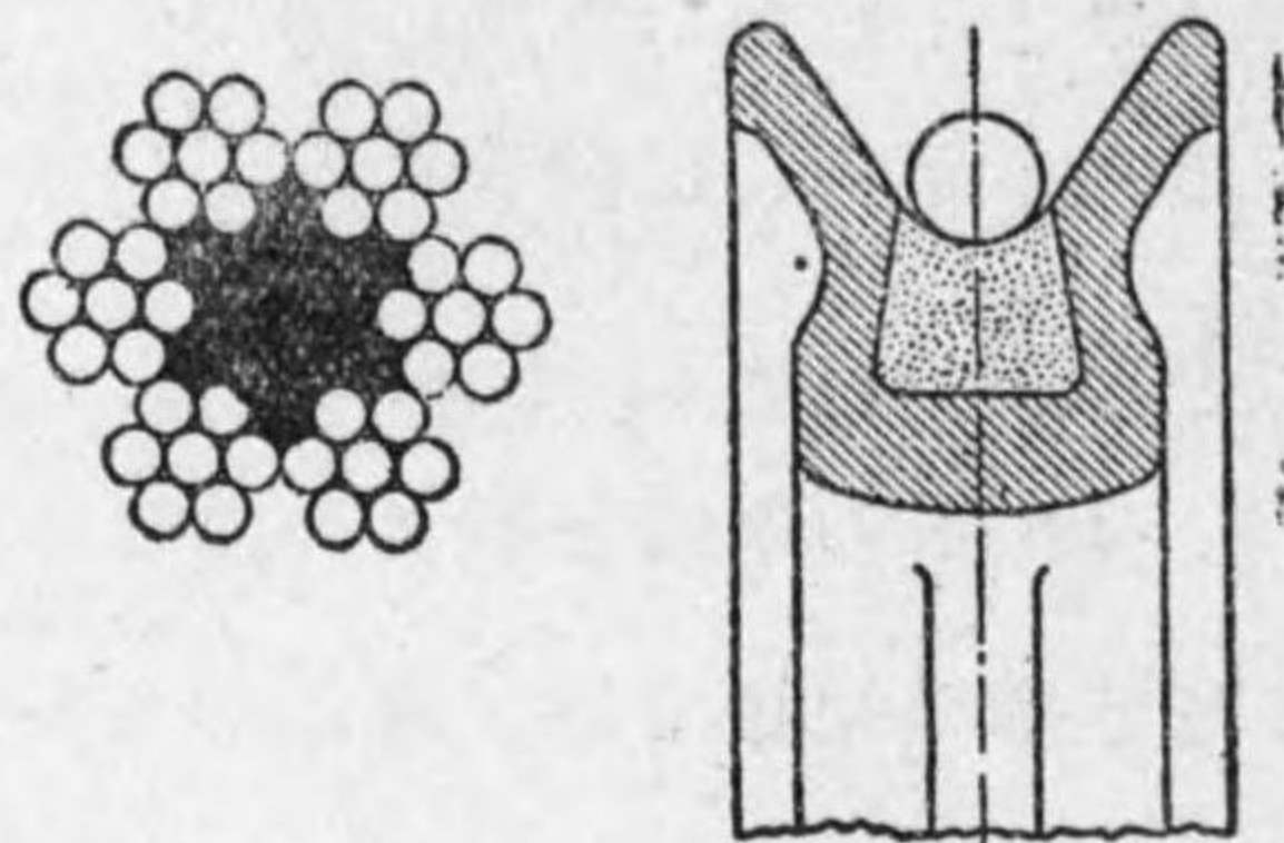
第 3-45 圖 鋼索と鋼索車
