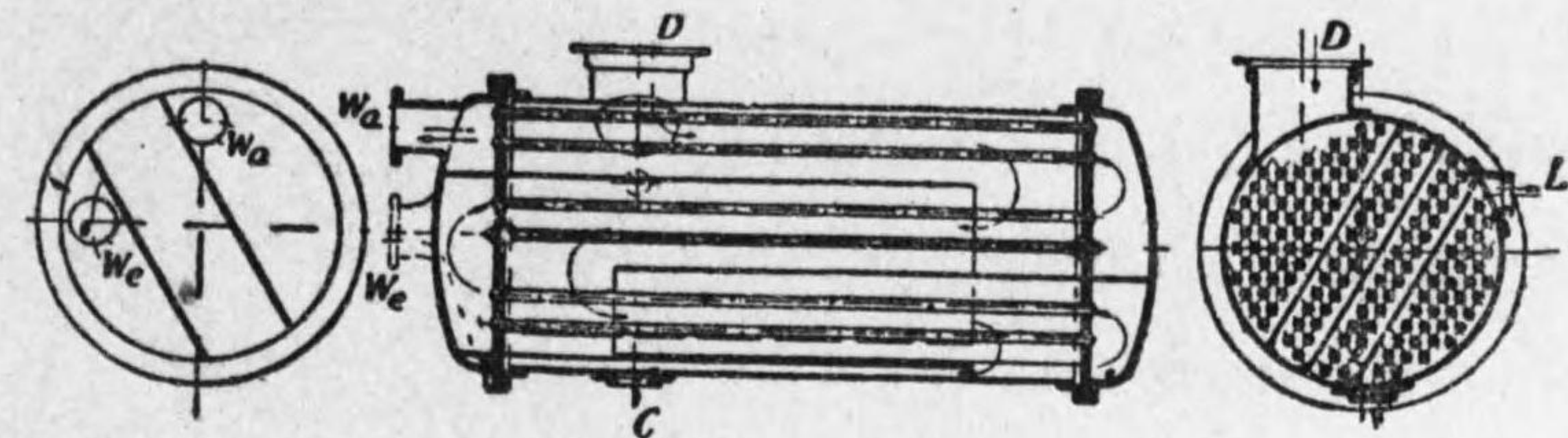
第 7-22 圖 表面凝結器
