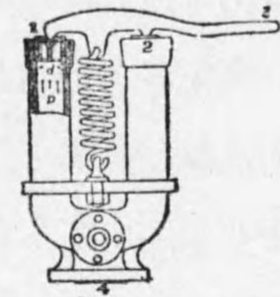
ばね安全弁(張力型) 第 5-21 圖
