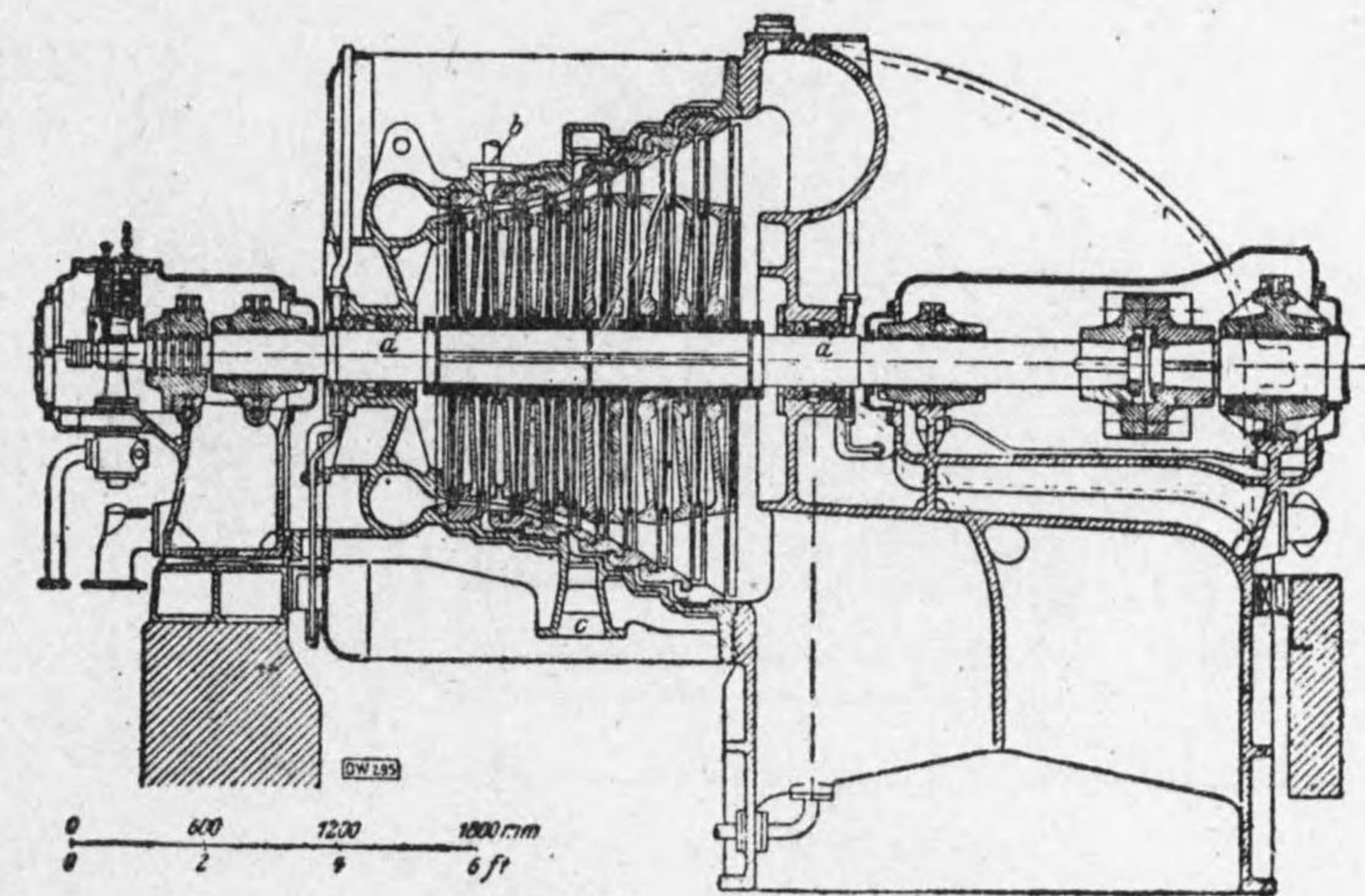
第 7-19 圖 ツエリタービン
