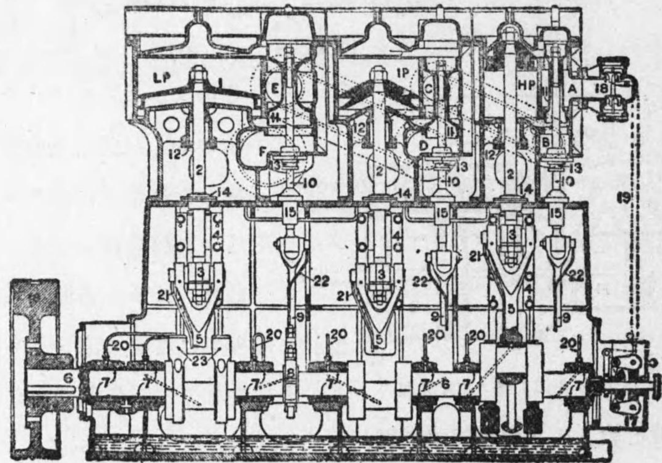
第 6-14 圖 三 段 膨 脹 機 關
