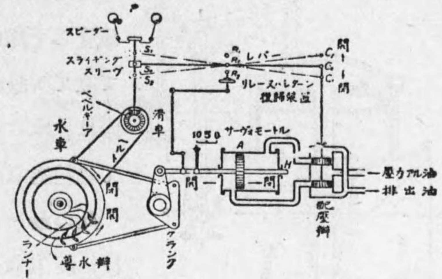
第 4-18 圖 調速機の構造圖
