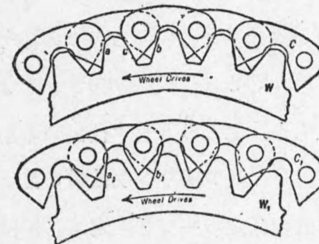
第 3-50 圖 無鎖
