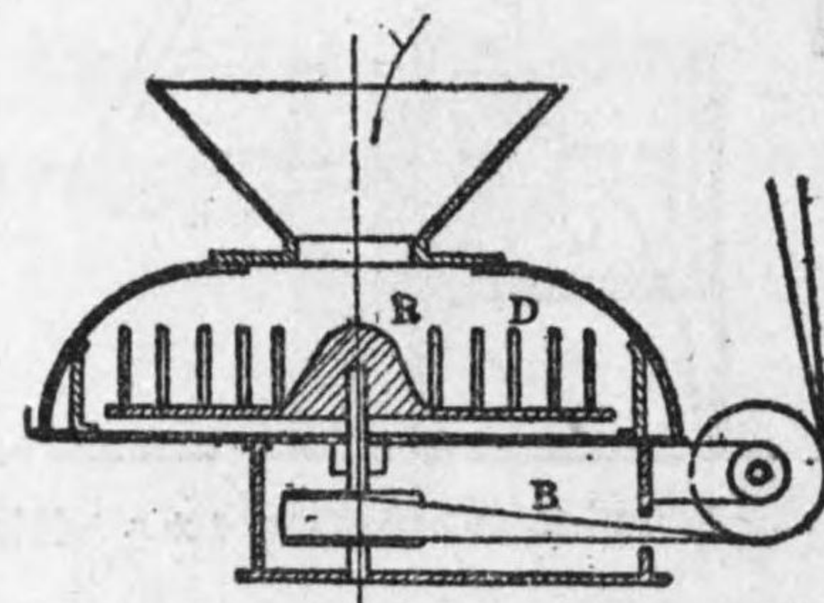
第 10-17 圖 砂 混 機
