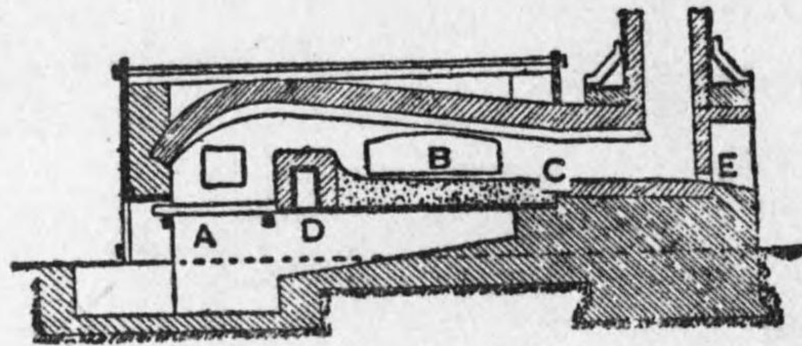
第 10-24 圖 反 射 爐
