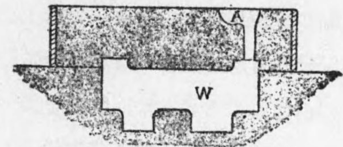
第10—10圖 床込め法
