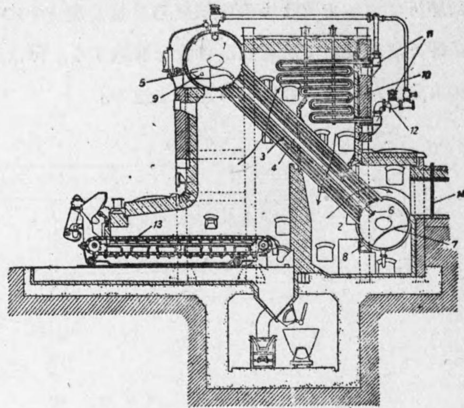
第5-9圖 タクマ罐
