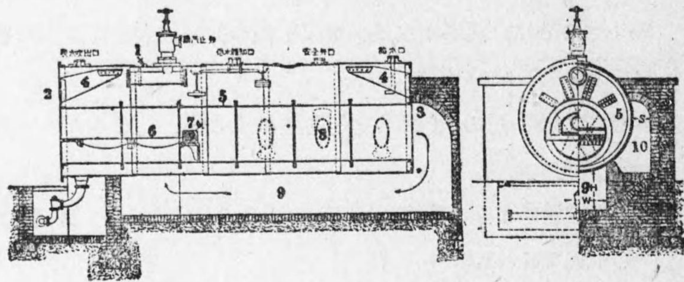
第 5-2 圖 コルニシ罐
