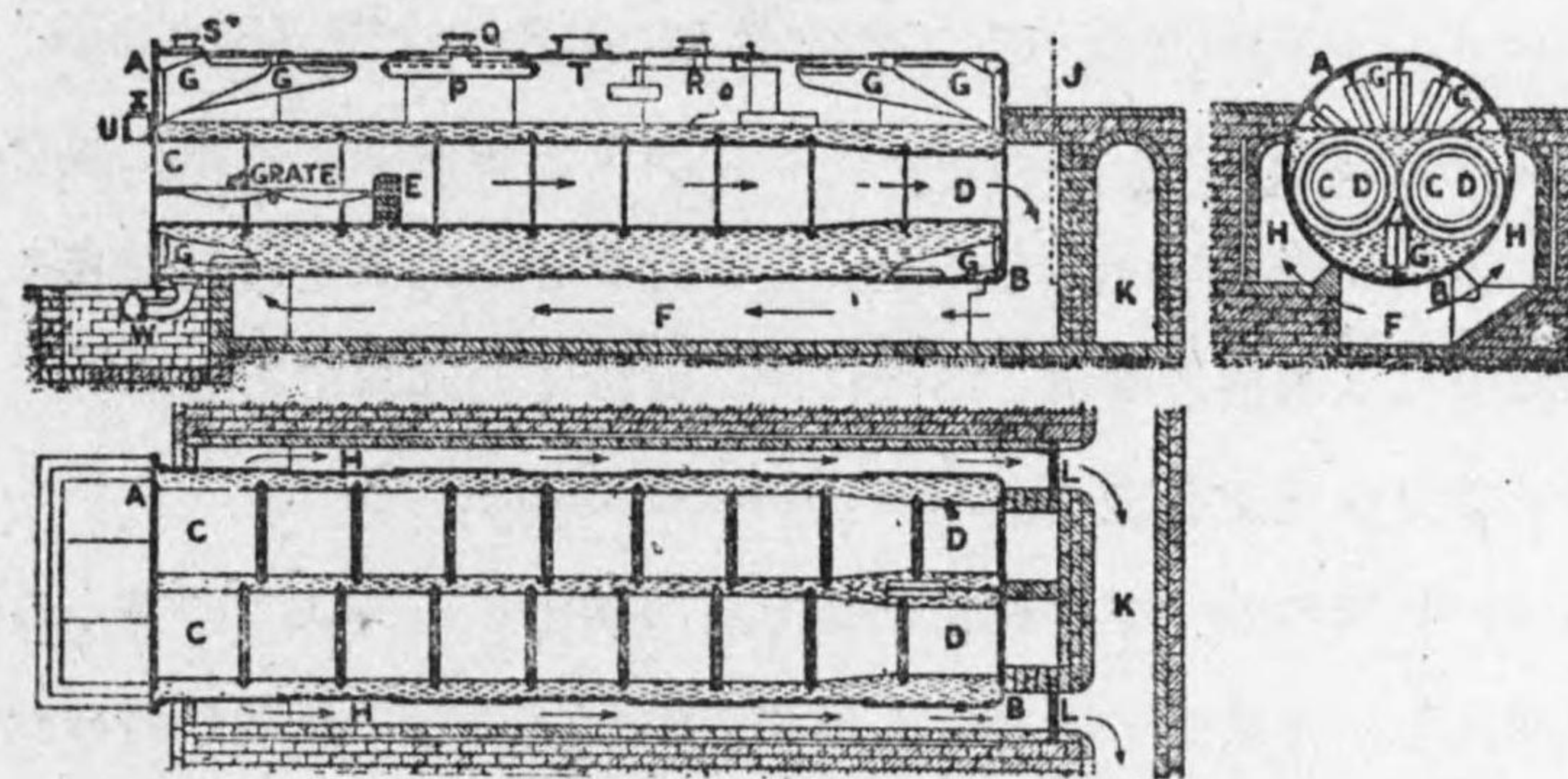
第 5-4 圖 ランカシ罐
