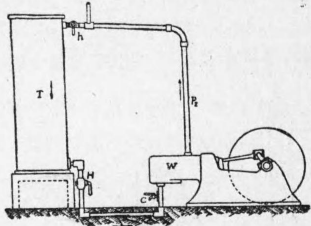
第 8-12 圖 熱サイフォン式冷却装置
