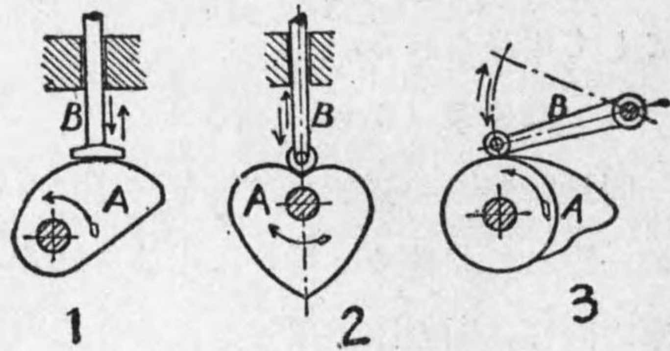
第3—34圖 板カム
