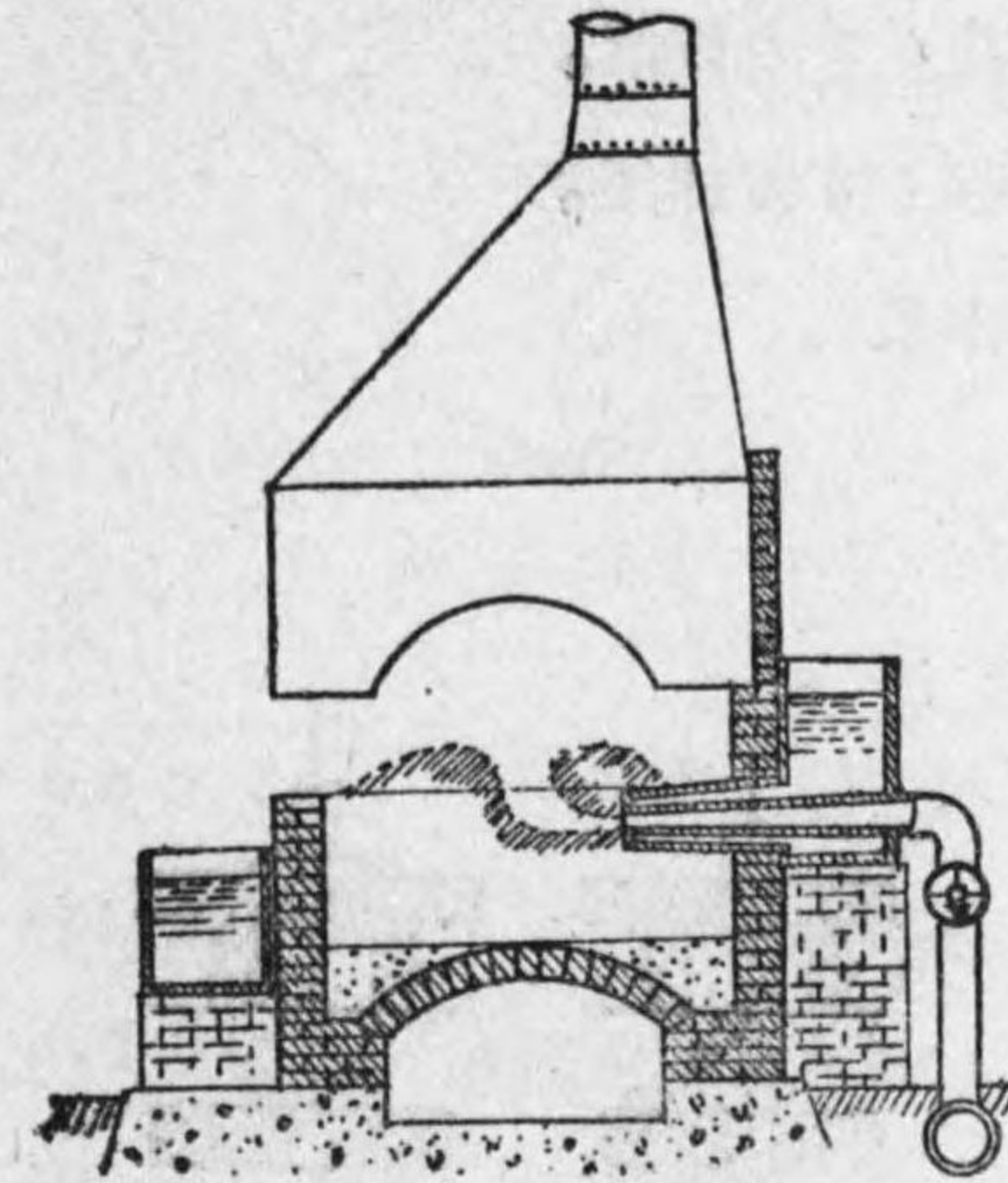
第 10-25 圖 煉瓦積火床
