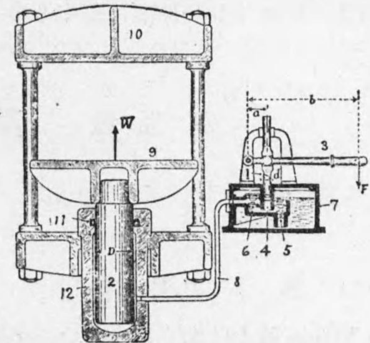
第 4-31 圖 水 壓 機
