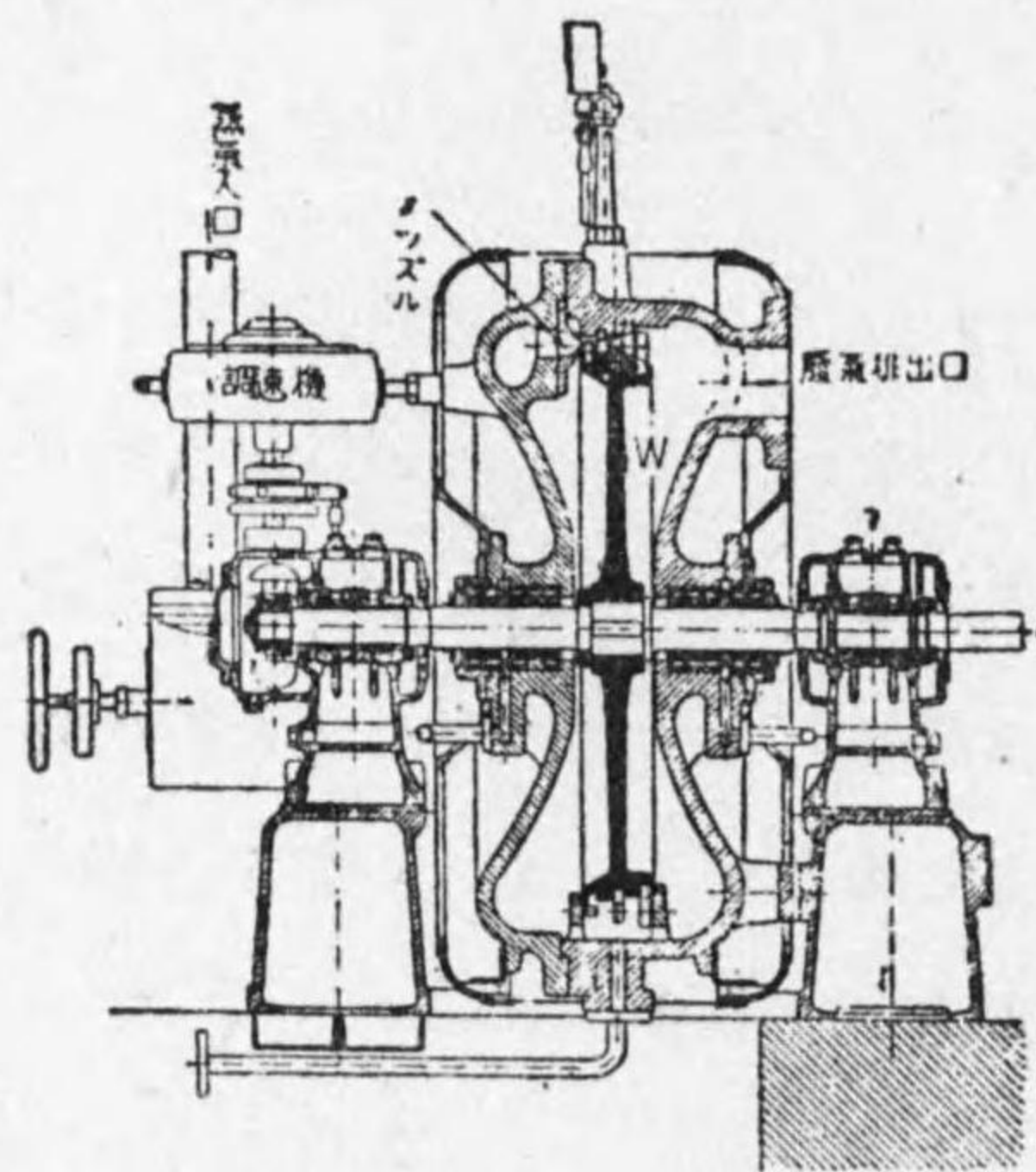
第 6-17 圖 一段カーチス・タービン
