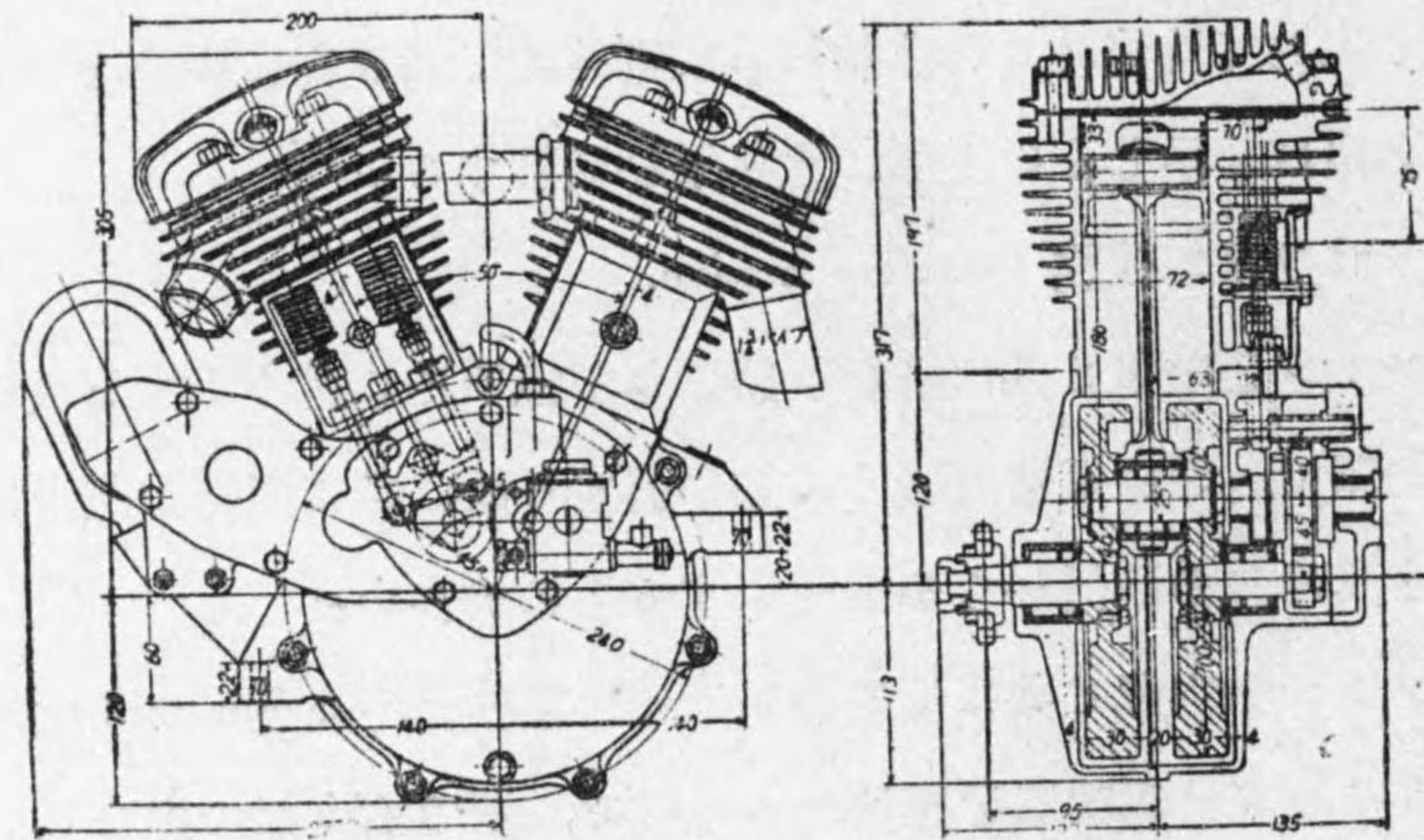
第 8-20 圖 自働自轉車用ガソリン機関
