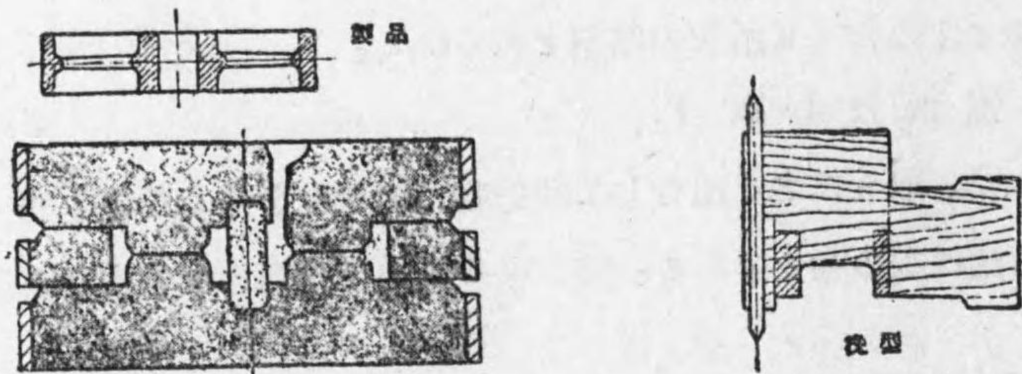
第10—7圖 挽 型
