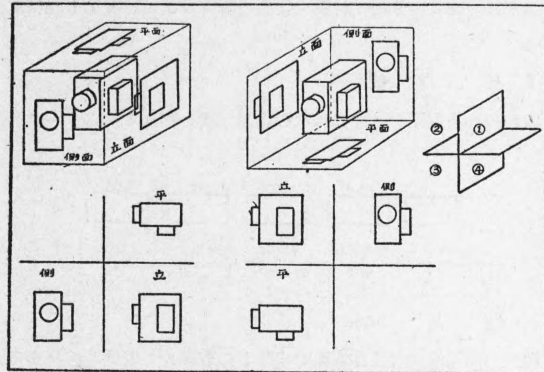
第 3-58 圖 第一角及第三角投影書法
