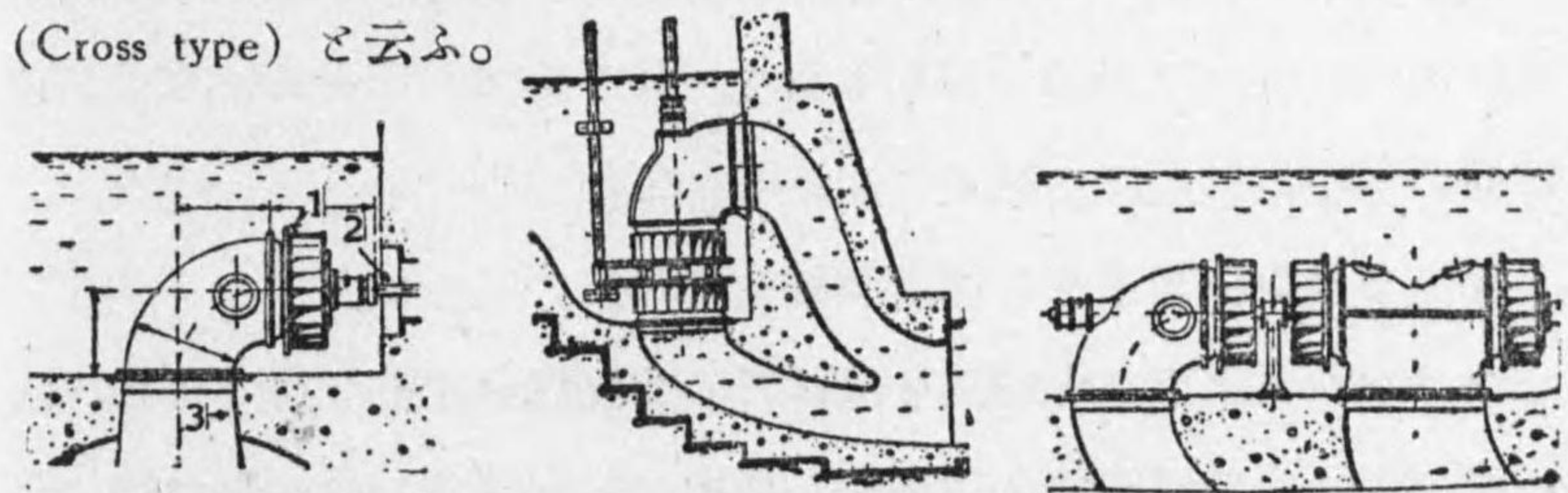
單車横型露出水車
