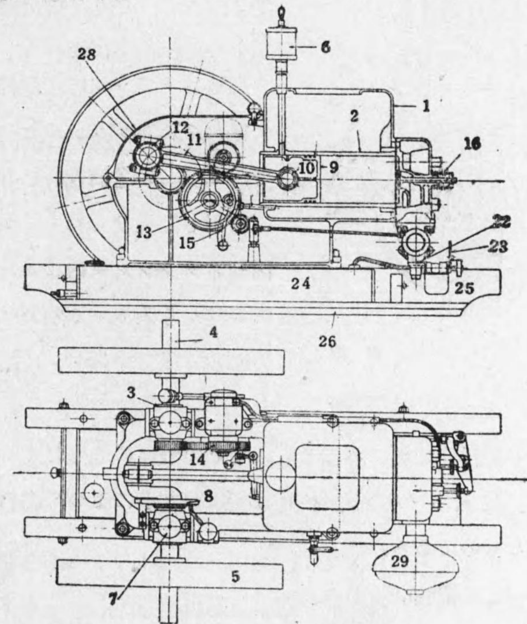
第 8-22 圖 農工用石油機関
