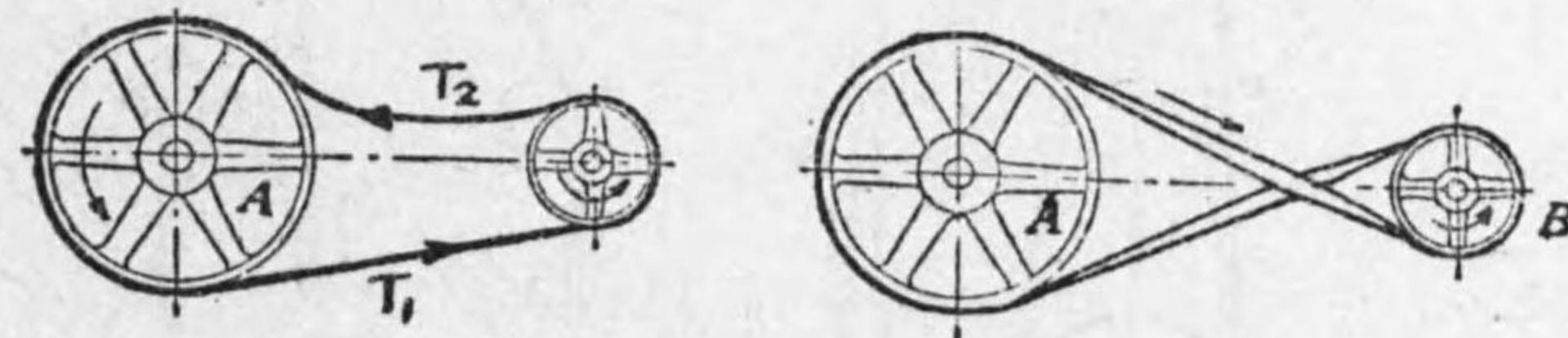
第3—37圖 ベルトの掛方
