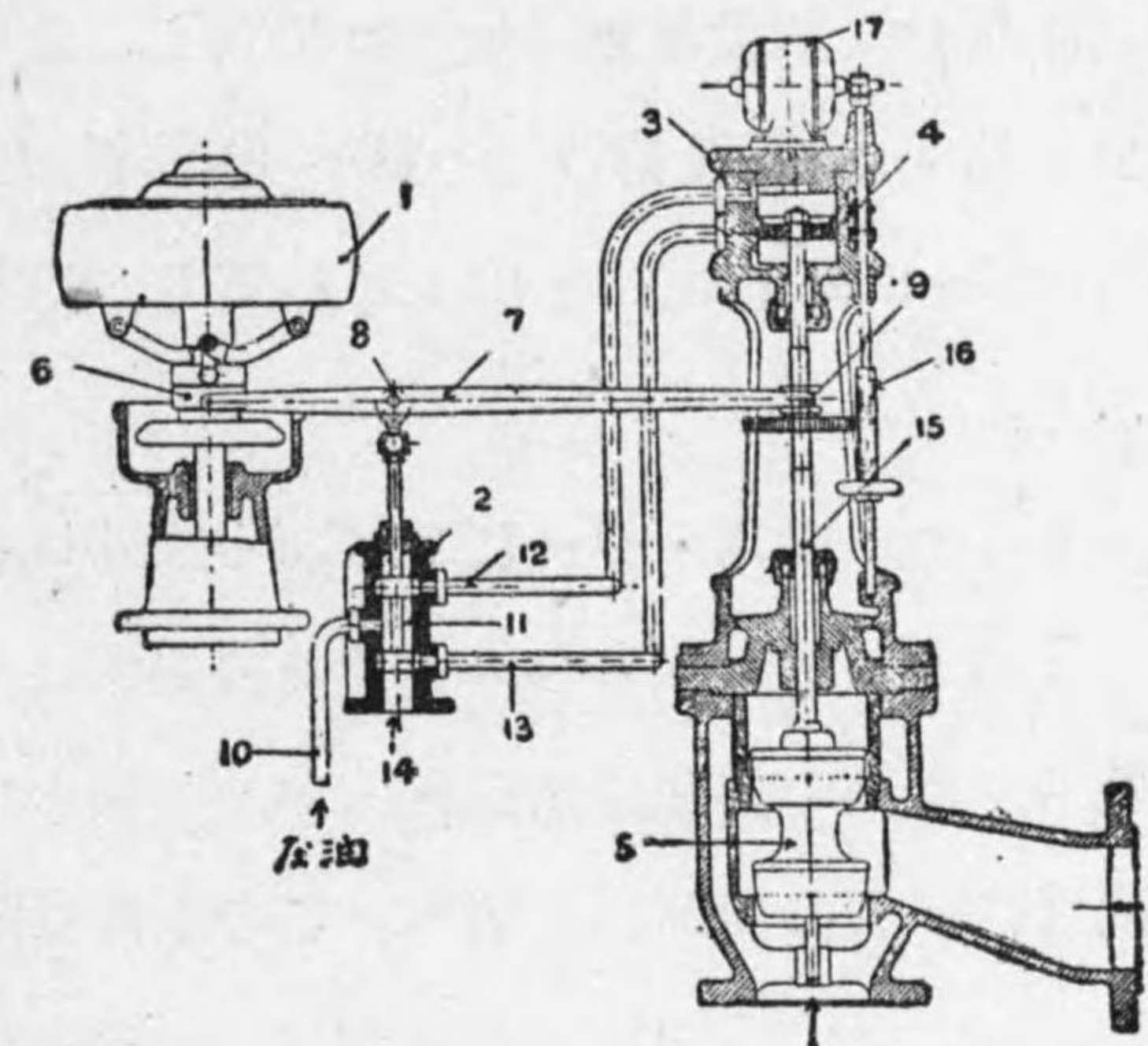
第7-16圖 絞り调速装置
