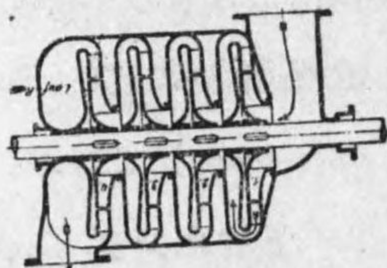
第 4-24 圖 四段タービンポンプ
