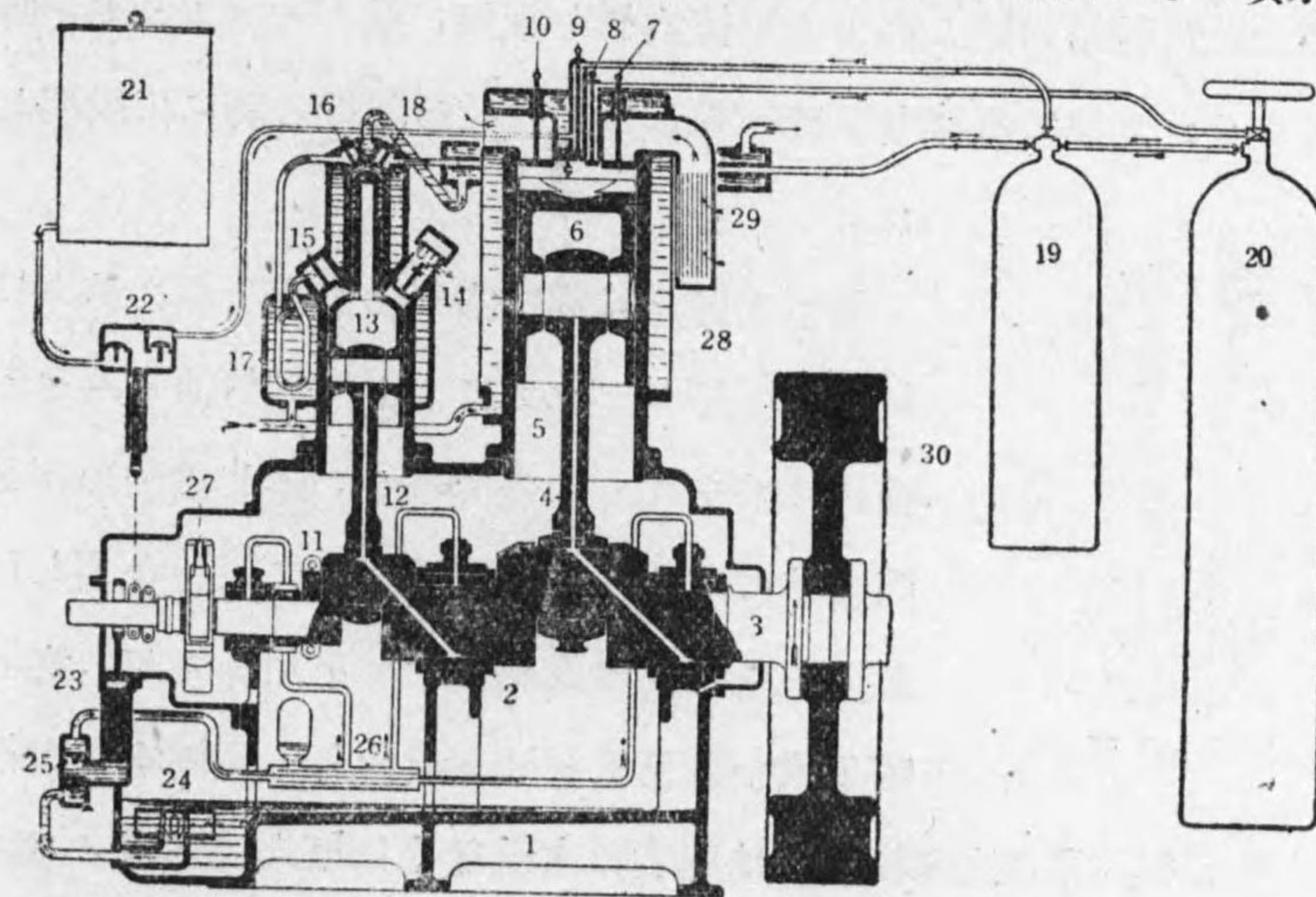
第 8-24 圖 空 氣 噴 射 式 ー ー ー 機 關
