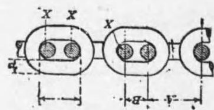
第3-51圖 輪形鎖
