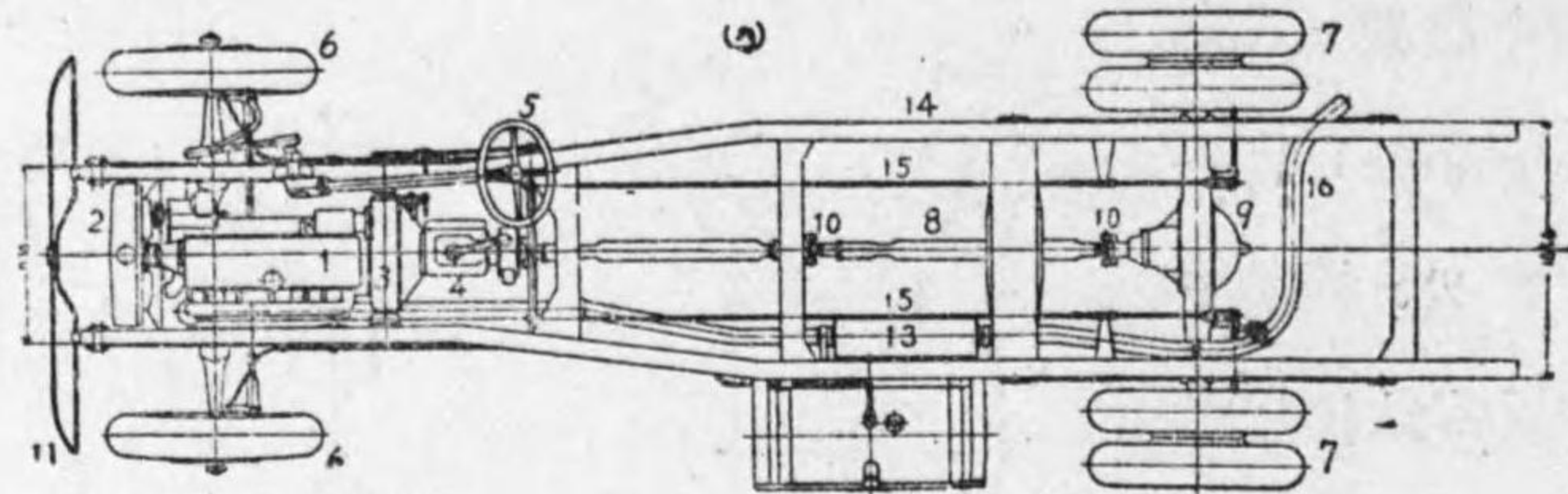
第 8-29 圖 乗合自動車々臺
