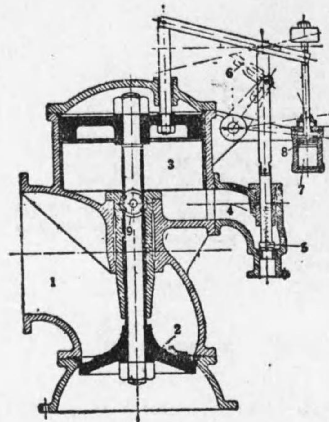
第 4-19 圖 水圧式水圧調整機
