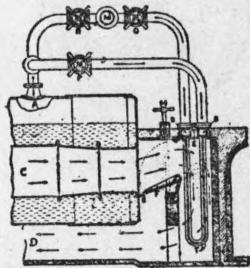
第5-24圖 ランカシ罐の過熱器
