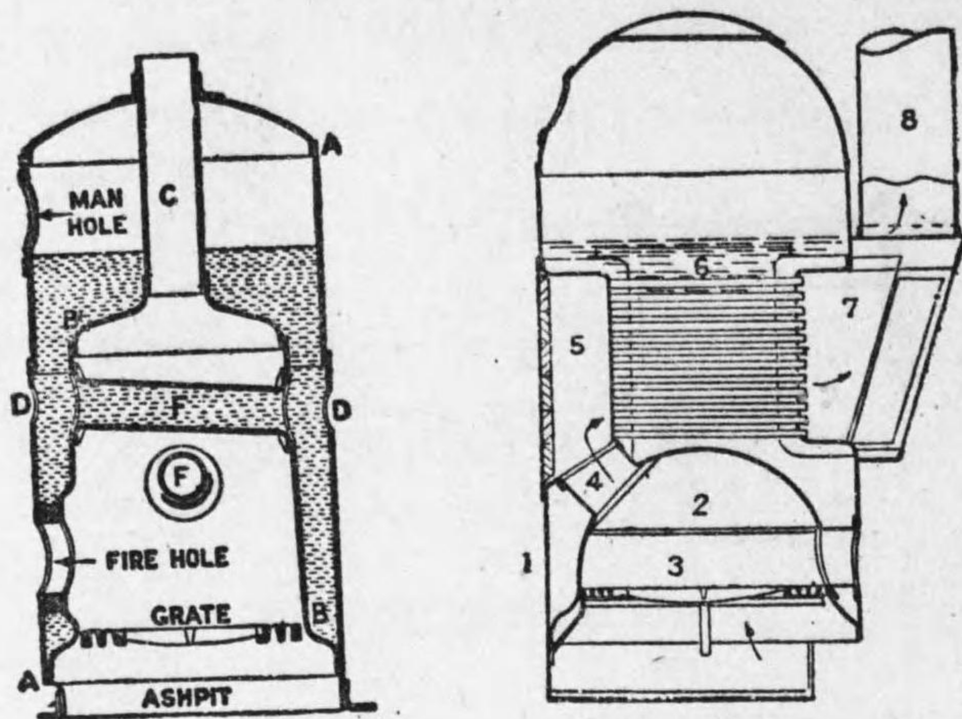
第 5-6 圖 コックラン鍋
