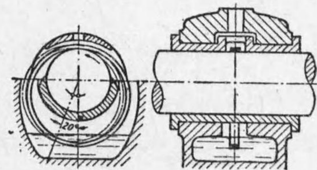
第3-15圖 給油輪軸承
