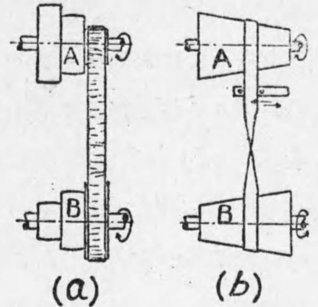
第 3-42 圖 段車と圓錐調車
