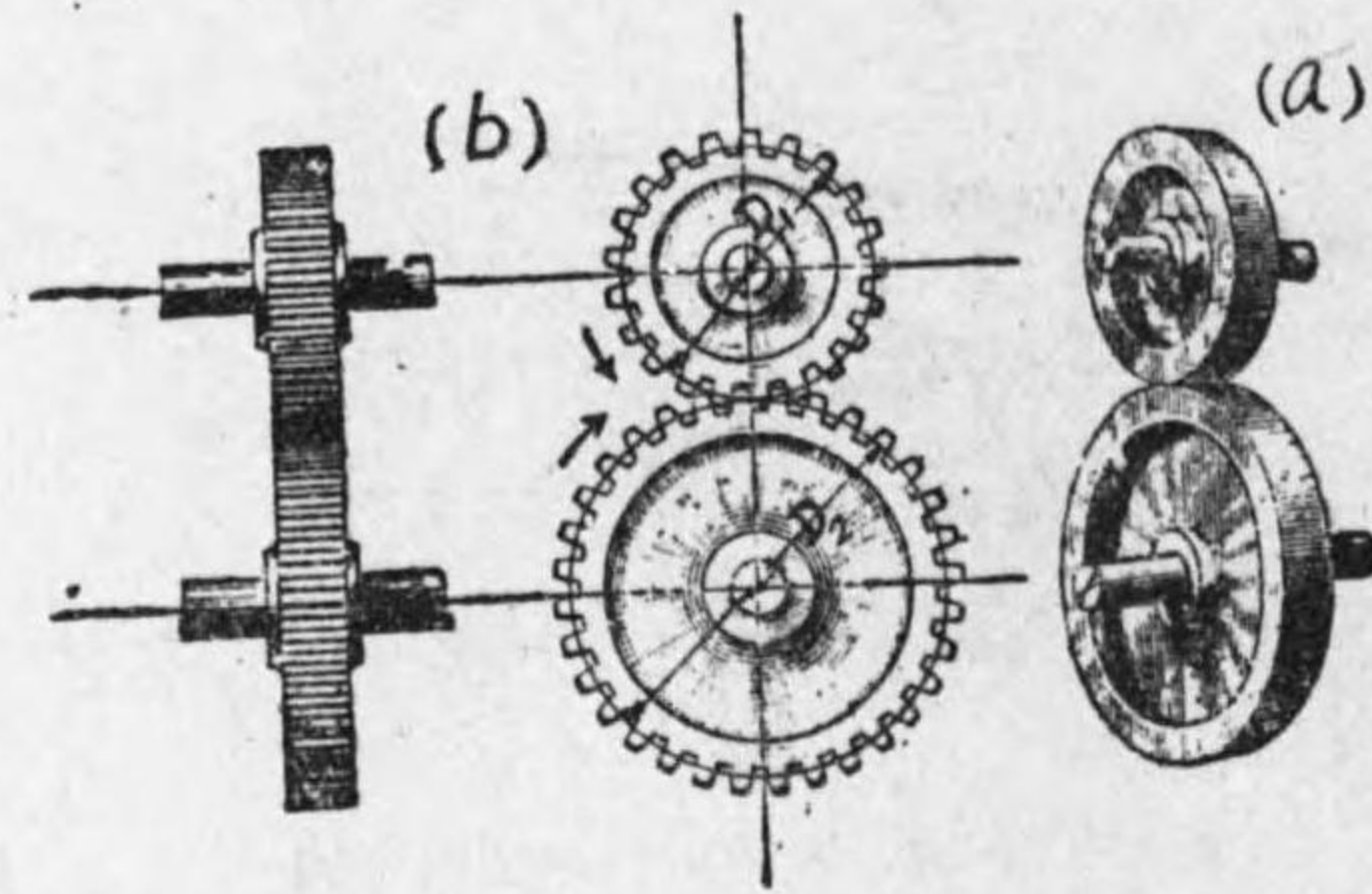
第 3—24 圖 正齒車
