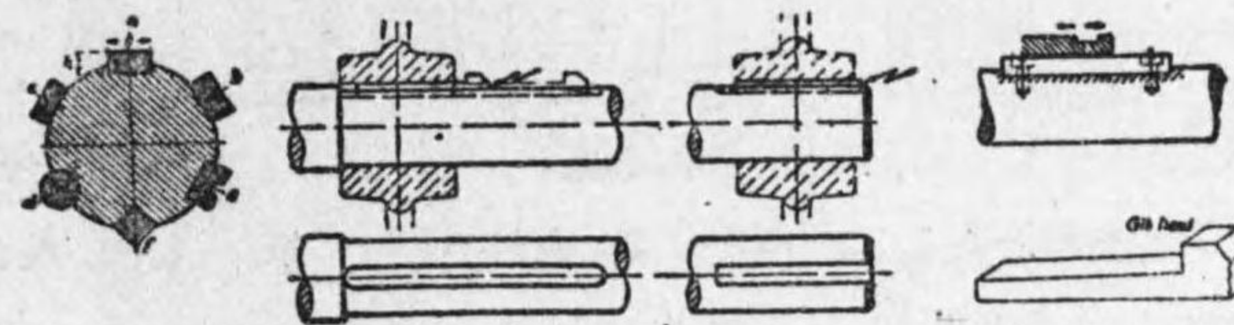
第 3-4 圖 キー
