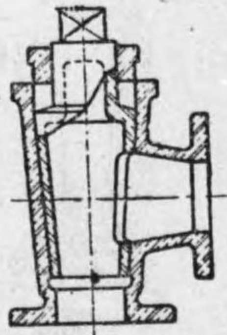
第 3-18 圖 肘コック
