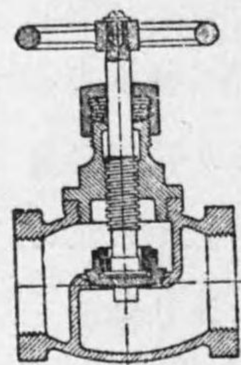
第 3-17 圖 球型弁
