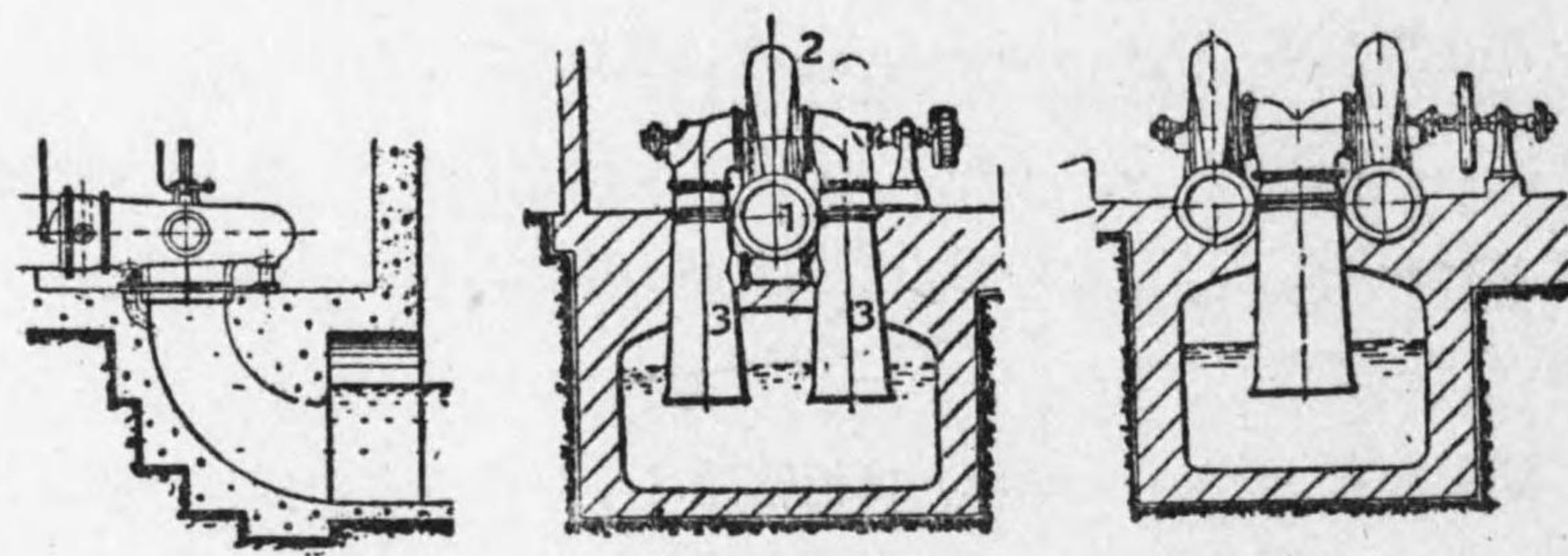
複車横型渦卷水車
