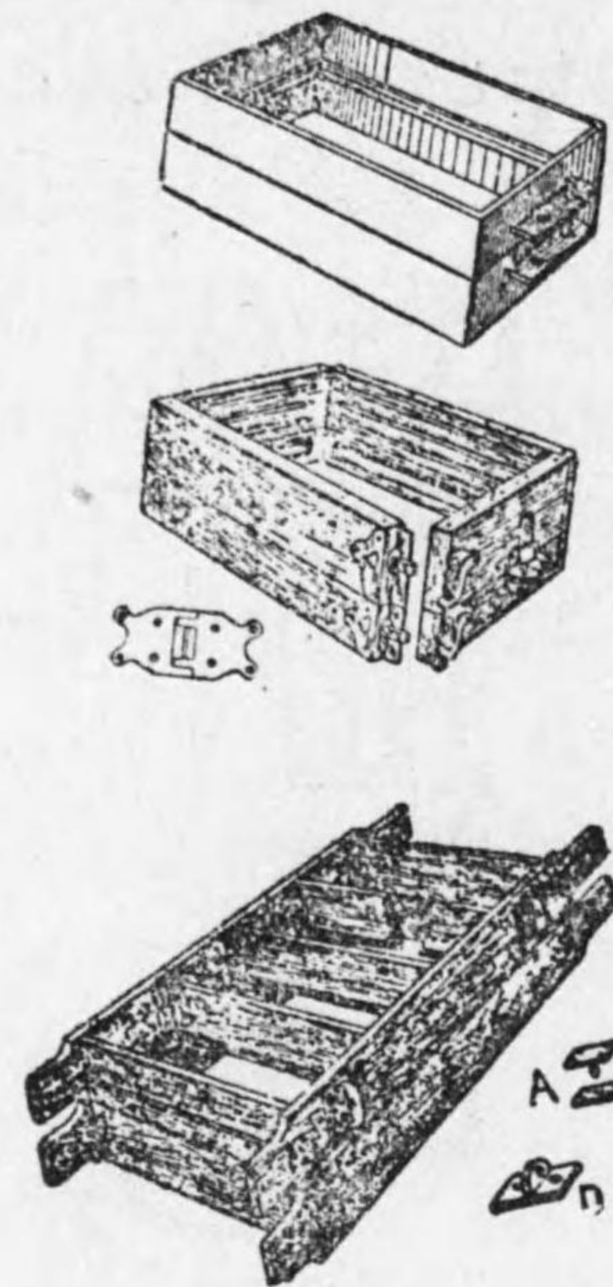
第 10-14 圖 鑄 型 枠
