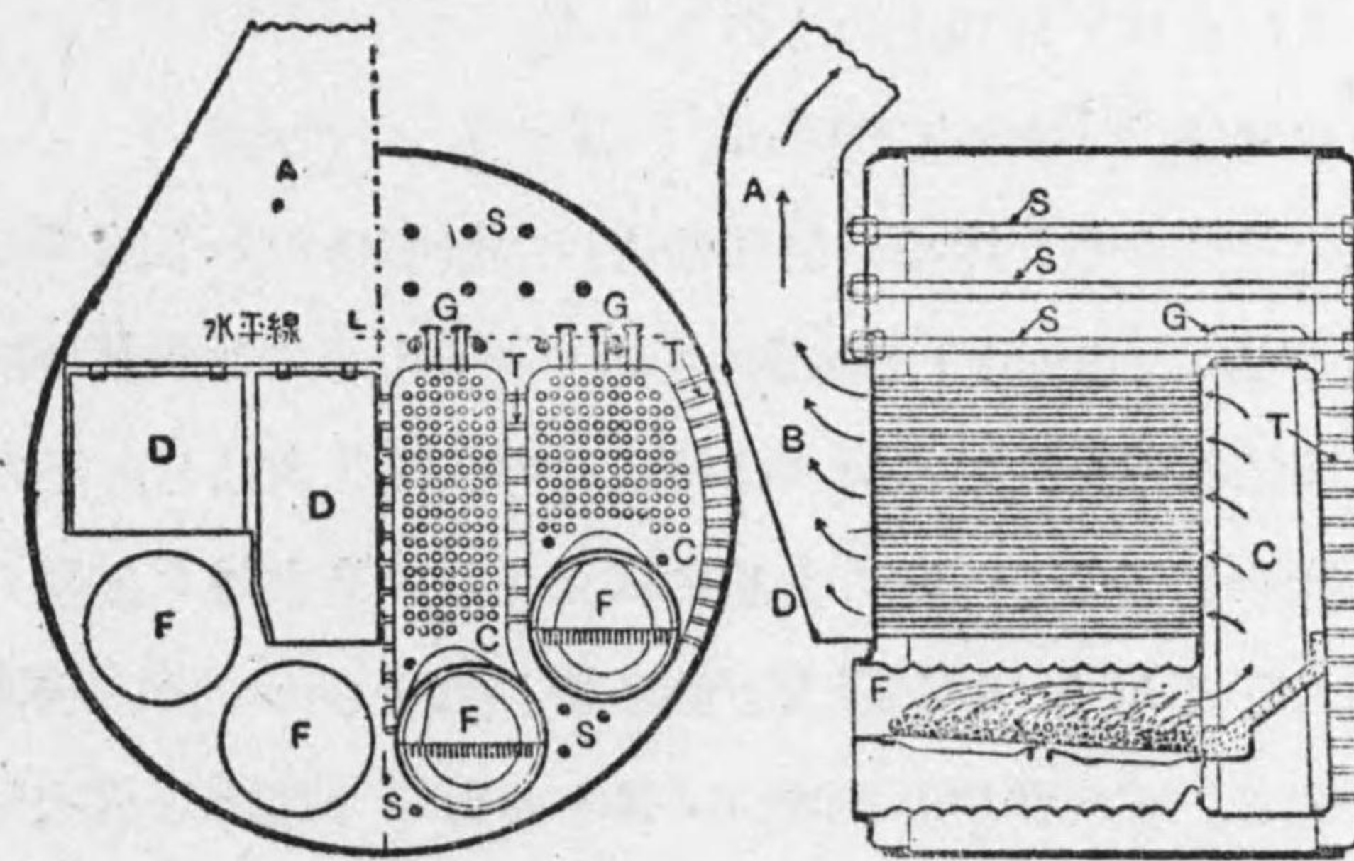
第 5-8 圖 スコッチ船用鍋
