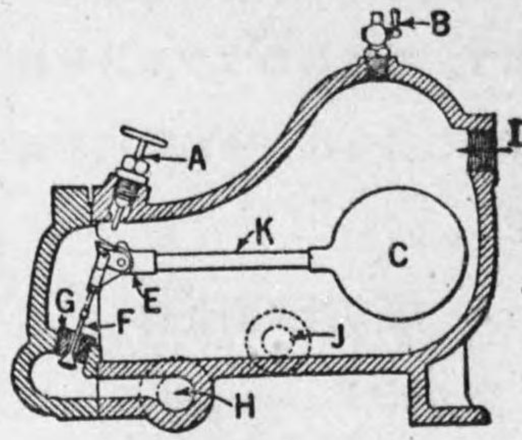
第5-23圖 スチームトラップ
