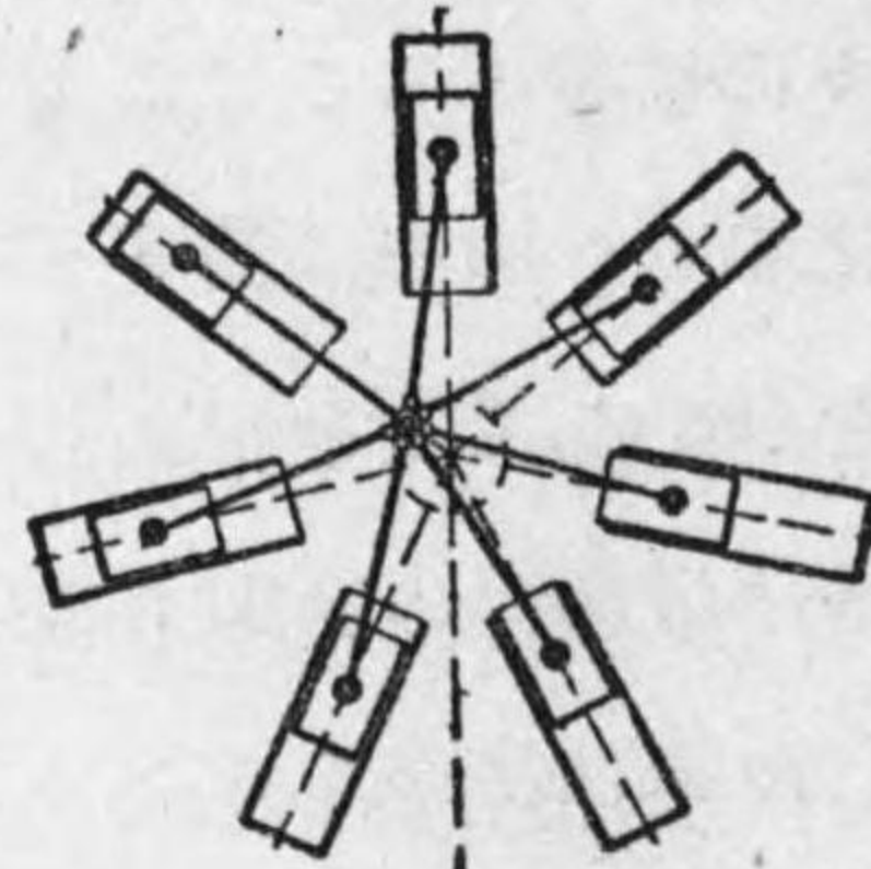
第 8—34 圖 星型機關
