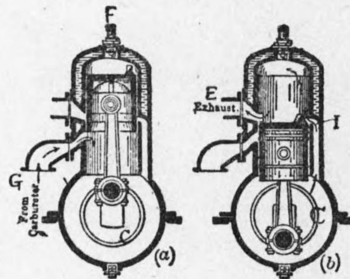
第 8-2 圖 ニサイクル機關
