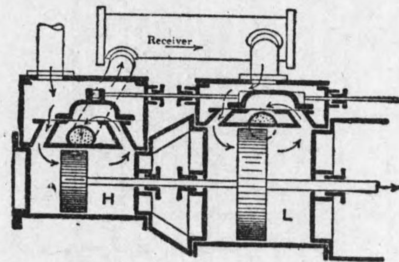
第 6—12 圖 串型機関
