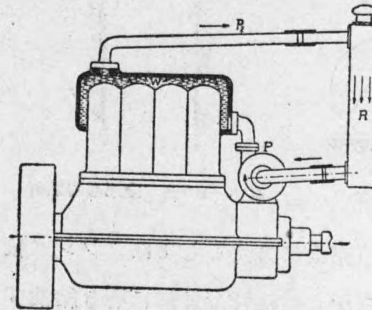
第 8-10 圖 自動車機關の強制循環冷却装置
