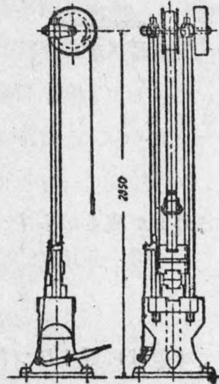
第 10-27 圖 落 錘
