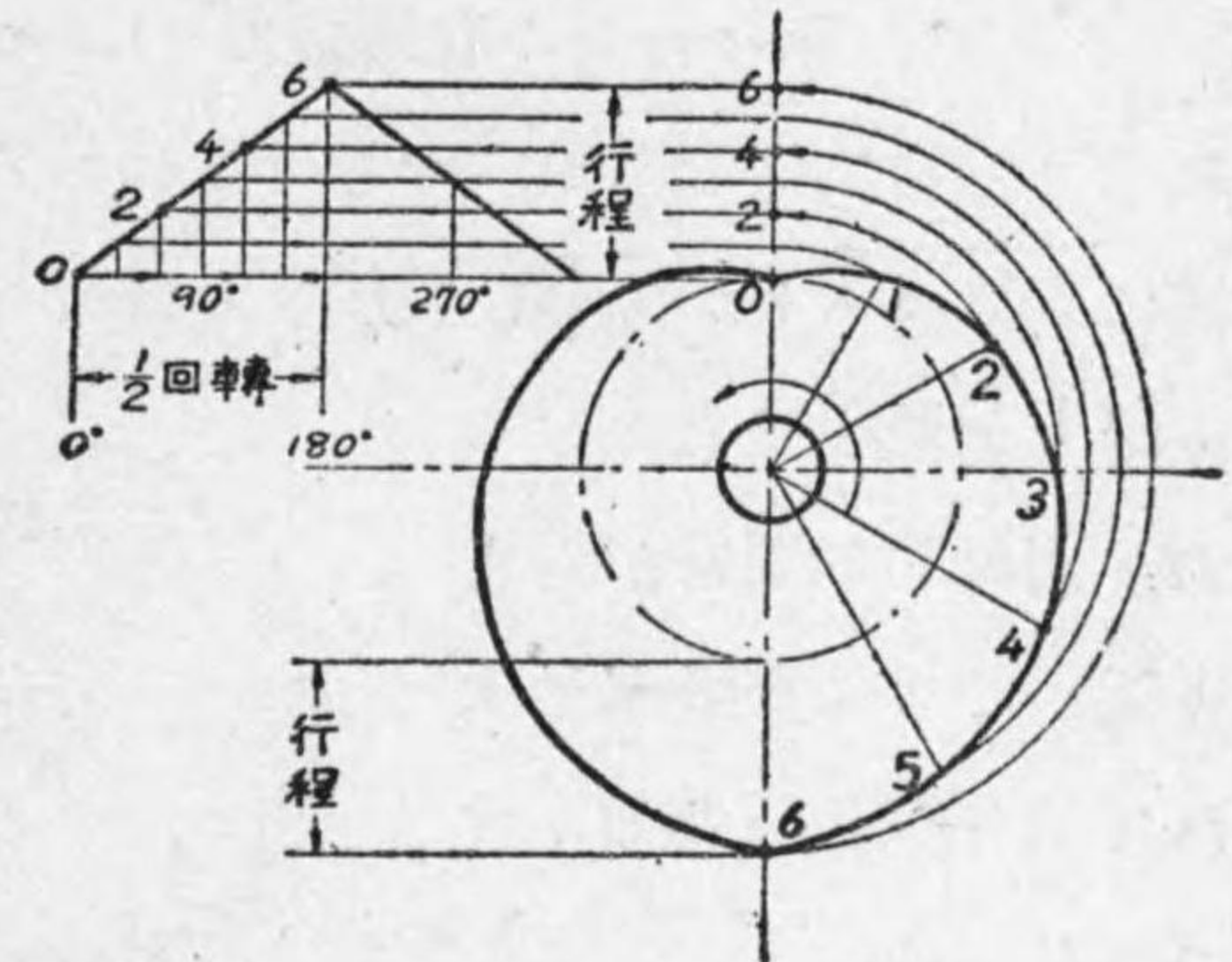
第3—36圖 ハートカムの畫法
