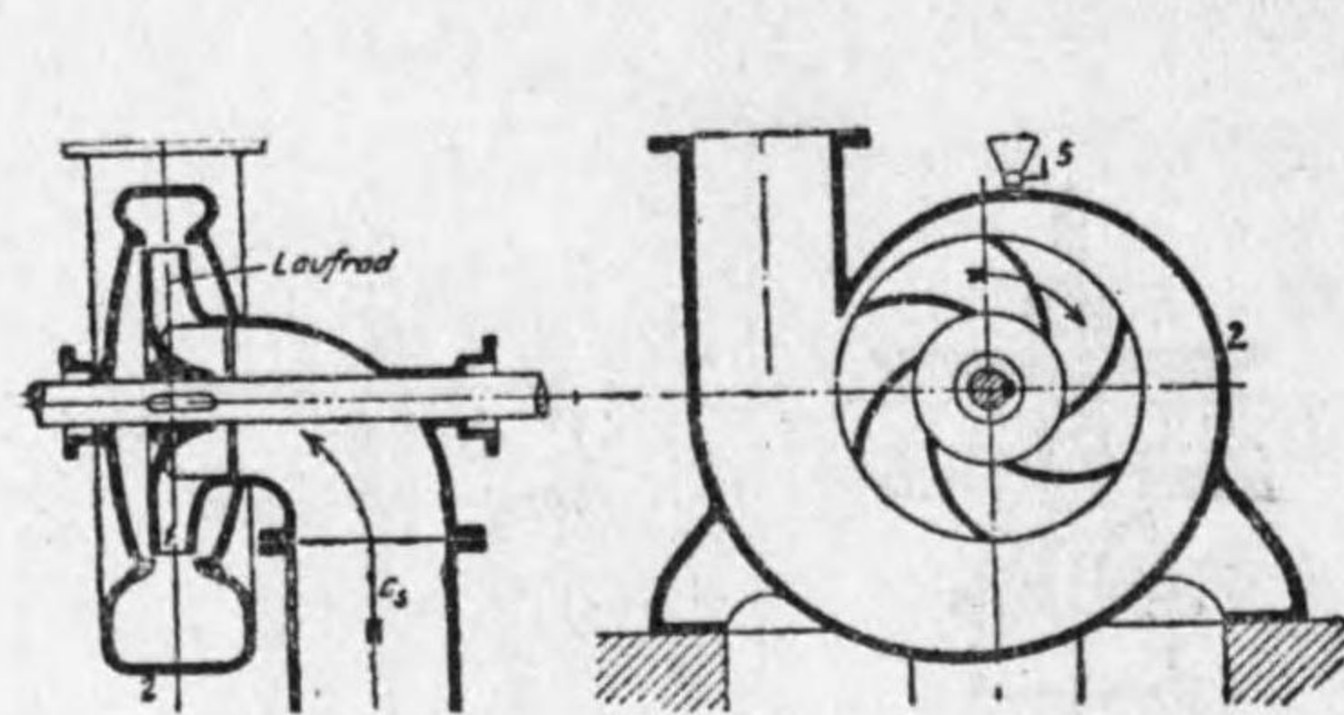
第 4-21 圖 片側吸込渦巻ポンプ
