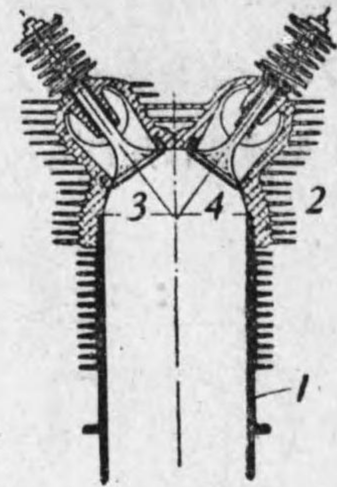
第 8-13 圖 空気冷却気筒
