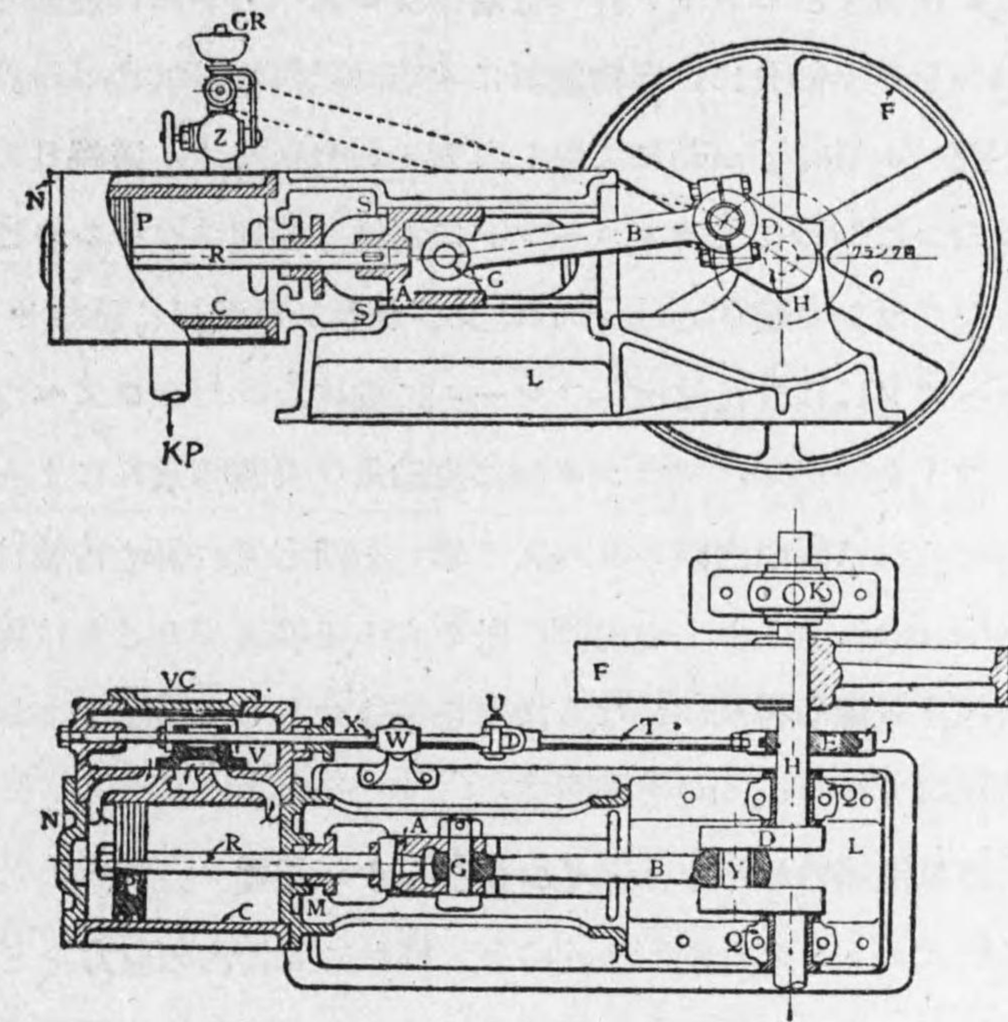
第 6-1 圖 蒸氣機關
