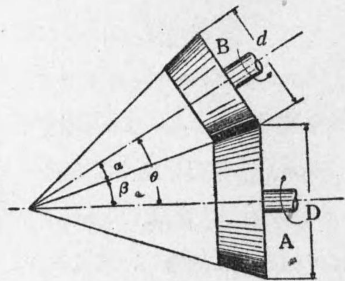
第 3-20 圖 外接圓錐摩擦車
