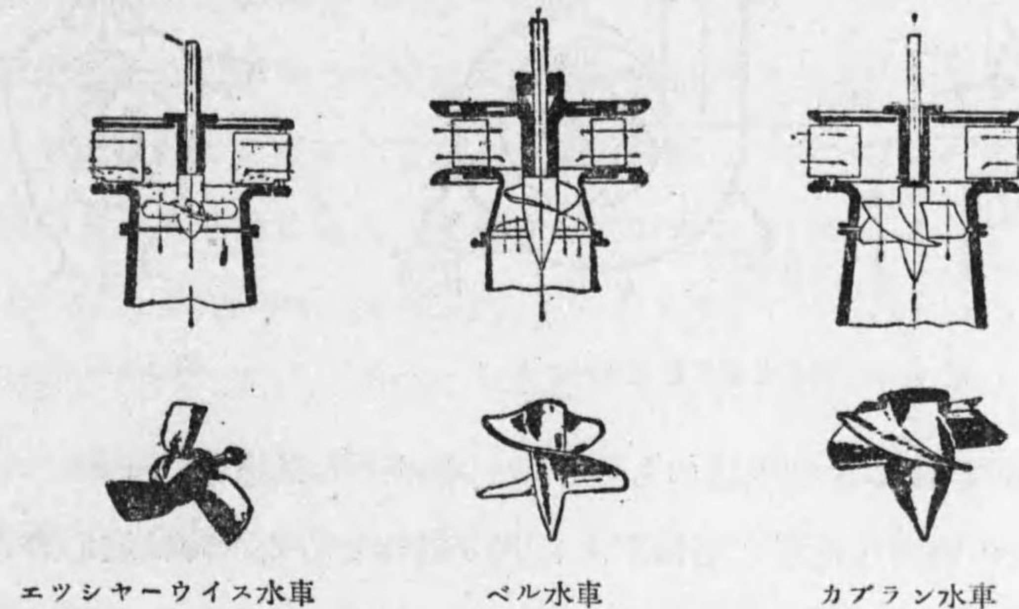
第 4-20 圖 プロペラー水車
