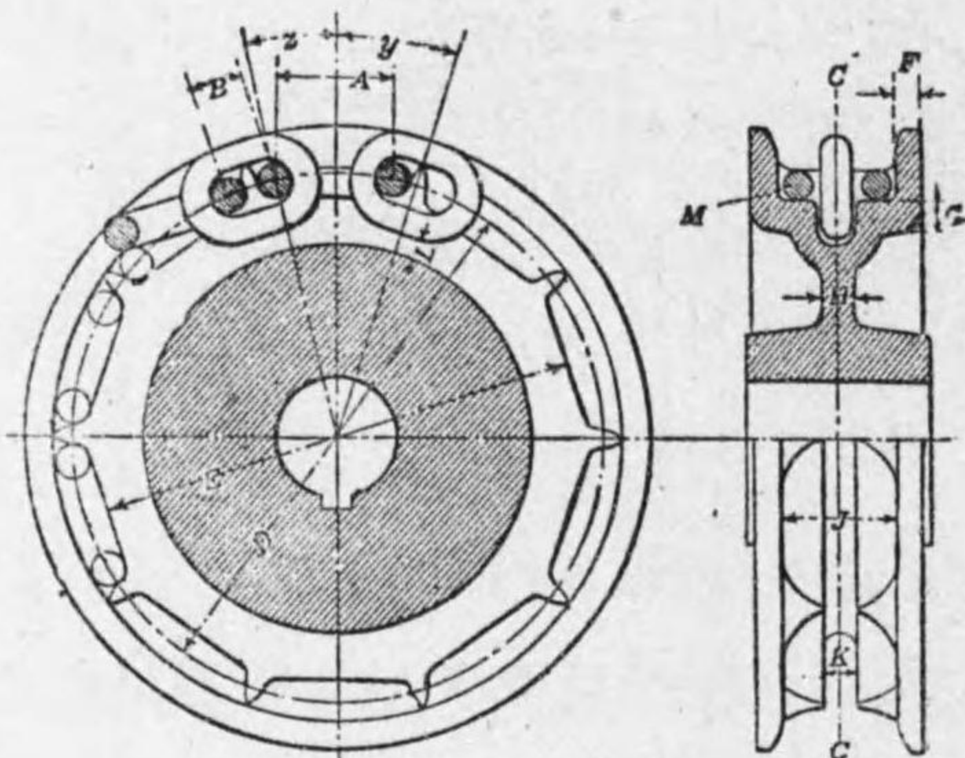
第3-52圖 荷揚用鎖車
