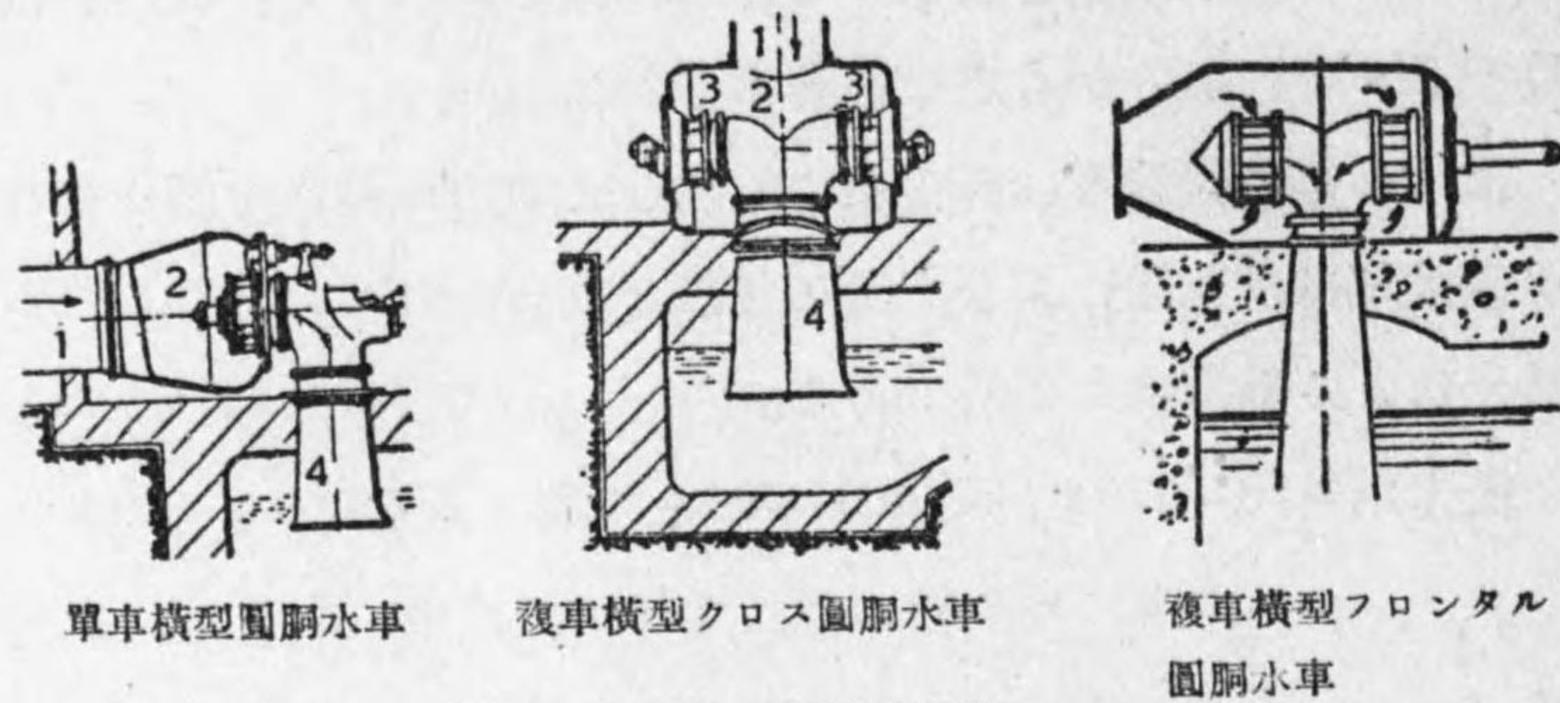
第 4~16 圖 圓筒型水車
