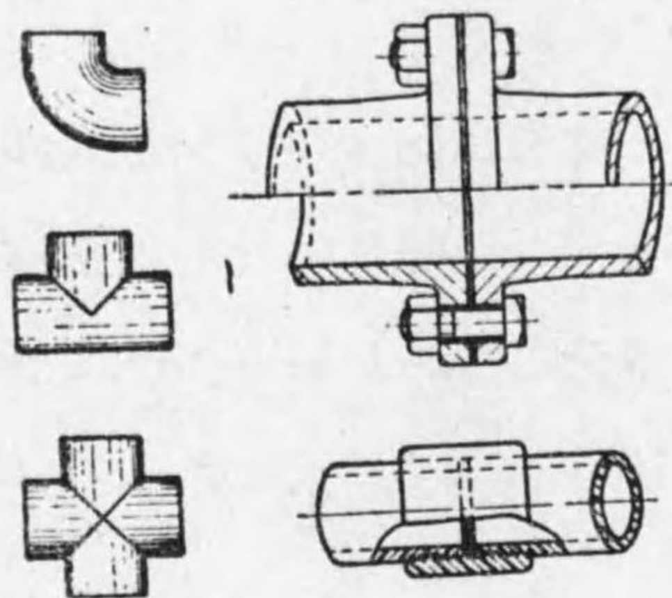
第 3-16 圖 管接手
