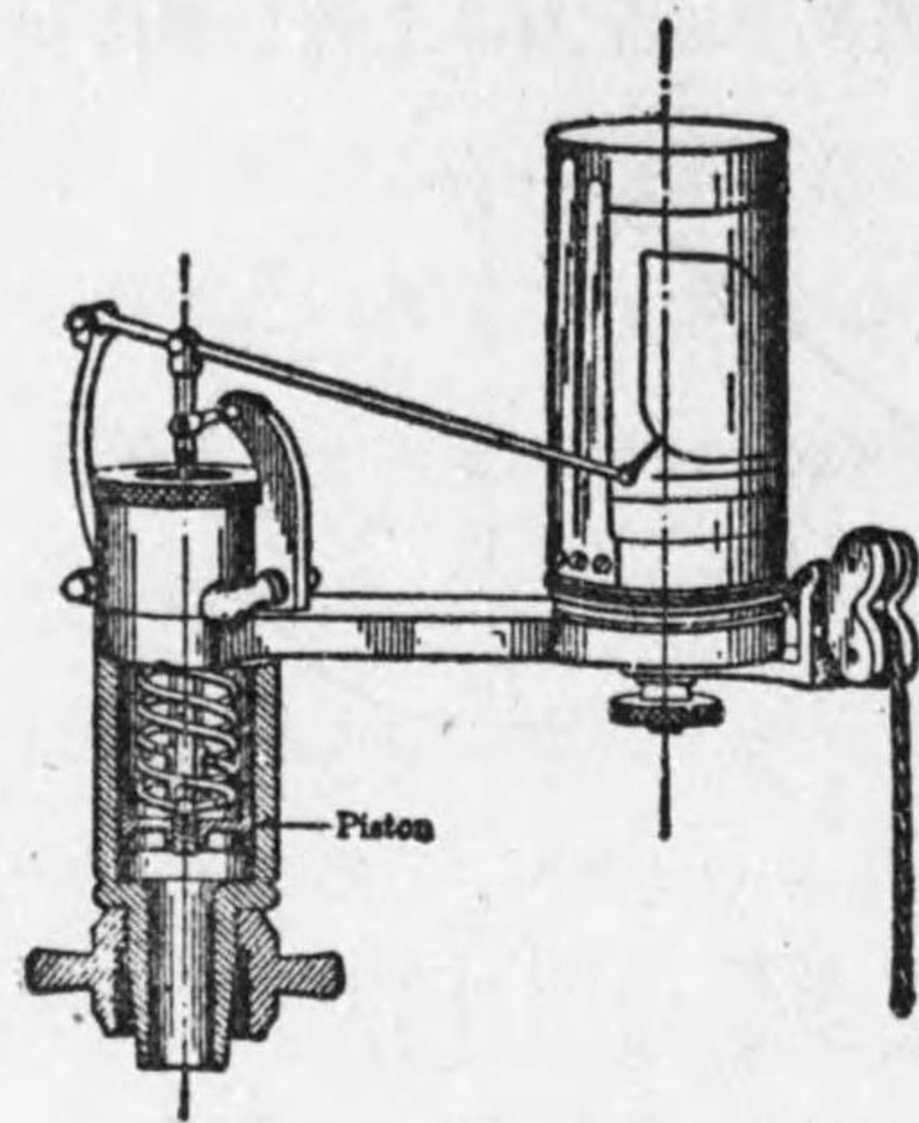
第 6-3 圖 インヂケータ-
