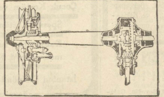
Arka dingil-azami mukavemet
