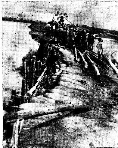
→作者在三元塔下視察搶險工程
