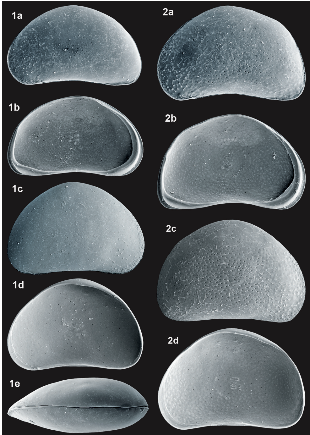
Potamocypris altenburgensis FUHRMANN, 2010 – Altenburg Rezentprobe 1046 1a - LVa (L 0,57), 1b - LVi (L 0,57), 1c - RVa (L 0,56), 1d - RVi (L 0,57), 1e - Cpd (L 0,60). Potamocypris arcuata (SARS, 1903) – Leipzig Rezentprobe 135 Weibchen: 2a - LVa (L 0,66), 2b - LVi (L 0,66), 2c - RVa (L 0,64), 2d - RVi (L 0,67).
