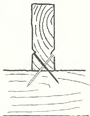
Toenailing
