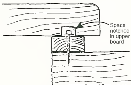
Dap
