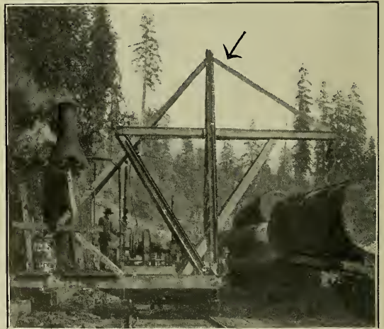
Fig. 6. Unloading Apparatus.
