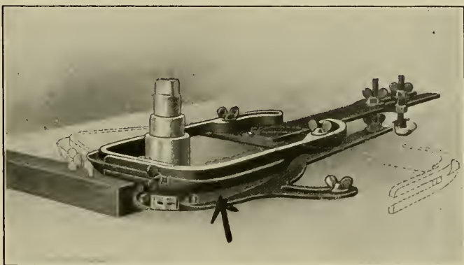
Fig. 178. K. C. Shaper Guard.
