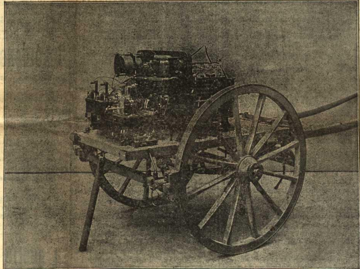
Estación militar transportable. Carro de los aparatos
