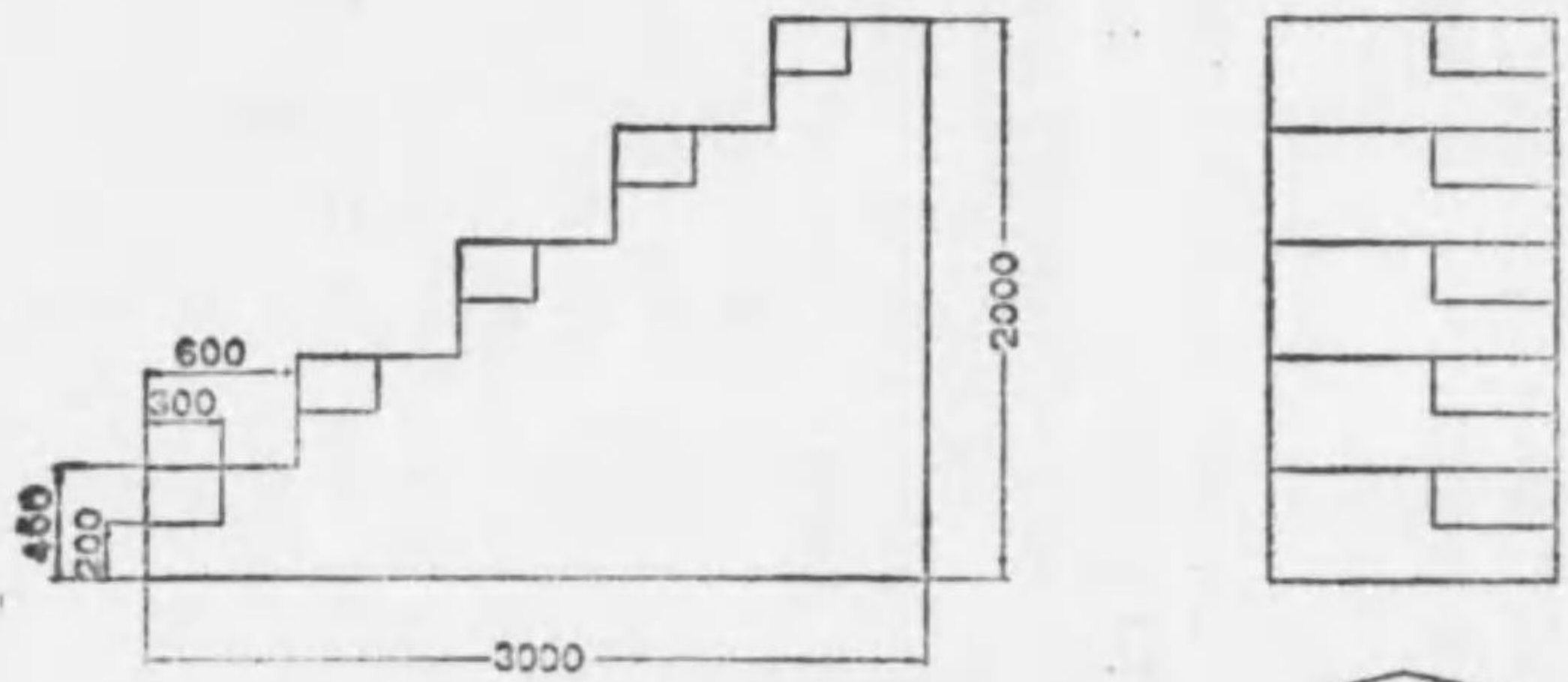
決勝審判臺ノ圖解
