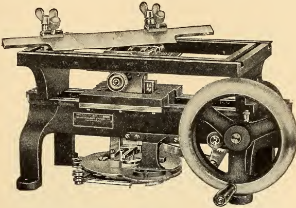
FIG. 118.—Minot precision microtome (Bausch & Lomb).
