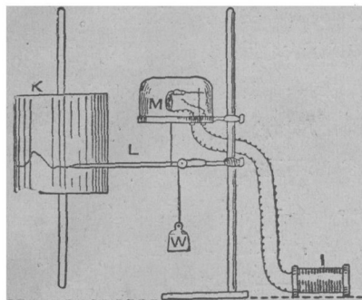
第二七圖 肌肉收縮的自記裝置
