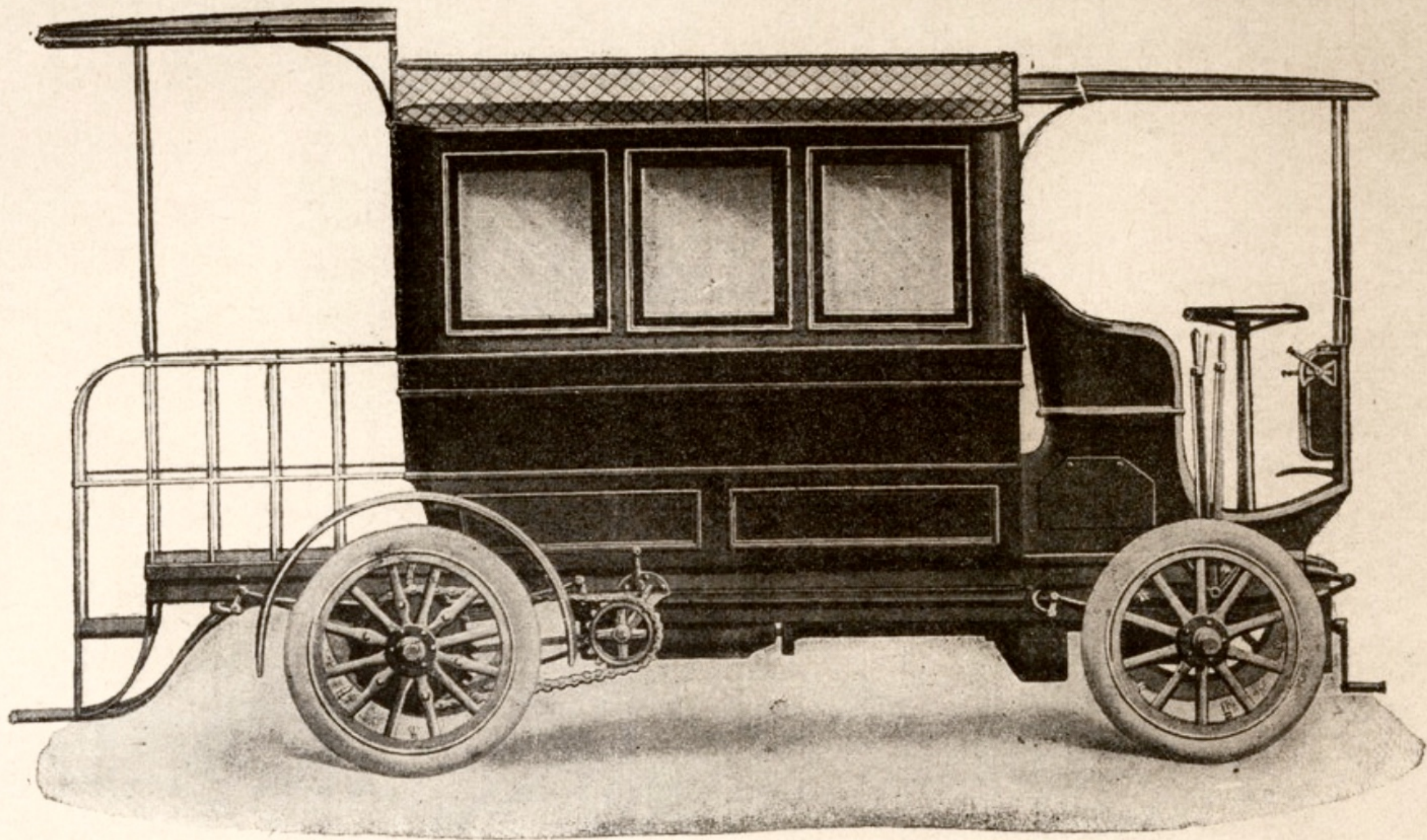
FIG. 2. — Petit omnibus pour service public avec plate-forme arrière (Ariès).
