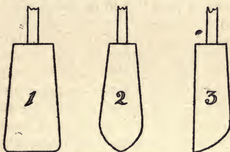
PISÉ HAND RAMMERS
