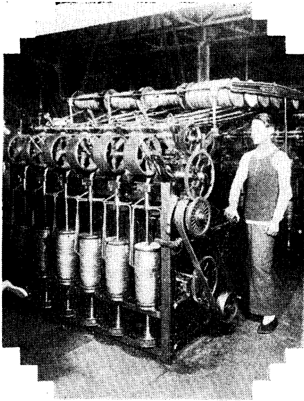
● 二道煉 條機 ● 併數毛條 為一條使 之成爲更 進一步之 相當重量 與細度
