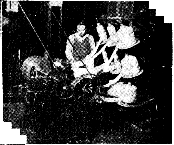
●纏球機● 將四根毛條 打成一球以 備梳毛機用
