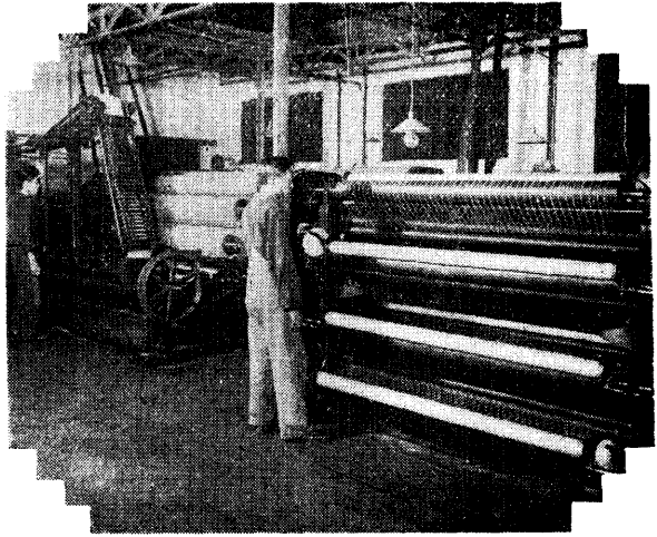
●粗梳鋼絲機●
