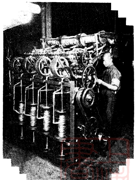
● 頭道煉 條機 ● 併數毛條 爲一條並 使至相當 之重量與 細度
