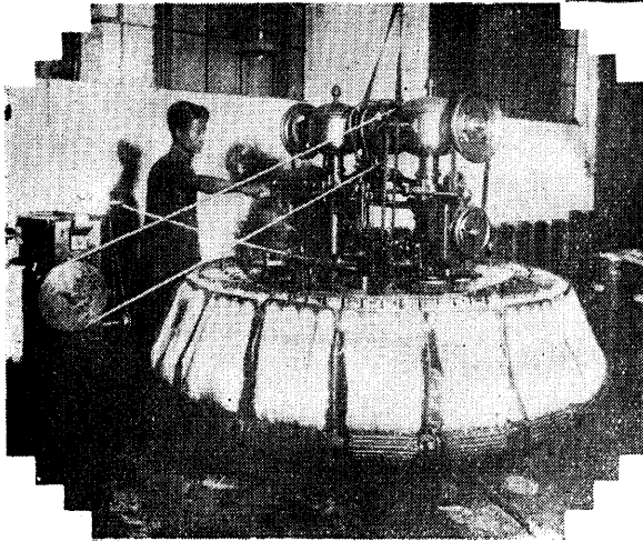
●諾布梳毛機● 此乃第三次重梳於 梳毛之外將長纖維 盡量收留使色光澤
