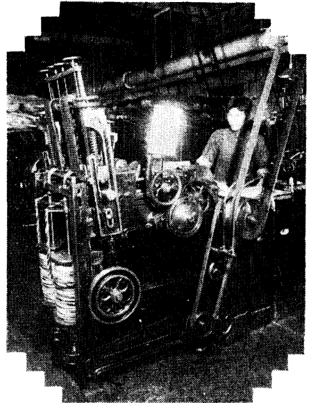
● 雙錠 機 ● 此爲第七 次（卽末 次）重梳 並爲第一 次機器加 撚度於毛 條
