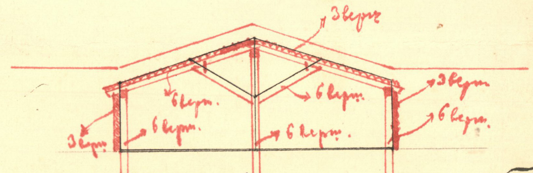
Разрѣзъ погреба въ ширину: отъ а. до б.
