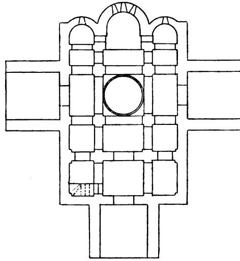
48. Лехне. Планъ церкви.
