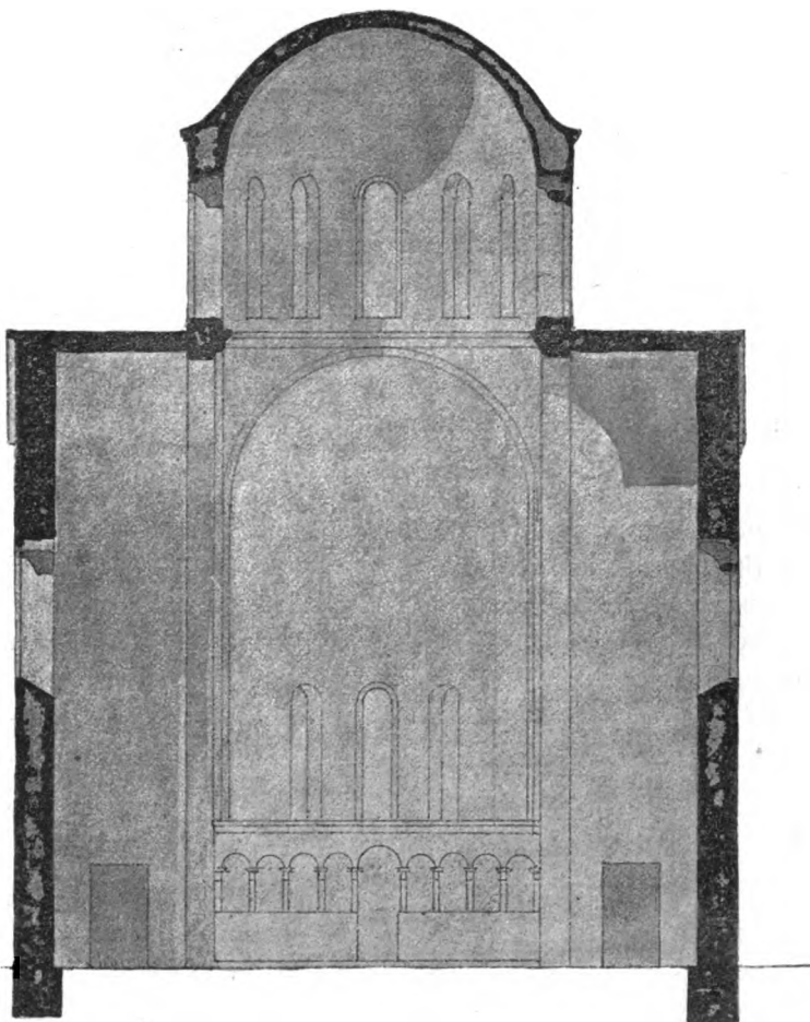
52. Пицунда. Разрѣзъ къ алтарной сторонѣ.
