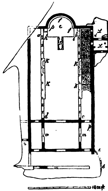
10. Планъ береговой базилики.
