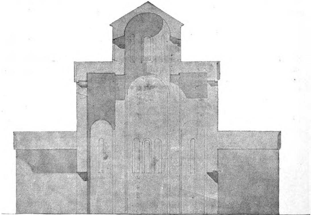
47. Лехне. Поперечный разрѣзъ.
