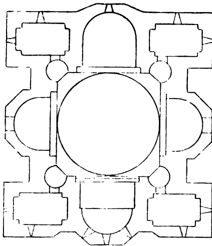
36. Атени. Планъ церкви.
