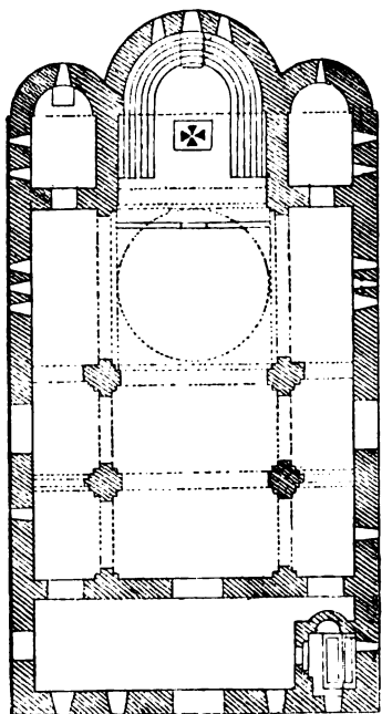
50. Планъ храма въ Пицундѣ.
