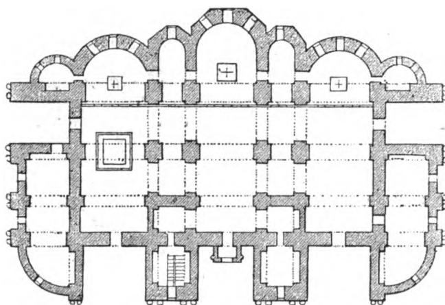
147. Планъ Михайловскаго собора.
