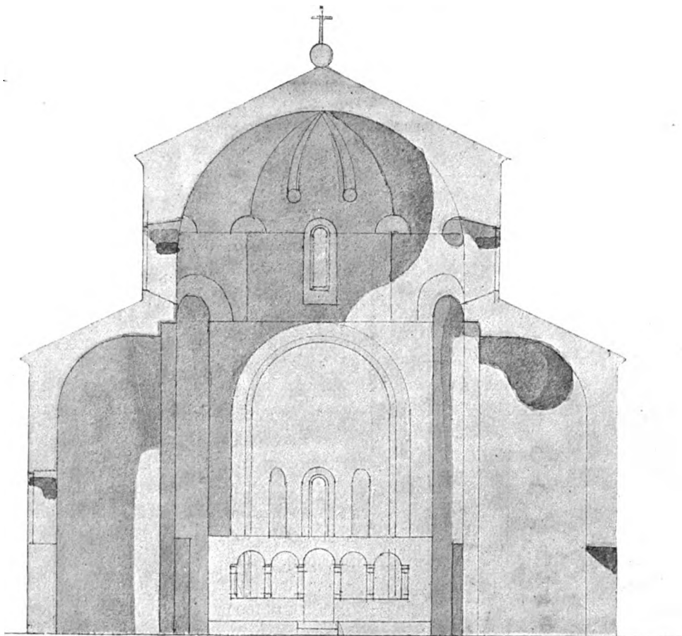
35. Атени. Поперечный разрѣзъ.
