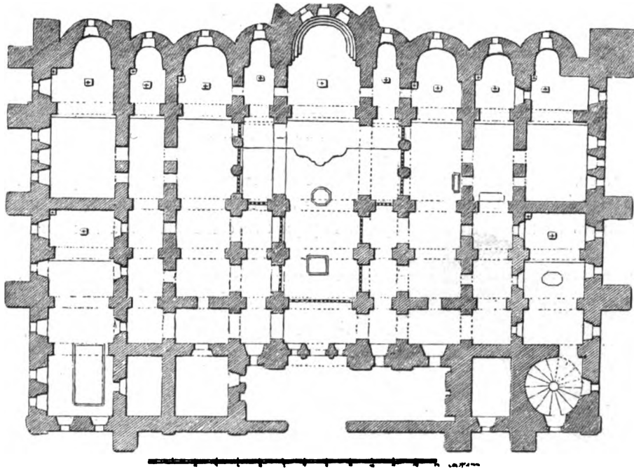
86. Планъ Софійскаго собора въ теперешнемъ его видѣ.
