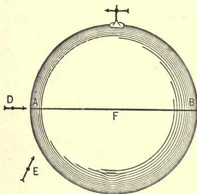
FIG. 5. GILBERT'S TERRELLA.
