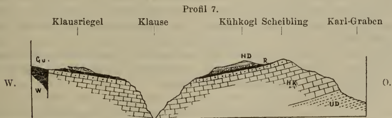
Profil der Klaus bei Krampen.
