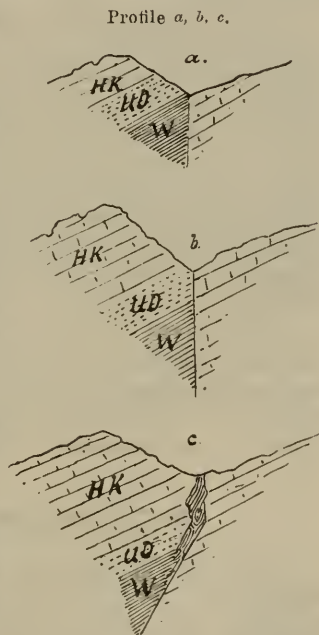
Schnitt a (durch den Sattel) einen der Sattelgräben) so
