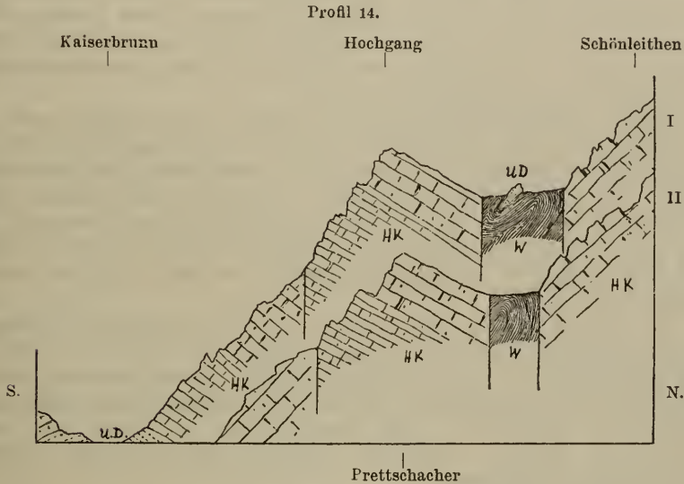
I. Profil durch Kaiserbrunn und den Hochgang. II. Profil durch den Prettschacher.
