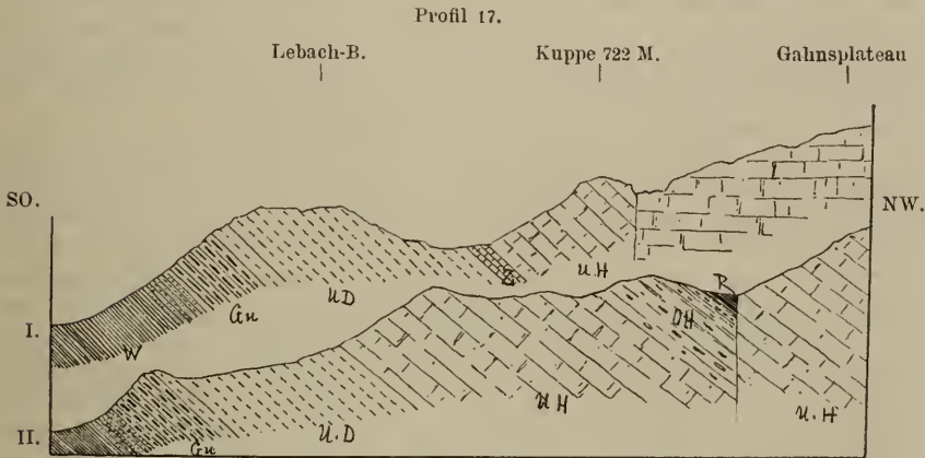
I. Profil durch den Lebach-Berg und das östliche Gahnspaneau. II. Profil durch den Rücken westlich von Sieding (Schafkogel).
