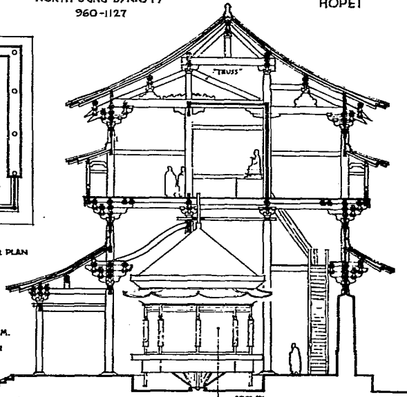
橫斷面 CROSS SECTION
